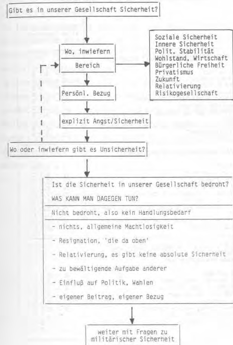
Übersicht 7: Struktogramm zum Frageblock "Sicherheit/Unsicherheit"
