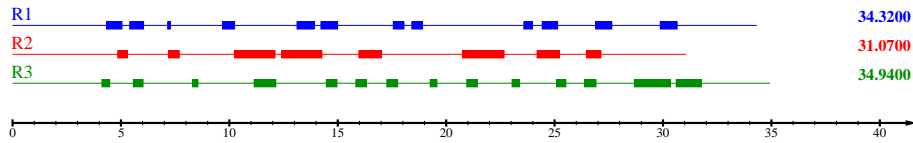
ABBILDUNG 1. Ursprüngliche Roboterschweißpfade.
