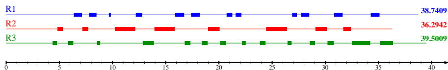
ABBILDUNG 3. Für eine Laserquelle optimierte Roboterschweißpfade.
