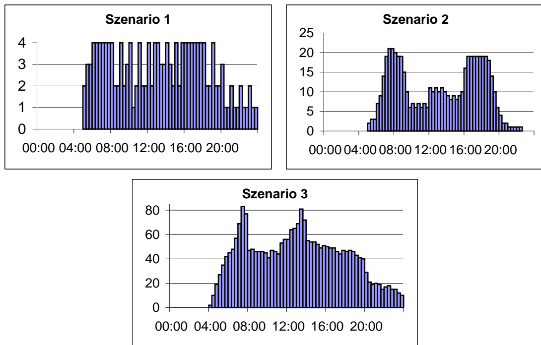
Abbildung 4: Fahrzeitprofile
