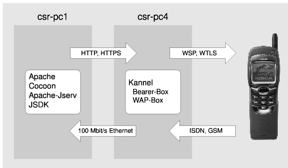
Abbildung 7: Konfiguration der WAP-Testumgebung
