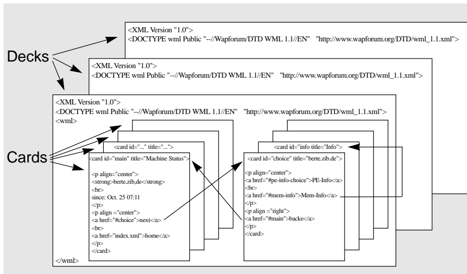
Abbildung 5: WML-Dokument mit seinen Decks und Cards
