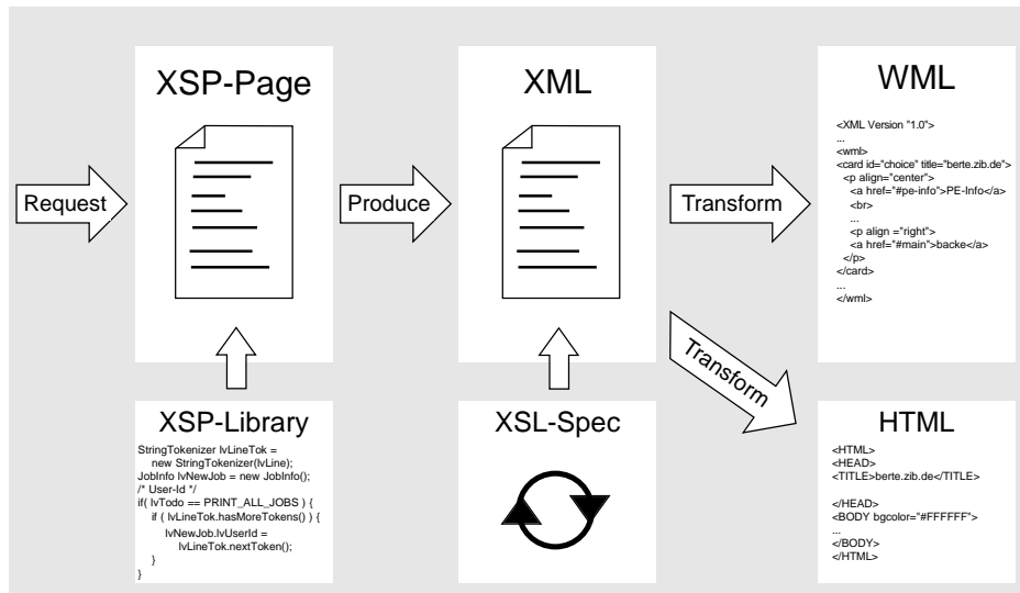
Abbildung 12: Das Cocoon-Verarbeitungsmodell
