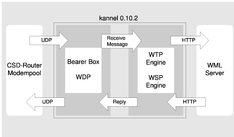
Abbildung 6: Die Kannel-Architektur
