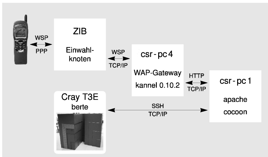
Abbildung 13: Testaufbau des WAP-Service im ZIB
