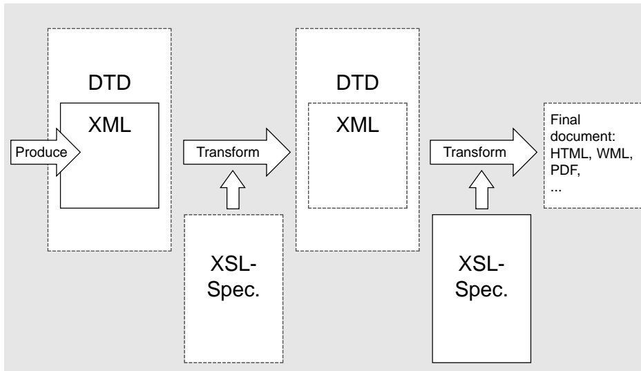
Abbildung 11: Das XML-Verarbeitungsmodell
