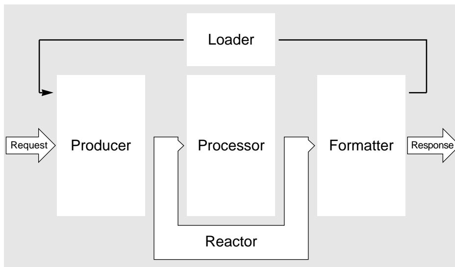
Abbildung 14: Das Cocoon-Verarbeitungsschema
