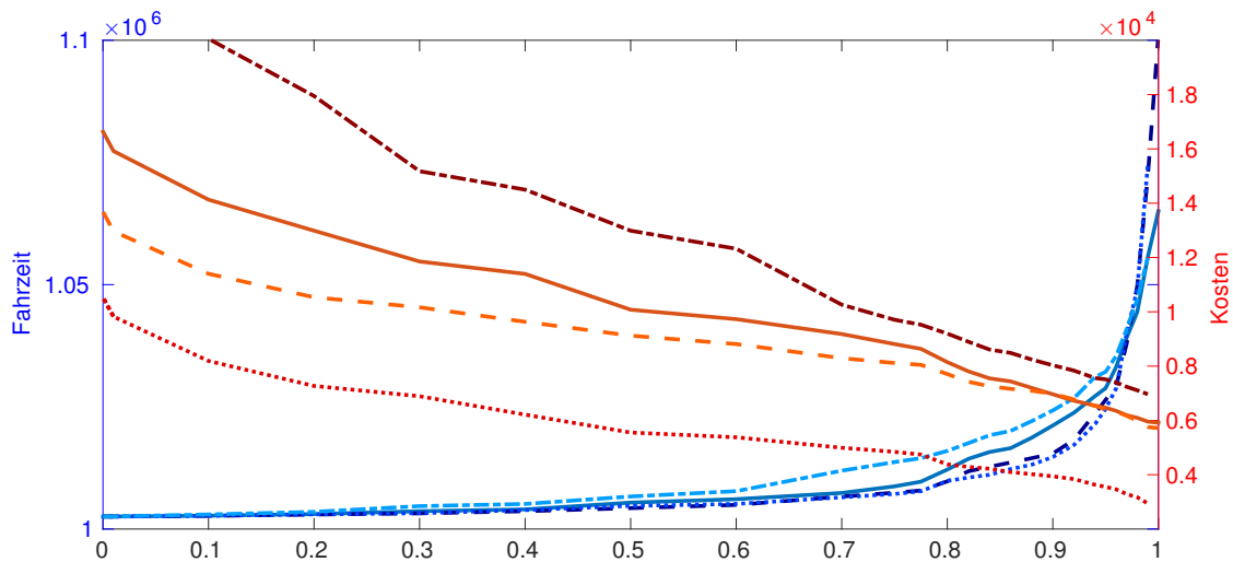
Abbildung 3: Pareto-Kurven für Szenario 1 „Standardtakt“ (gepunktet), Szenario 2 „Mindestbedienhäufigkeit“ (gestrichelt), Szenario 3 „Mindestbedienhäufigkeit + Tram“ (durchgezogen) und Szenario 4 „Mindestbedienhäufigkeit + Tram + Takt“ (gestrichpunktet). Abhängig von dem Wert eines Parameters \lambda (Werte zwischen 0 und 1) werden Kosten und Fahrzeiten (in Minuten, mit Umsteigestrafe) für die Zielfunktion prozentual gewichtet. Ein Wert von 1 bedeutet, nur die Kosten sind wichtig (100%=1) und die Fahrzeiten unwichtig (0%=0), ein Wert von 0 bedeutet das Gegenteil.
