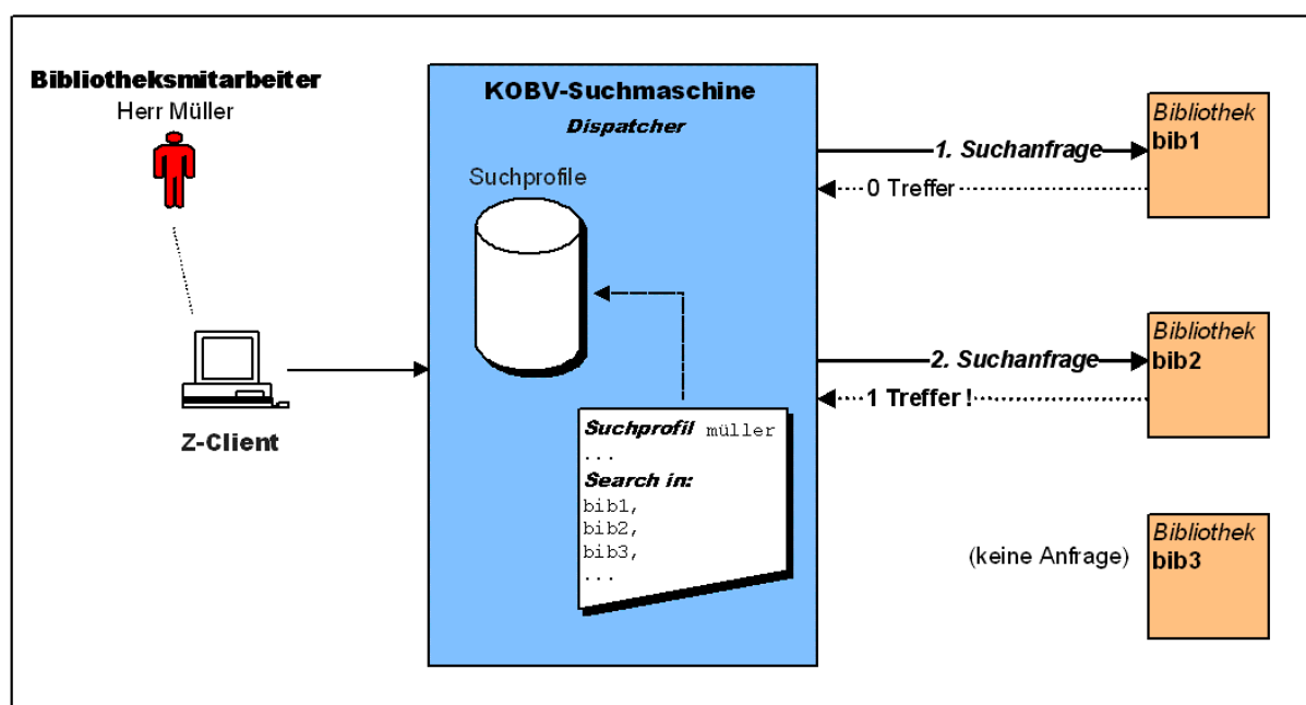
Abbildung 6: Sequentiell verteilte Suche
