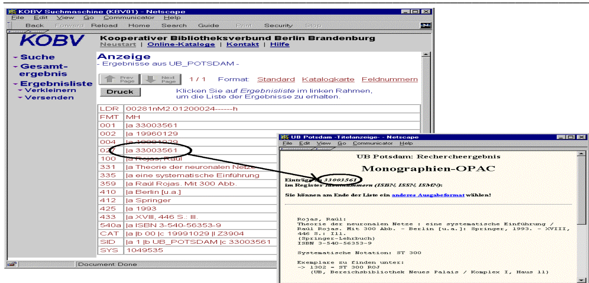
Abbildung 5: WEB-Link Funktion
