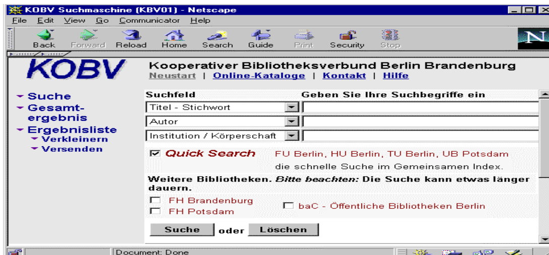
Abbildung 3: Suchmaske (Bildschirmausdruck)
