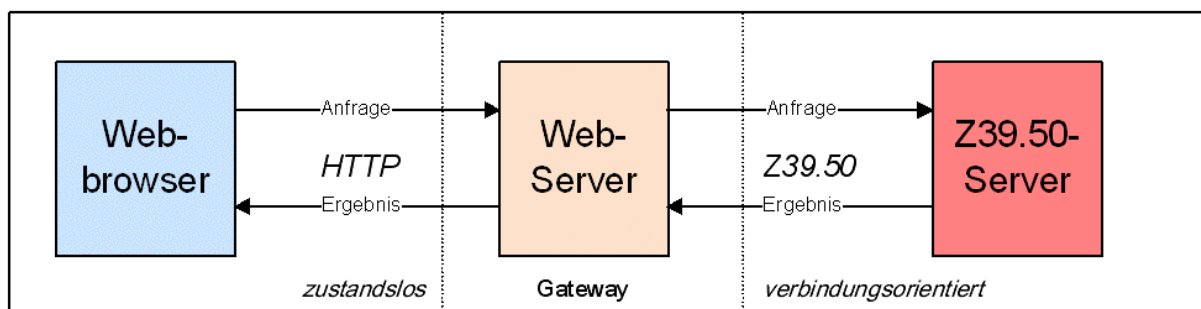
Abbildung 2: WWW-Z39.50-Gateway
