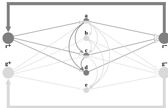
Abb. 3. "Geschumpfter" Digraph (V', A') .
