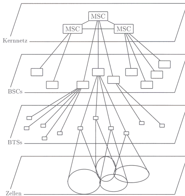
Abbildung 1. Hierarchische GSM-Infrastruktur
