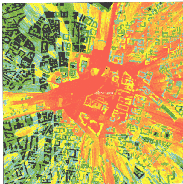
Abbildung 3. Prädiktion der Signalstärke einer GSM-Antenne
