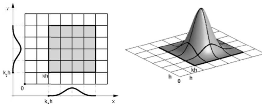
Abb. 3: Konstruktion in \mathbb{R}^2 (links), B-Spline in \mathbb{R}^2 (rechts)
