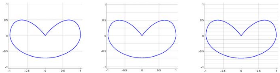
Abbildung 6: Verfeinerung des Gitters in y -Richtung
