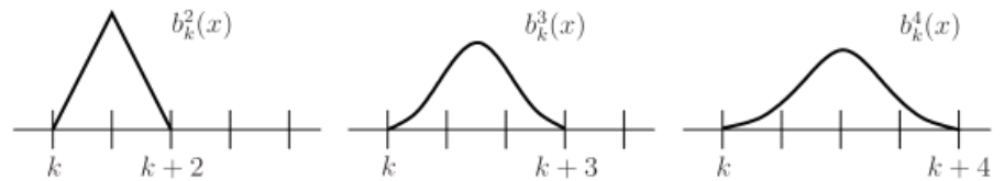
Abb. 2: B-Splines der Ordnung 2, 3 und 4 mit Knoten aus den ganzen Zahlen
