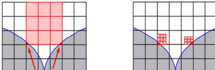
Abb. 5: Träger mit zwei Schnittbereichen im Gebiet (links), kopierter und
