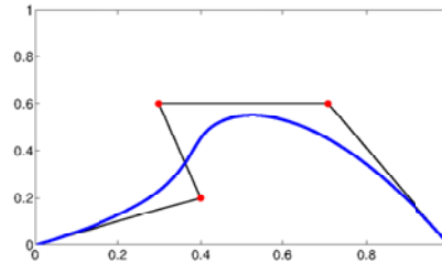
Abb. 3: Splinekurve der Ordnung 4 mit 5 Kontrollpunkten
