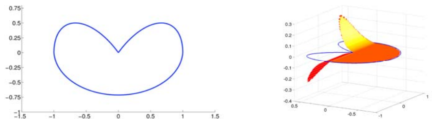
Abb. 1: Gebiet im \mathbb{R}^2 (links), zu approximierende Funktion (rechts)
