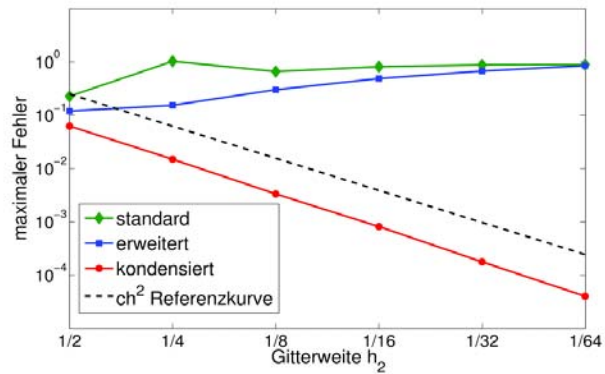
Abbildung 7: Approximationsfehler bei Verfeinerung der Gitterweite h_2
