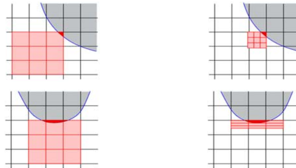
Abb. 4: Träger mit kleinen Schnittbereichen (links), kondensierte Träger (rechts)
