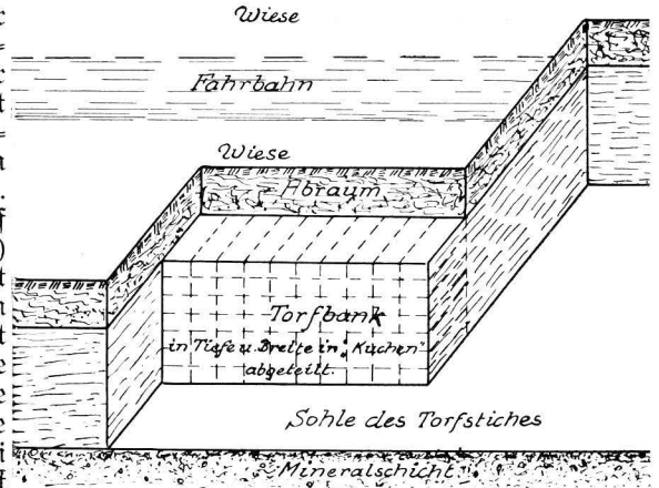
Darstellung eines Torfstiches / Zeich.: Kulturbaumeister Braach.
