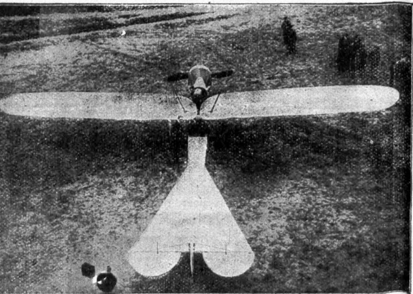
Ein zusammenklappbarer Flugapparat in Insektenform.
