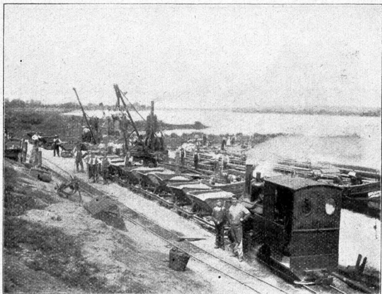
Oder-Umschlagstelle der Oderbruchbahn in Kienitz.
