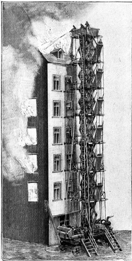
Die nach Art der „Nürnberger Schere“ konstruierte neue Feuer-Rettungsleiter während des Gebrauches bei einem Brande.
