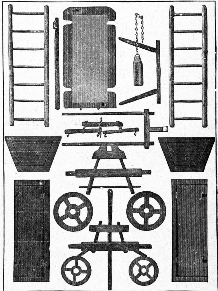
Abb. 1. Der Ackerwagen in seine Teile zerlegt.
