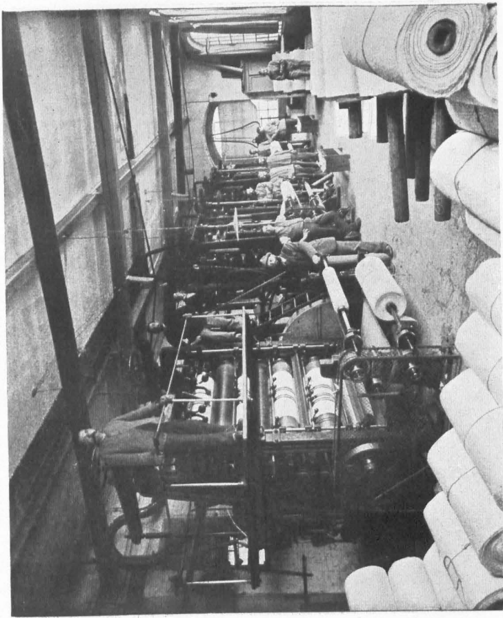
Kalanderraum: Auf den übereinanderliegenden Walzen erscheint das Papier, das hier Glanz und Glätte erhält.
