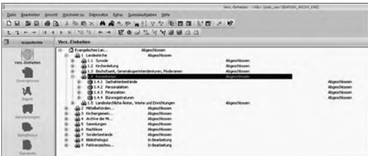
Anlage 1: Baumstruktur.
