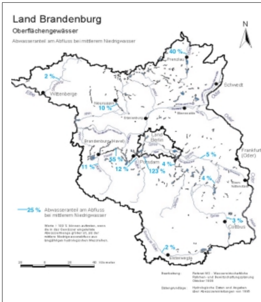
Abb. 2: Abwasseranteil in größeren Brandenburger Fließgewässern
