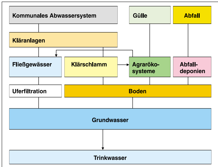
Abb. 1: Eintragungspfade für Humanarzneimittelwirkstoffe in die Umwelt
