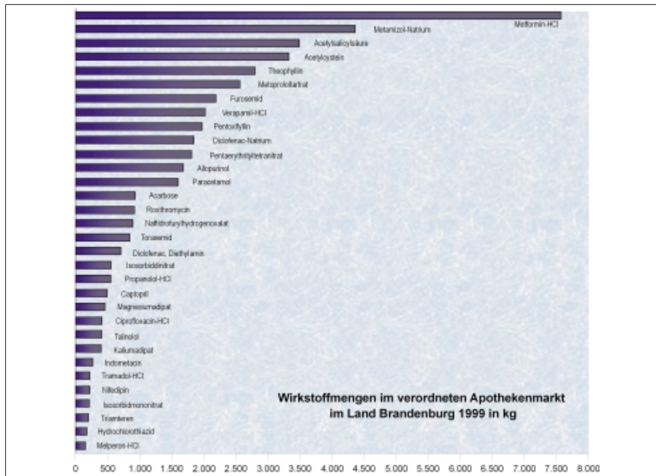
Abb. 3: Wirkstoffmengen im verordneten Apothekenmarkt im Land Brandenburg 1999 in kg
