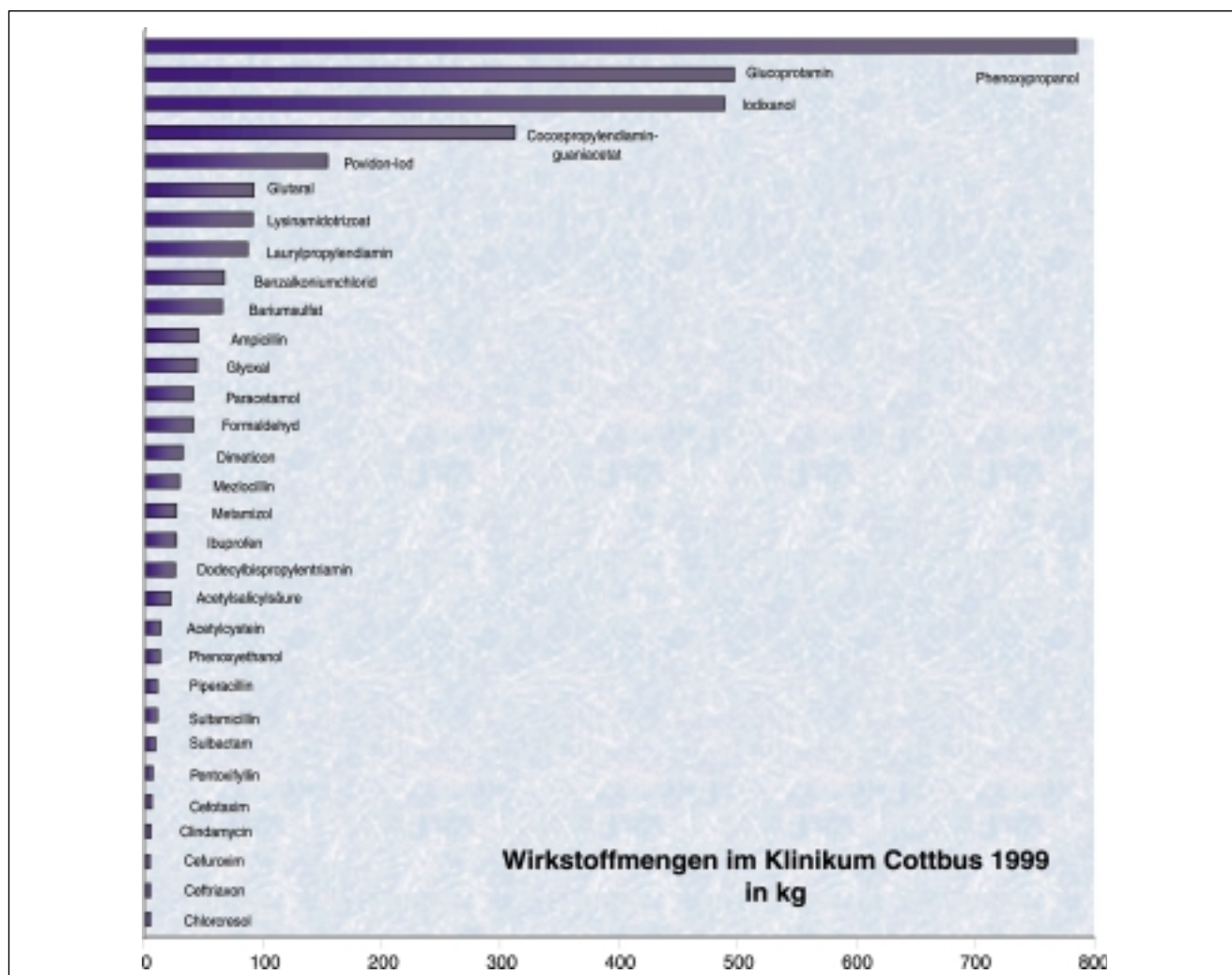
Abb. 4: Wirkstoffmengen im Klinikum Cottbus 1999 in kg
