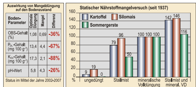
Relativerträge ausgewählter Nutzpflanzen in Abhängigkeit von der Düngung auf schwach schluffigem Sandboden im 9-jährigen Mittel (GÄBERT, 2010).
