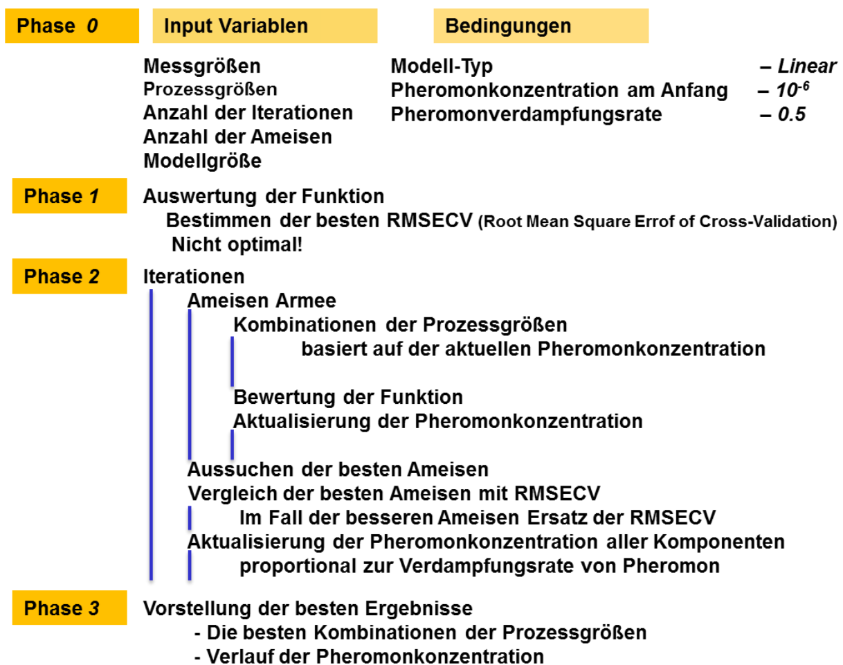
Abbildung 7: Schema eines ACO-Algorithmus.
