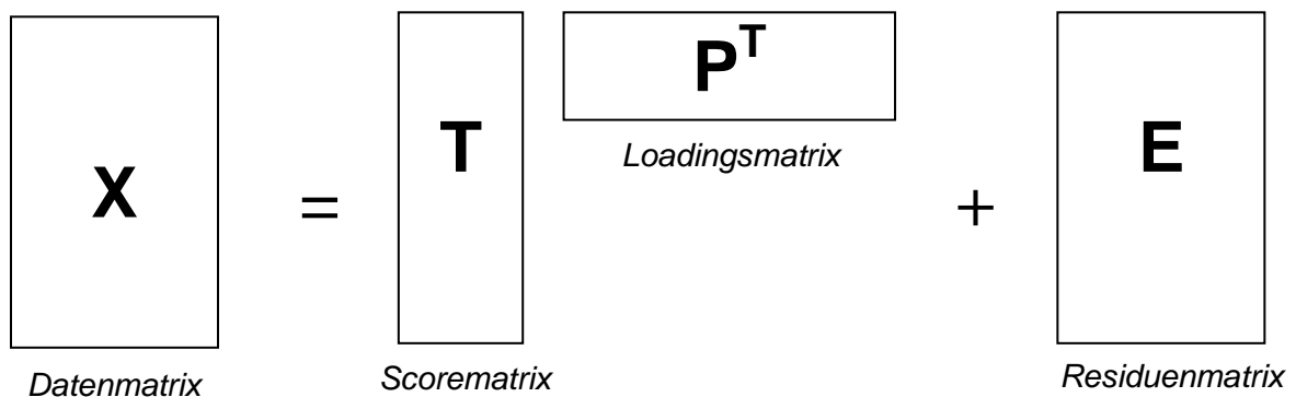
Abbildung 5: Die Hauptkomponentenanalyse (PCA).
