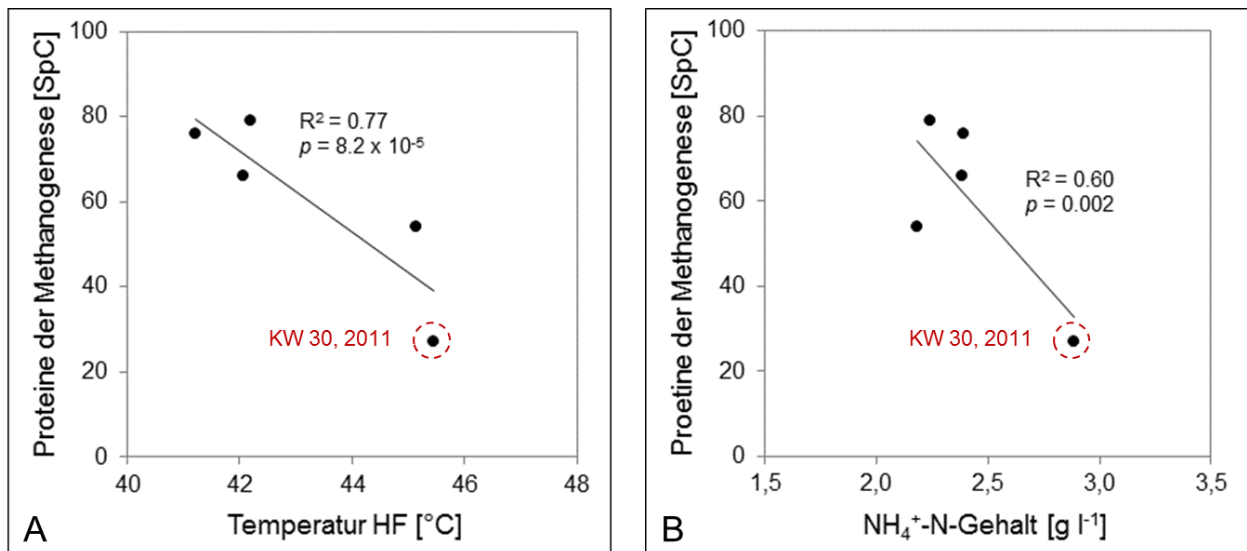
Abbildung 7: Korrelation der Methanogeneseproteine mit der Prozesstemperatur (A) und dem Ammoniumstickstoffgehalt im Gärrest (B). Dargestellt ist die lineare Regression mit dem Korrelationskoeffizienten ( R^2 ) und der statistischen Signifikanz ( p -Wert).
