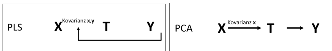
Abbildung 6: Unterschied zwischen der PCR- und PLSR- Methoden.
