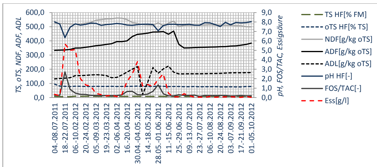
Abbildung 2: Verlauf der chemischen Messdaten der BGA Erchinger (03).
