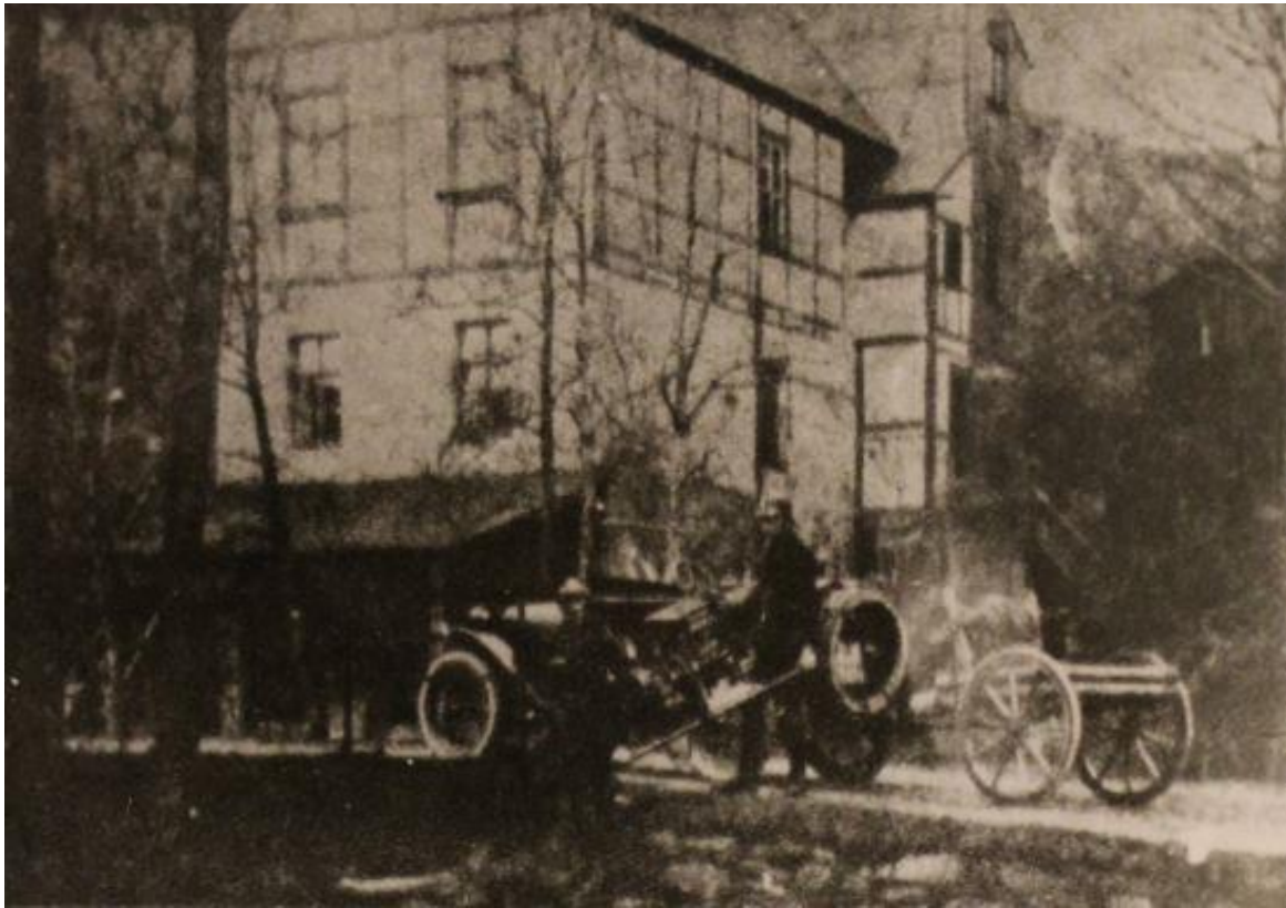
Umgebauter größerer PKW als Zugfahrzeug für einen TSA mit offener Bauausführung
