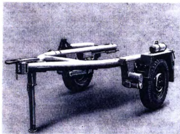
Fahrgestell ausgefahren
