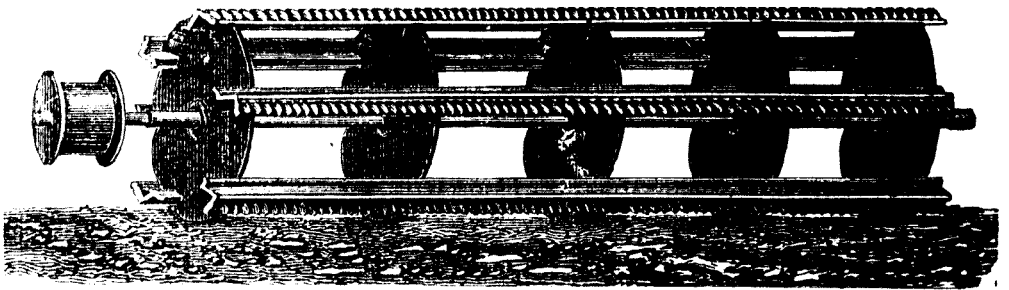
Neue Victoria-Dreschtrömmel.
