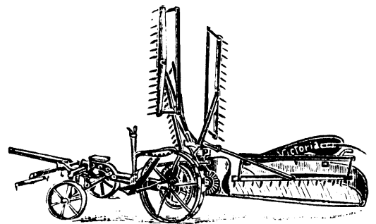
Uiktorja-Getreidemäher mit Vordergestell.
