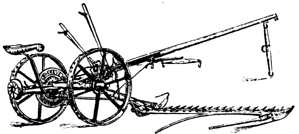
„Buckeye“ Grasmäher
