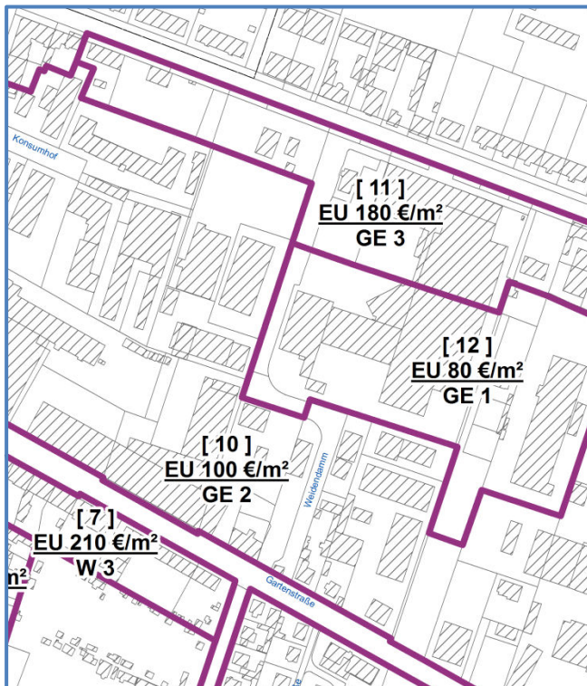
Abb. 60 Auszug aus der Bodenrichtwertkarte "Besondere Bodenrichtwerte im Entwicklungsbereich Babelsberg" (Stichtag 31.12.2016)
