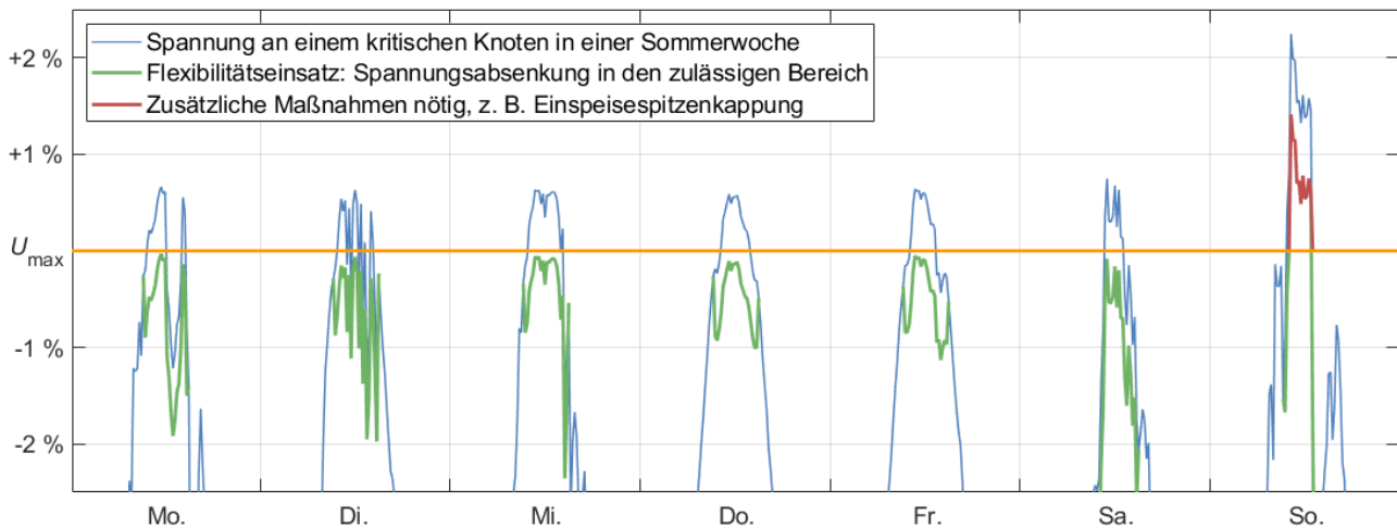
Abbildung 3: Beispiel für die spannungssenkende Wirkung eines Flexibilitätseinsatzes
