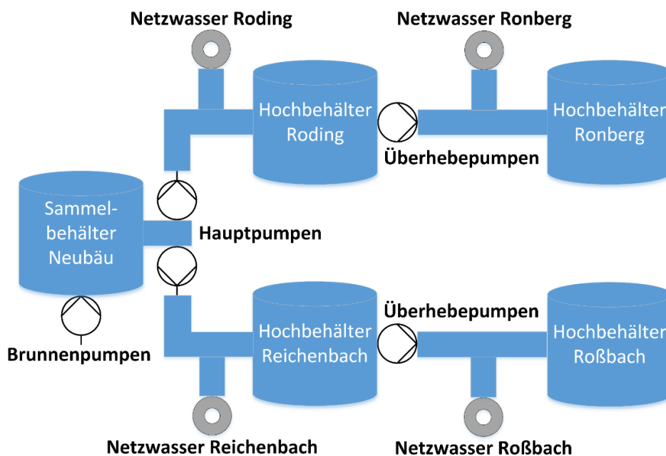
Abbildung 9: Schematischer Aufbau des Pumpenmodells der Kreiswerke Cham
