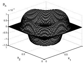
FIG. 5.4. Adjoint state p_h .
