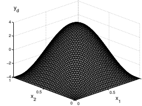
FIG. 5.1. Desired state y_d .
