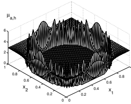
FIG. 5.10. Lagrange multiplier \mu_{a,h} .
