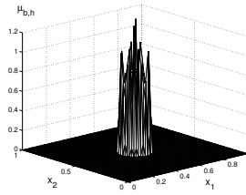
FIG. 5.11. Lagrange multiplier \mu_{b,h} .
