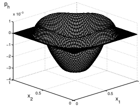
FIG. 5.9. Adjoint state p_h .
