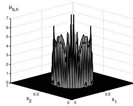
FIG. 5.6. Lagrange multiplier \mu_{b,h} .
