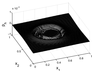
FIG. 6.35. Adjoint state p_h
