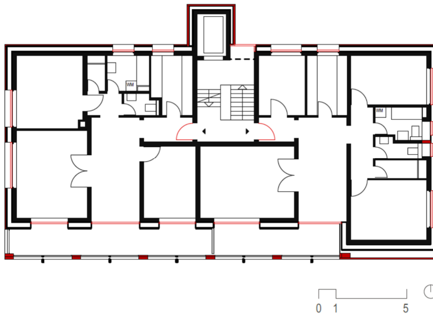
Bild 5.27: Grundriss 1.-8.OG (Neubau ist rot dargestellt) - Generalsanierung Wohnhochhaus Pforzheim
