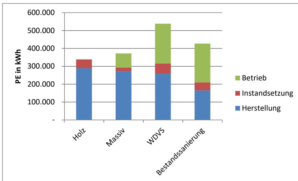
Bild 5.39: Haus Simpel – Primärenergiebedarf im Vergleich der Konstruktionsalternativen
