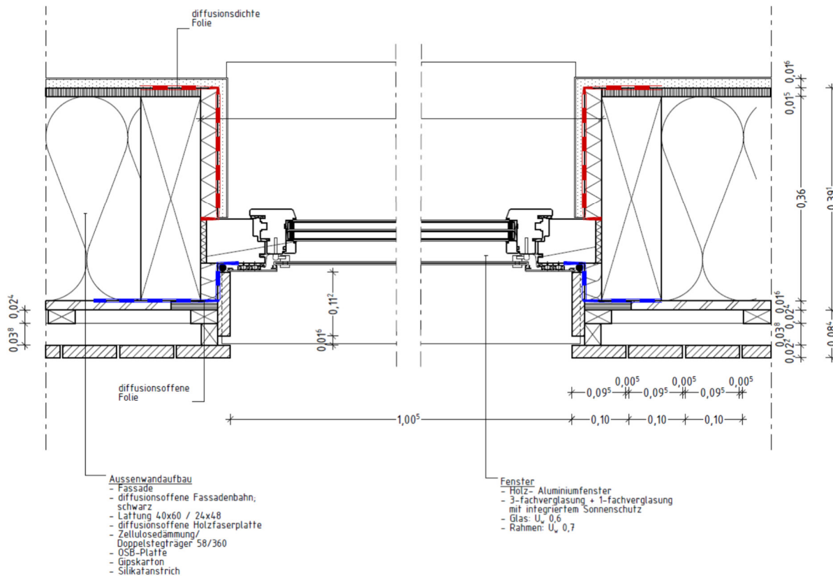
Bild 5.5: horizontaler Fassadenschnitt – Haus 2019
