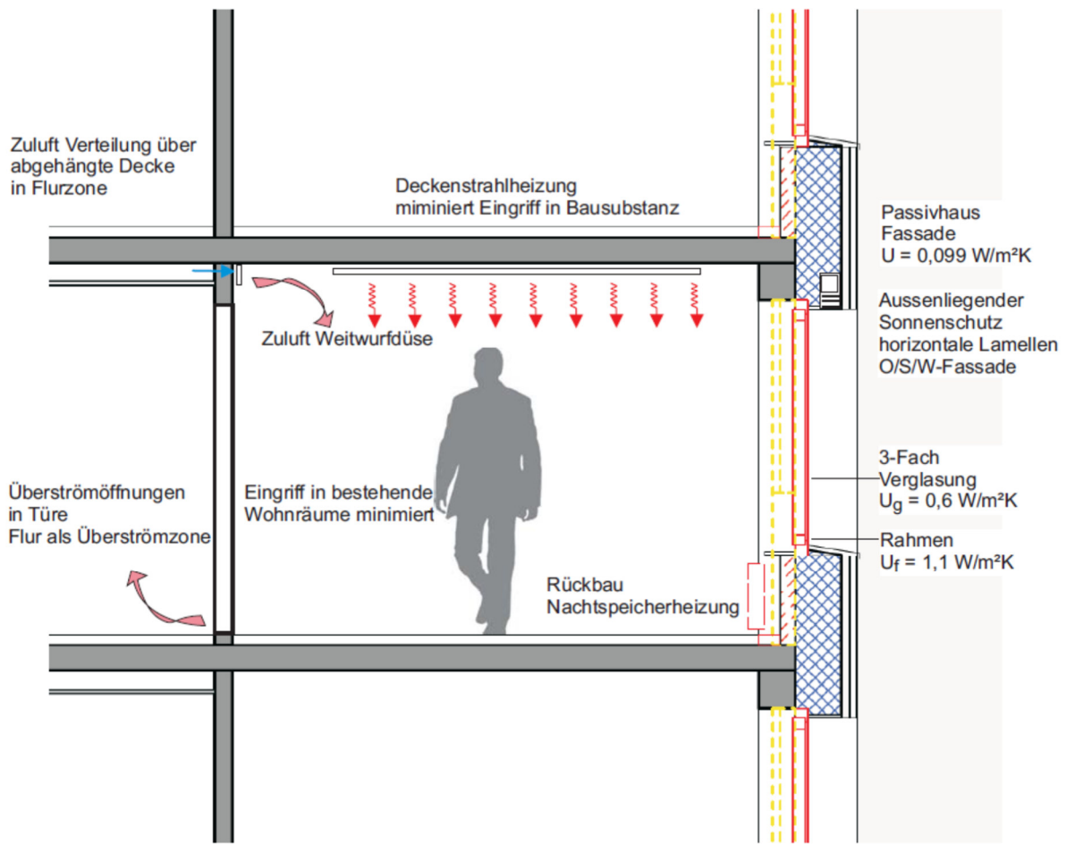
Bild 5.30: Energiekonzept im Detail – Generalsanierung Wohnhochhaus Pforzheim
