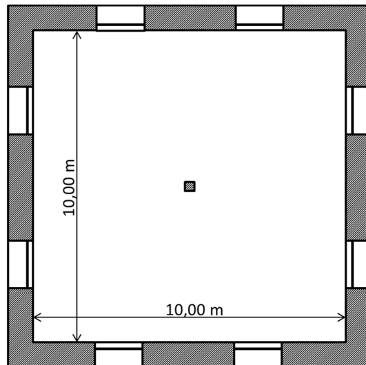
Grundriss
