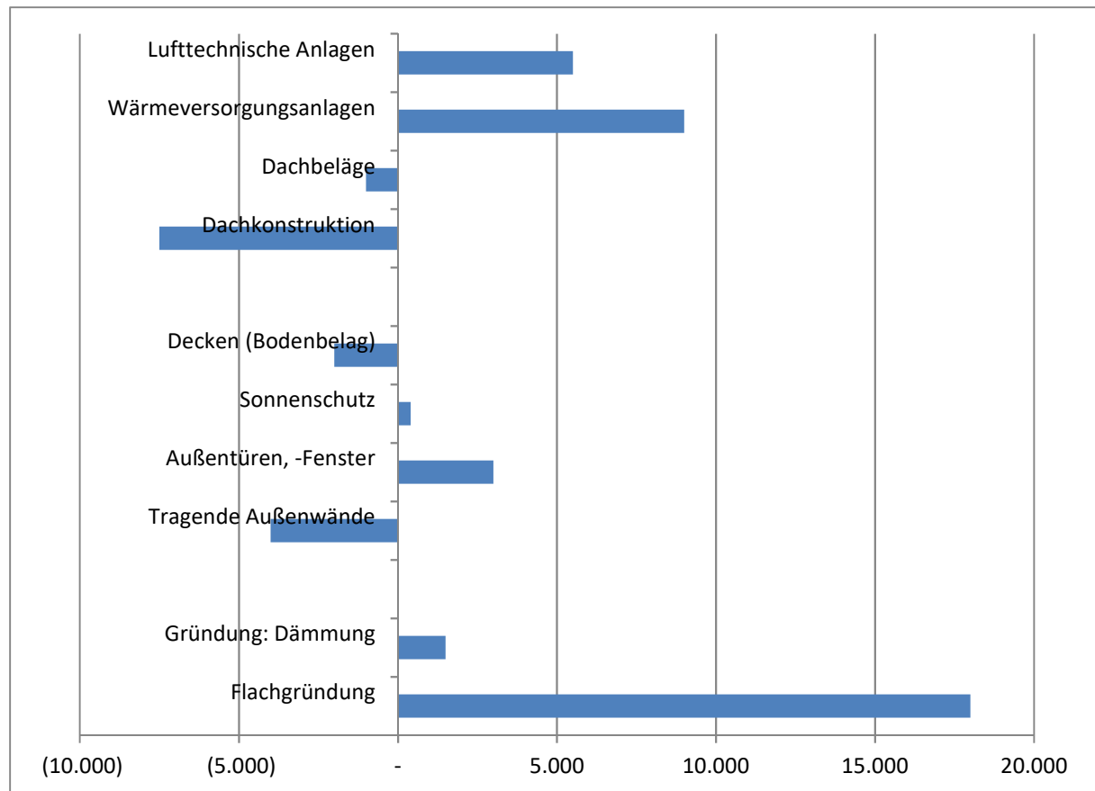
Bild 4.3: CO 2 -Bilanz für Holzbau (vgl. Haus Simpel)
