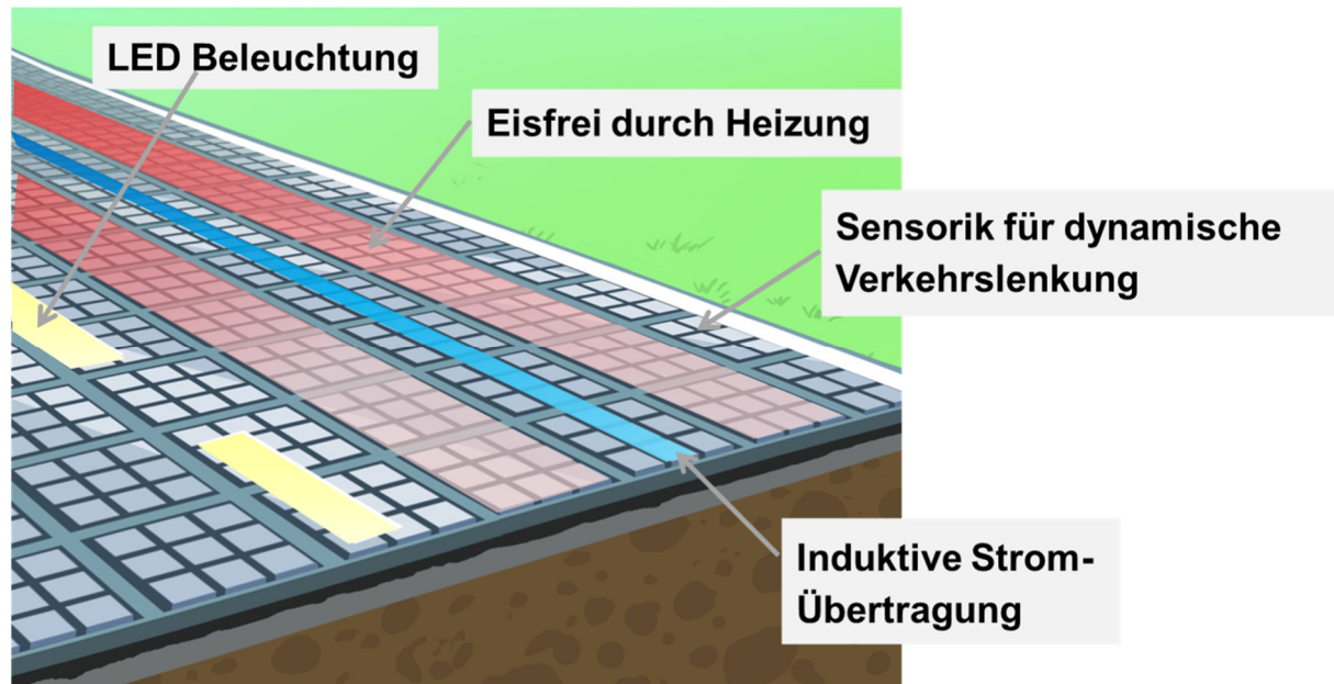
Bild 4.7: Photovoltaik im Straßenbelag – Optionen für die Nutzung
