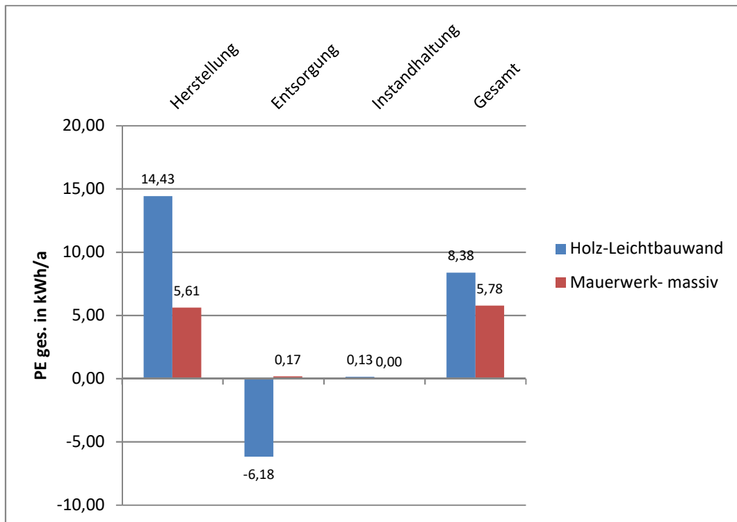
Bild 3.20: Primärenergieaufwand (PE gesamt) je nach Wandkonstruktion bei 50 Jahren Lebensdauer (je 1m 2 und Jahr)
