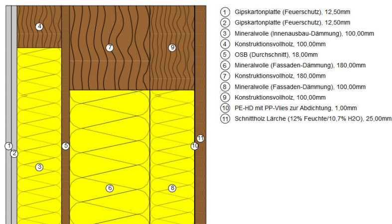
Bild 3.18: Leichtbauwand aus Holzwerkstoffen und Dämm-Material
