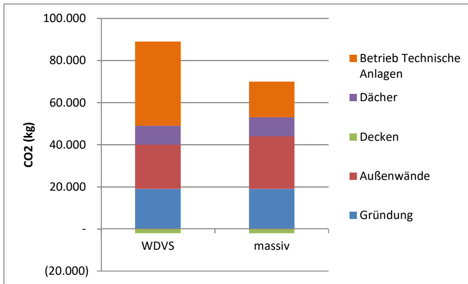
Bild 5.38: CO 2 -Anteile je Bauelement und Fassadenalternative - „Haus Simpel“
