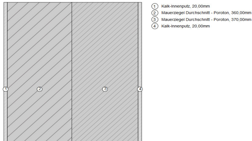
Bild 3.17: Mauerwerkswand mit Kalkputz (innen und außen)
