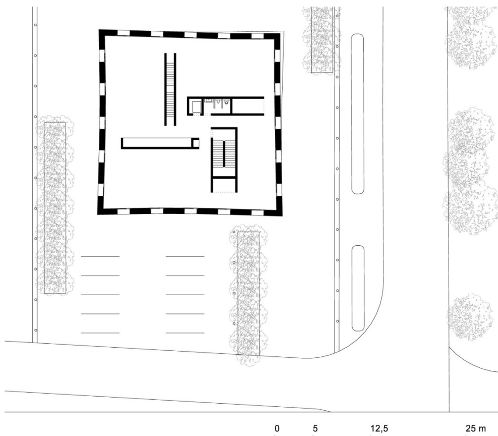
Bild 5.14: Grundriss - Haus 2226 in Lustenau
