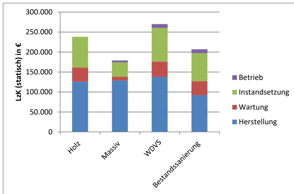
Bild 5.40: statische LzK (gesamt) im Vergleich der Konstruktionsalternativen - Haus Simple
