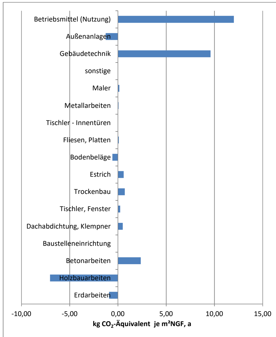
Bild 5.12: CO 2eq je nach Bauelement im Lebenszyklus - Haus 2019
