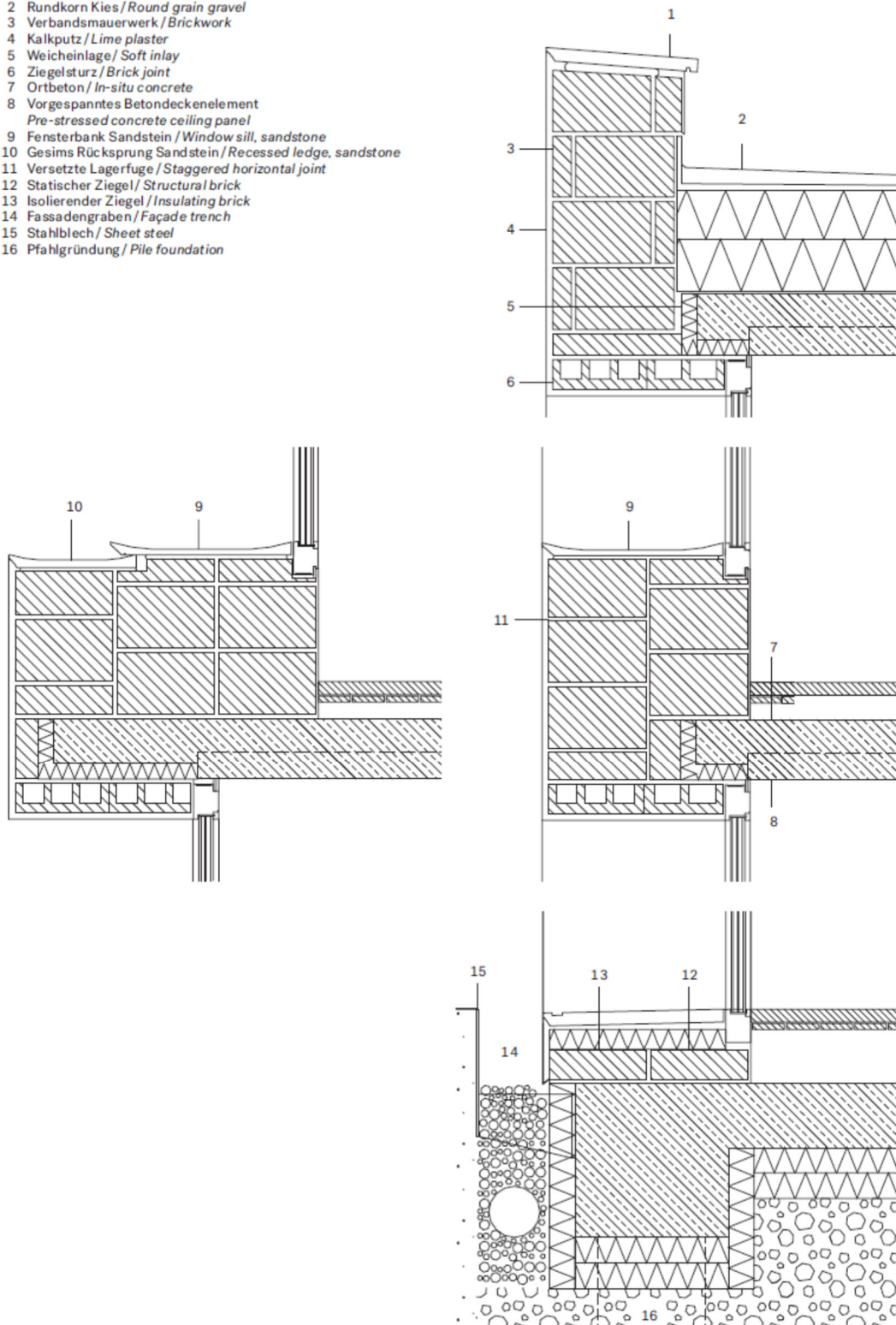
Bild 5.19: Konstruktionsdetails – Haus 2226
