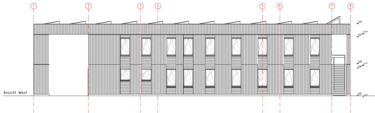
Bild 5.2: Ansicht - Haus 2019
