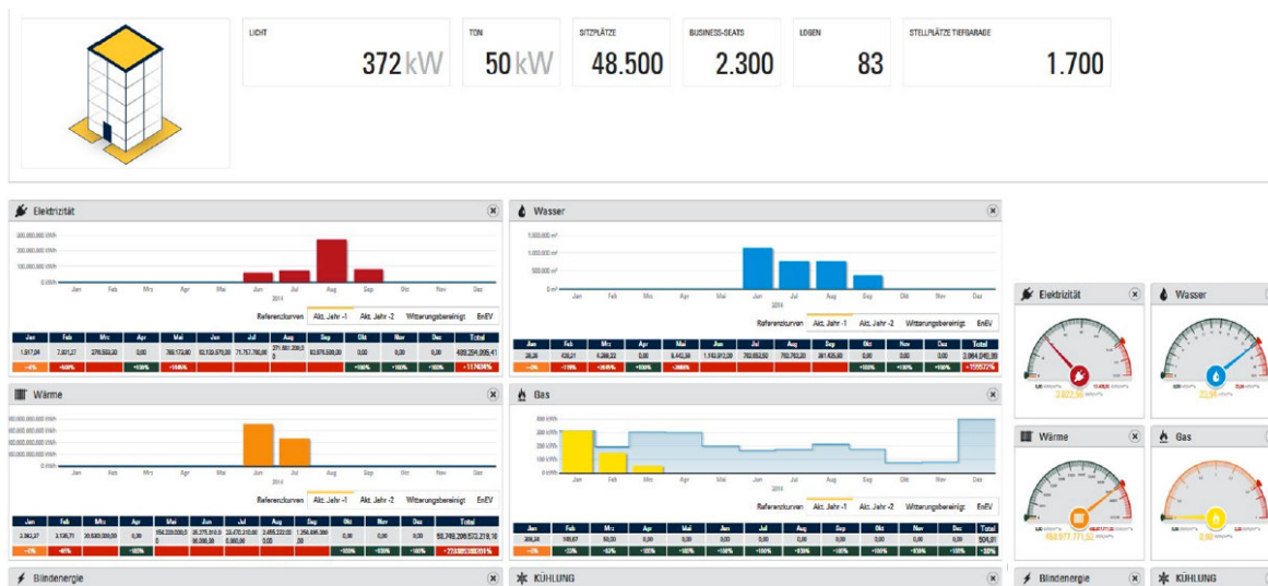
Bild 3.28: Grafische Auswertung der gemessenen Daten (enerlutec, Bilfinger, 2015)
