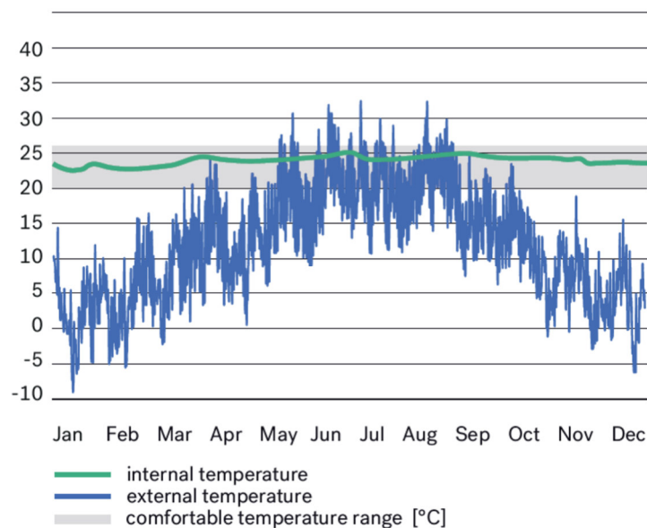
Bild 5.21: Haus 2226 – Innen- und Außentemperatur im Jahresdurchschnitt
