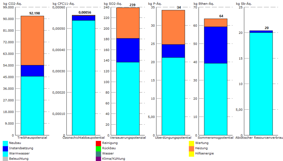
Bild 2.12: Screenshot Legep, Wirkungsbilanz für „Haus Simple“ mit Wärmedämmverbundsystem-Fassade
