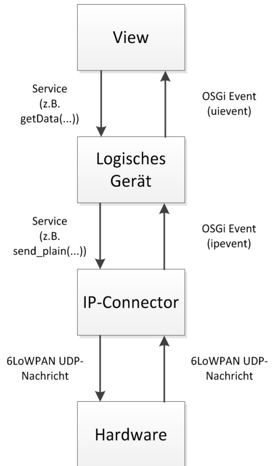
Bild: 1 OSGI-Bundle Struktur des Informatiklabors
