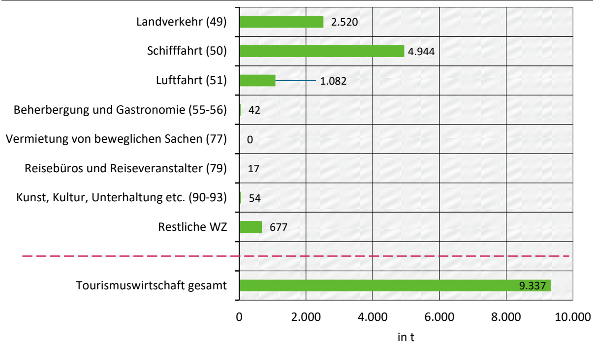
Abbildung 29: Tourismusinduzierter Feinstaubausstoß (PM 2,5 ) nach Wirtschaftsbereichen (2019)
