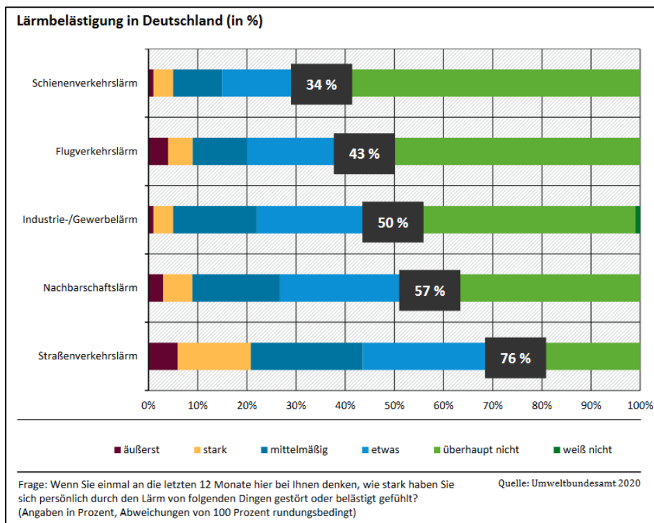
Abbildung 52: Lärmbelastigung in Deutschland
