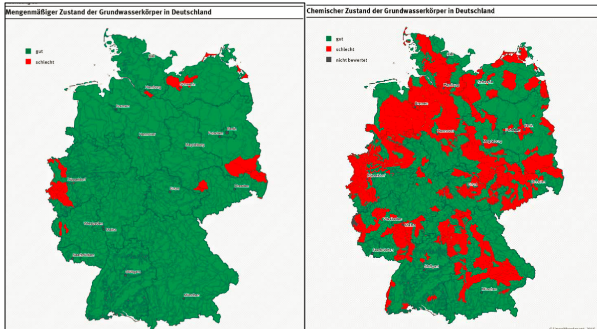
Abbildung 57: Mengenmäßiger und chemischer Zustand der Grundwasserkörper in Deutschland
