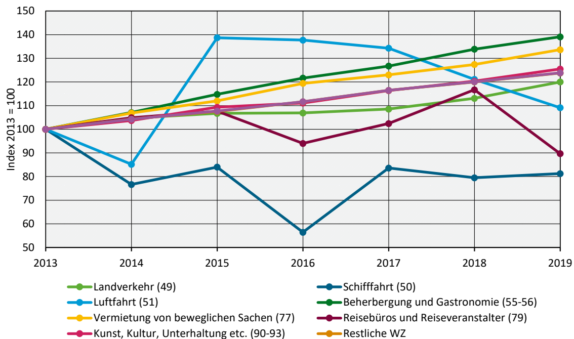
Abbildung 13: Entwicklung der Bruttowertschöpfung in den tourismusrelevanten Wirtschaftsbereichen
