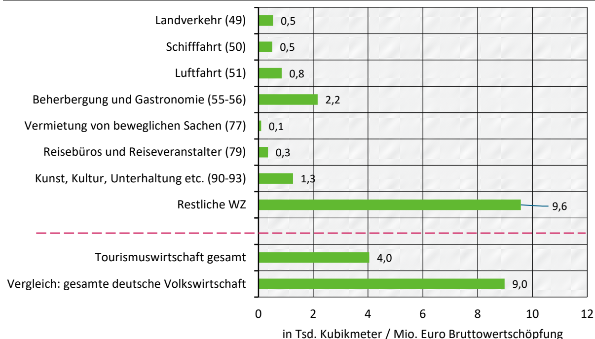
Abbildung 33: Wasserintensität der tourismusrelevanten Wirtschaftsbereiche, der Tourismuswirtschaft und der gesamten deutschen Volkswirtschaft (2016)
