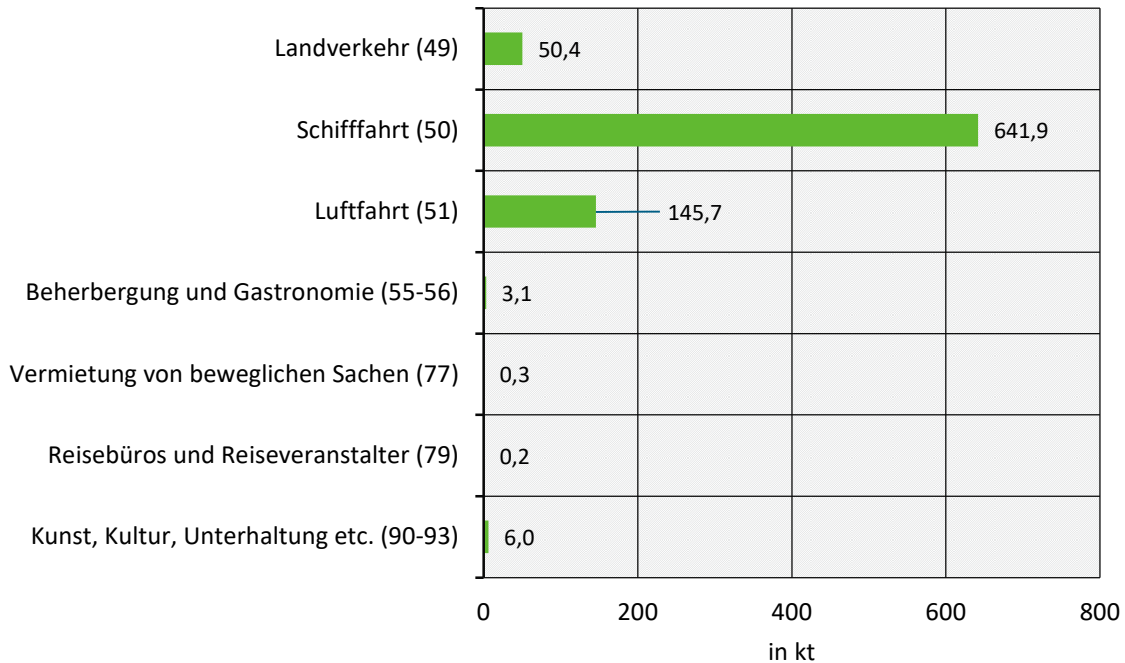
Abbildung 22: NOx-Emissionen der tourismusrelevanten Wirtschaftsbereiche (2019)
