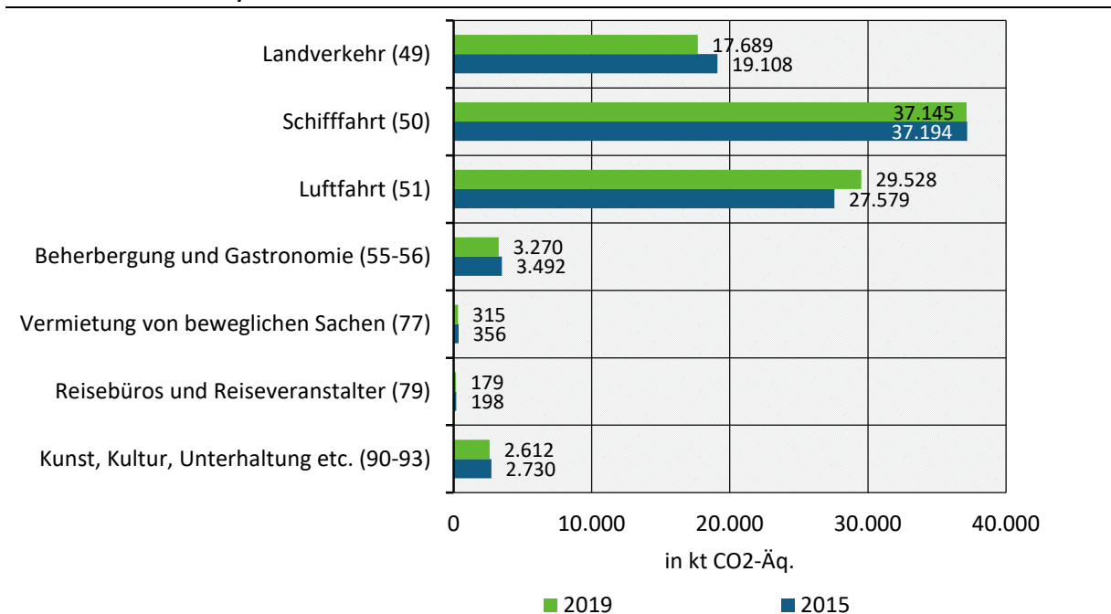
Abbildung 19: Treibhausgasemissionen der tourismusrelevanten Wirtschaftsbereiche (2019 vs. 2015)
