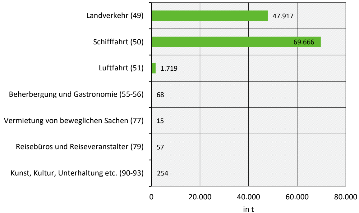
Abbildung 25: PM 10 -Emissionen der tourismusrelevanten Wirtschaftsbereiche (2019)
