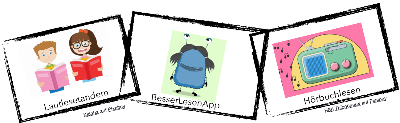
Abb 4: Lautleseverfahren.
