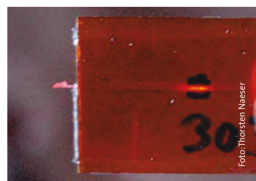
Zur einfacheren Handhabung der Fasersensoren entwickelter «Optischer Dehnmessstreifen».
