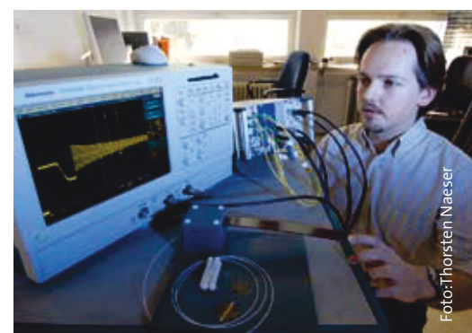
Im Labor für Optoelektronik entwickelte Auswertevorrichtung für optische Fasersensoren zur Aufnahme der Bewegungsfrequenz von Probanden in einem NMR.
