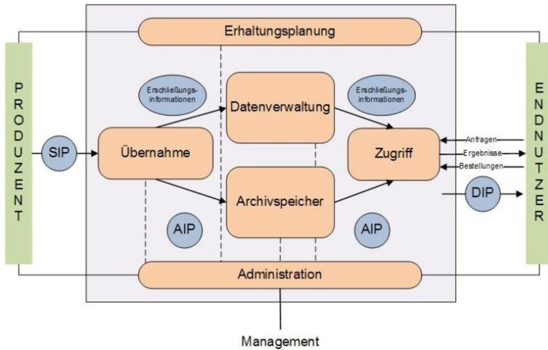
Abbildung 1: OAIS-Funktionseinheiten 1
