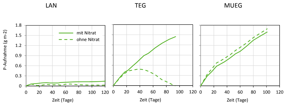
Abbildung 2.36. Kumulative P-Aufnahme der Sedimente vom LAN (links), TEG (Mitte) und MUEG (rechts) während des zweiten, anaeroben Experiments mit und ohne NO 3 -Anwesenheit. Während beim LAN durch die NO 3 -Zugabe eine geringe zusätzliche P-Aufnahme erreicht wurde, zeigen die Sedimente des TEG eine deutlich gesteigerte P-Aufnahme bei NO 3 -Anwesenheit. Die eisenreichen Sedimente des MUEG nehmen unabhängig von NO 3 große Mengen an P auf.
