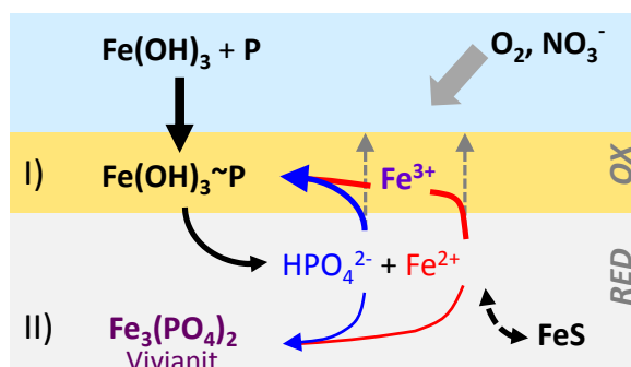
Abbildung 2.29. Prinzipielle Mechanismen der I) reversiblen und II) dauerhaften P-Bindung an Eisen im Sediment von Seen. ( \text{O}_2 -Sauerstoff, \text{NO}_3^- -Nitrat, \text{Fe(OH)}_3 -Eisenhydroxid, \text{FeS} -Eisensulfid, OX-oxidierte Sedimentschicht, RED-reduzierte Sedimentschicht)
