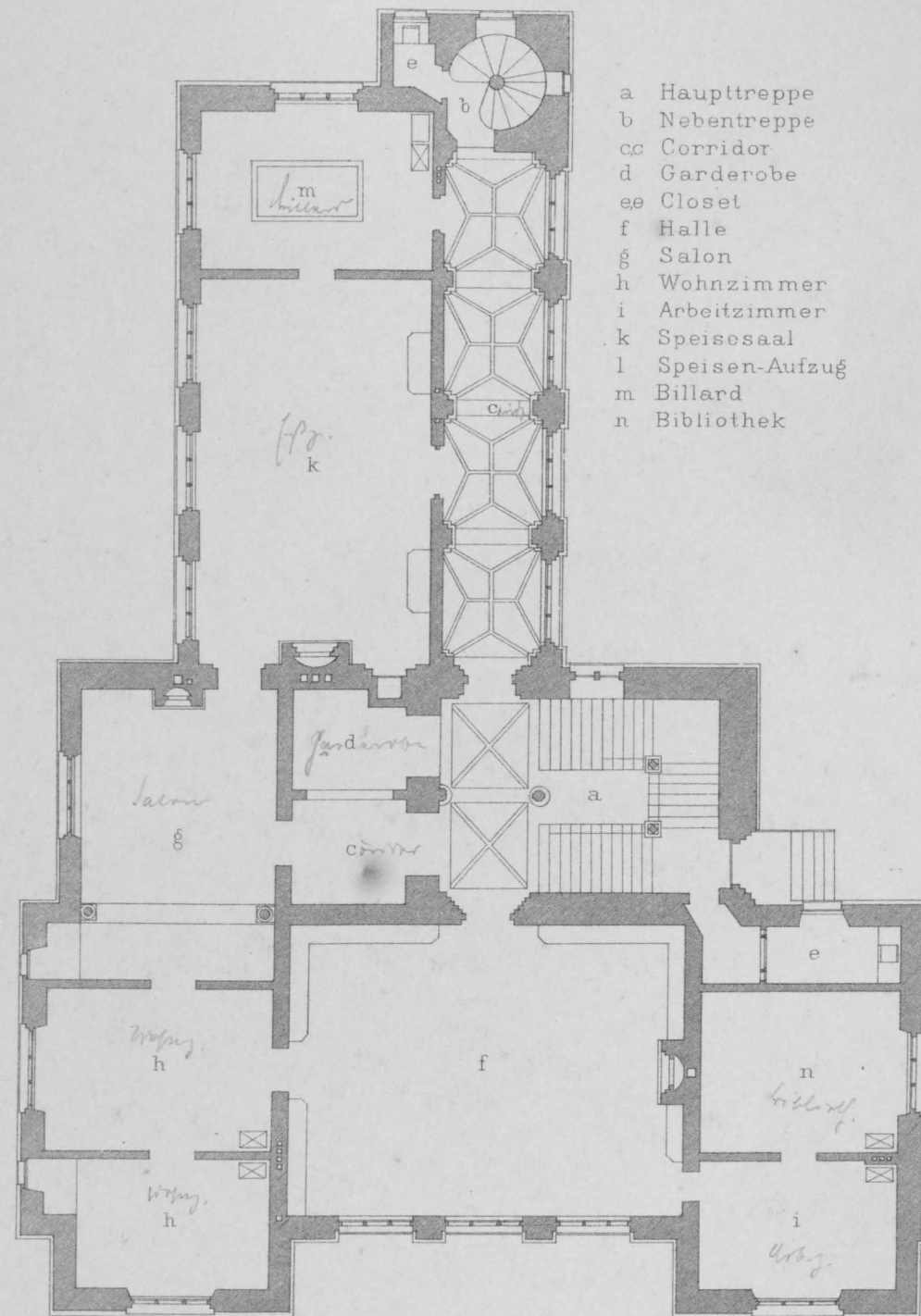
Grundriss des Erdgeschosses
