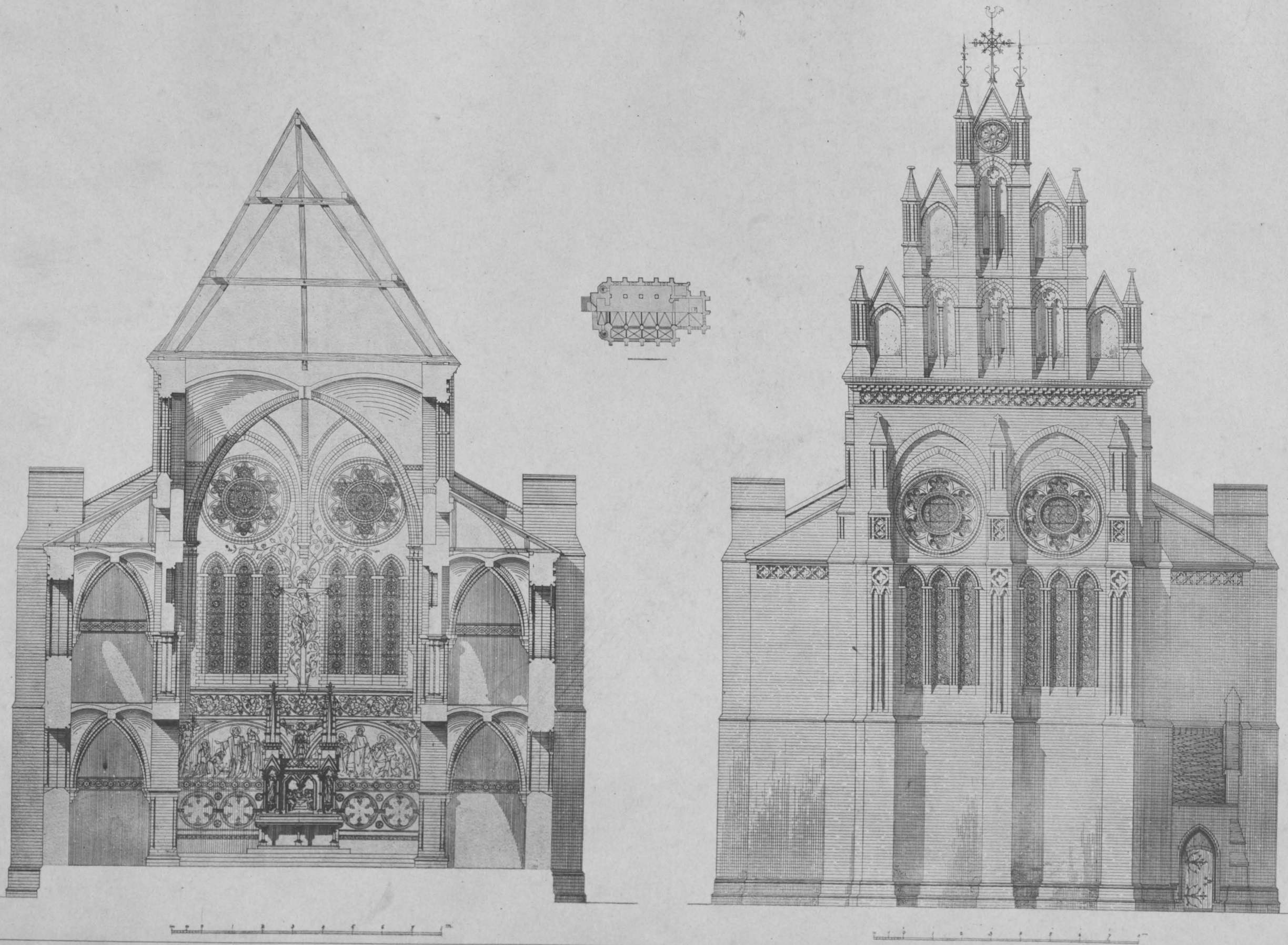
EVANGELISCHE KIRCHE OSTSEITE, QUERSCHNITT, GRUNDRISS
