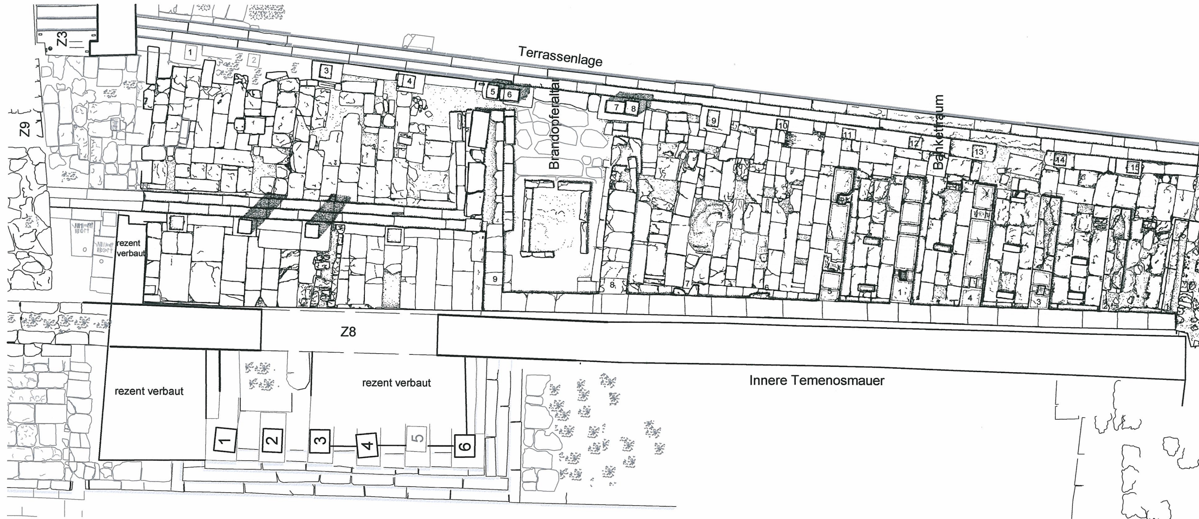
Aufsicht Terrassenanlage und Inneres Propylon
