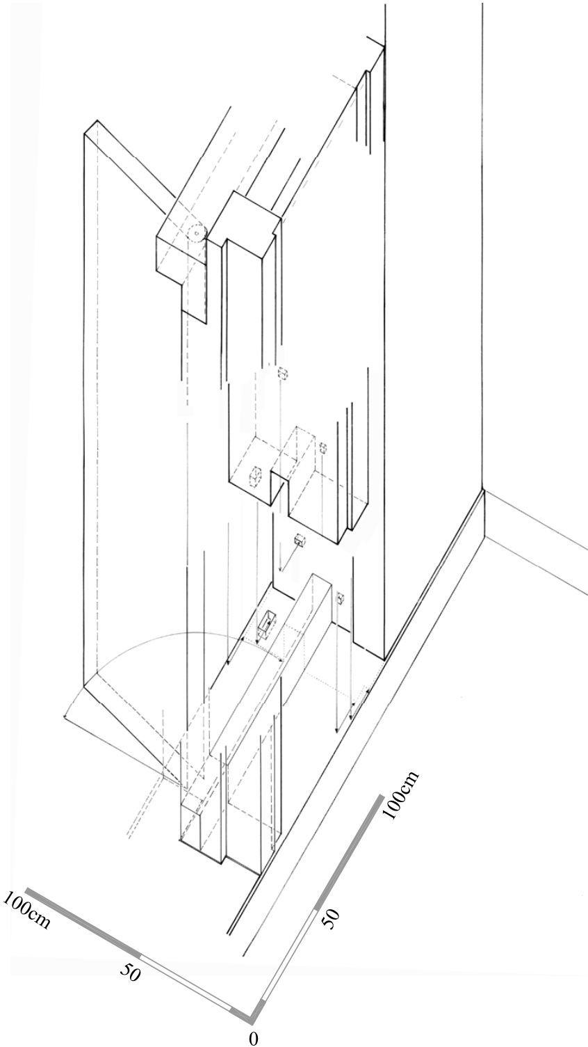
Rekonstruktionsvorschlag Eingangssituation am sog. Schatzhaus
