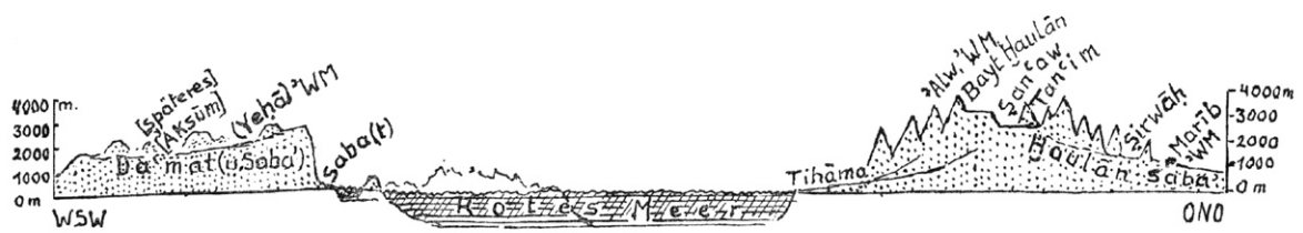
b. Reliefprofil von Aksum (afrikanische Seite) durch das Rote Meer bis Marib (südarabische Halbinsel)
