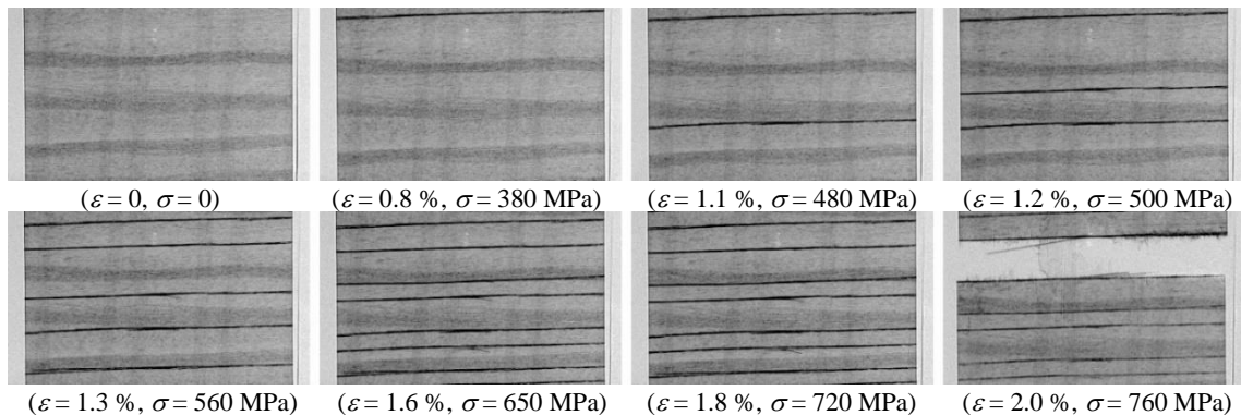
Abb. 5. Ausgewählte SXRR-Aufnahmen des Zugversuchs an der Gelege-Probe 133-3: Beginn des Versuchs, das anschließende Auftreten von 90°-Zwischenfaserrissen bis zum Erreichen einer gesättigten Rissdichte und den anschließenden Bruch. Die Bilder entsprechen einer Größe von 11 \times 7.2 \text{ mm}^2 . Die jeweilige Dehnung ( \varepsilon ) und Spannung ( \sigma ) ist unter jedem Teilbild angegeben.
