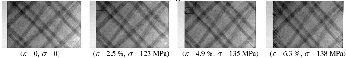
Abb. 6. Ausgewählte SXRR-Aufnahmen des Zugversuchs an der Gelege-Probegewebe 133-17: Beginn des Zugversuchs, den ersten 90°-Riss, die ersten 45°-Zwischenfaserrisse und die Schädigung vor dem Bruch.
