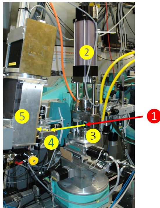
Abb. 3. Versuchsaufbau – Synchrotronstrahlung (monochromatisch, 1), Zugvorrichtung (inkl. Aktuator, Kraftmessdose und Einspannung, 2), Zugprobe (3), Analysatorkristall (4), Flachdetektor (5).
