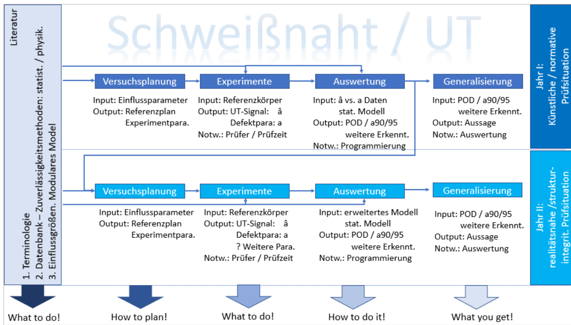
Abb. 4. Ferritische Schweißnahtprüfung im Kraftwerksbereich
