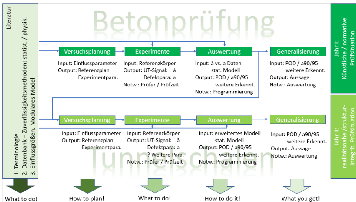
Abb. 5. Prüfung der Tunnelinnenschalen aus Stahlbeton
