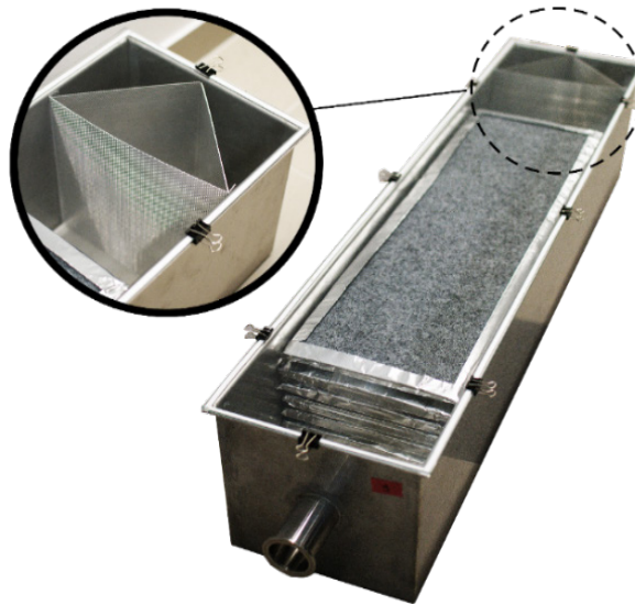
Abbildung 6: CLIMPAQ-Emissionskammer [Quelle: eigene Darstellung, HTW Berlin]
