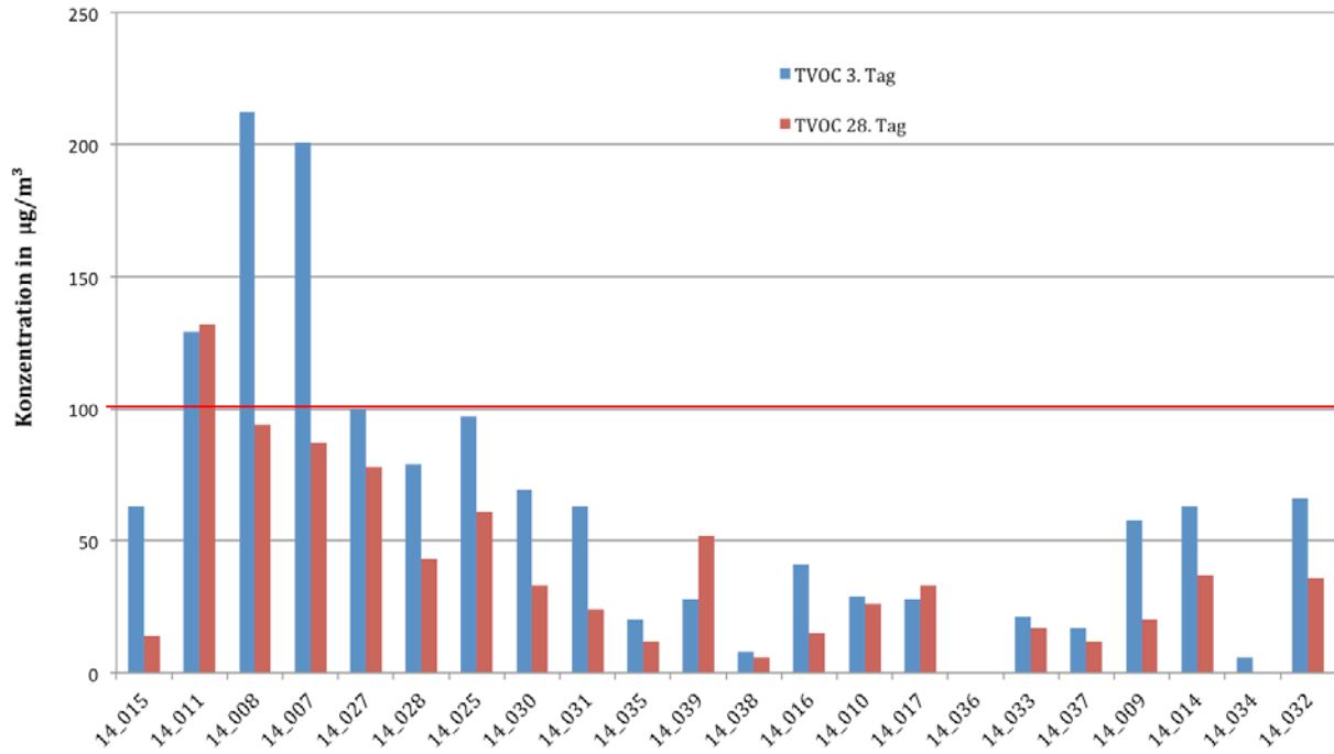
Abbildung 26: TVOC-Werte der AgBB-Auswertung der textilen Bodenbeläge am 3. und 28. Tag (rote Linie: Grenzwert 28. Tag UZ 128 = 100 µg/m³) [Quelle: eigene Darstellung, BAM]
