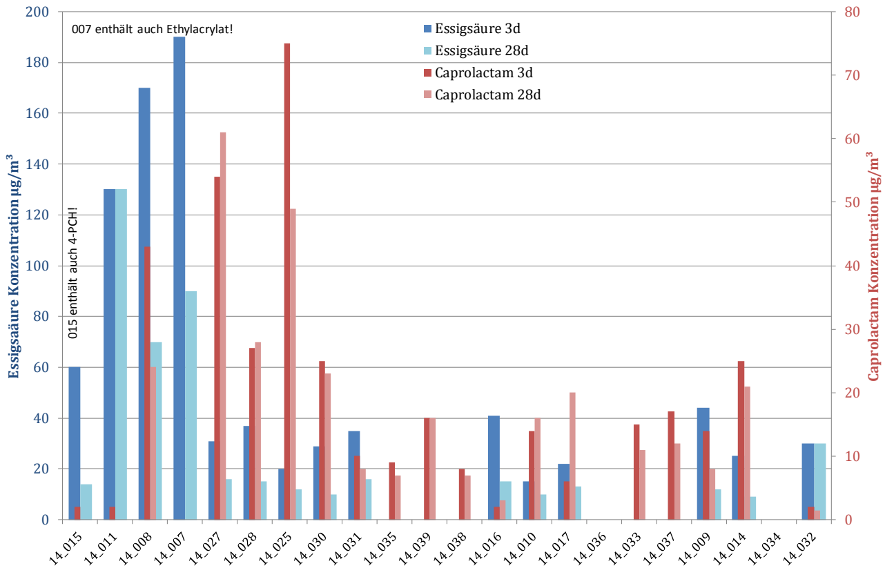
Abbildung 27: Konzentrationen von Essigsäure und Caprolactam der textilen Bodenbeläge [Quelle: eigene Darstellung, BAM]
