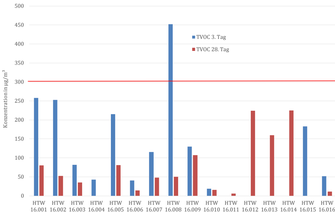
Abbildung Z5: TVOC-Werte der AgBB-Auswertung der elastischen Bodenbeläge am 3. und 28. Tag (rote Linie: Grenzwert UZ 120 = 300 µg/m 3 ) [Quelle: eigene Darstellung, BAM]
