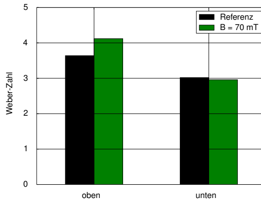
Abbildung 5.9: Vergleich der Weber-Zahlen aus den Simulationen aus Abschnitt 4.1 für die obere und untere Schmelzbadoberfläche ohne und mit elektromagnetischer Unterstützung.
