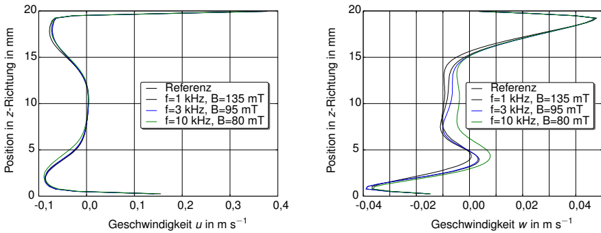
Abbildung 4.18: Geschwindigkeitsverteilungen u in Schweißrichtung sowie in Vertikalrichtung w entlang eines vertikalen Schnittes 3 mm hinter der Dampfkapillare in der Symmetrieebene des Schmelzbades für eine Schweißgeschwindigkeit von 0,3 m/min bei 20 mm dickem AISI 304.
