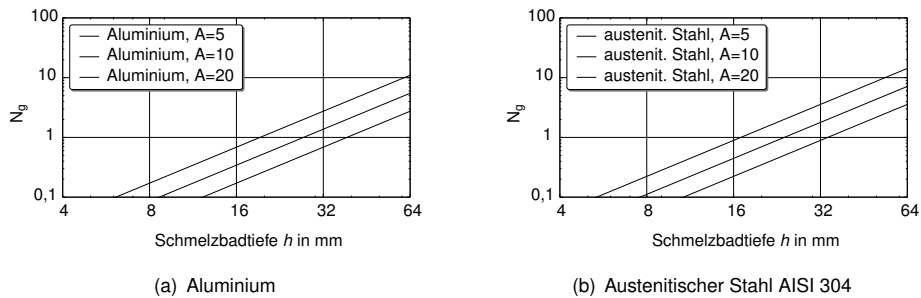
Abbildung 2.7: Das Verhältnis N_g des hydrostatischen Druckes und des Druckes durch die Oberflächenspannung für verschiedene Aspektverhältnisse der Schmelzbadtiefe zur Schmelzbadbreite A = h/2L = 5, 10, 20 in Abhängigkeit der Schmelzbadtiefe h für Aluminium und austenitischen Stahl AISI 304.
