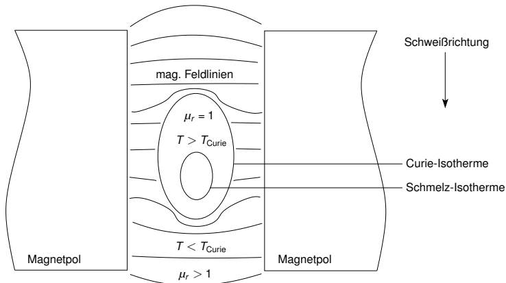
Abbildung 5.13: Magnetische und unmagnetische Bereiche beim Schweißen von Stahl.
