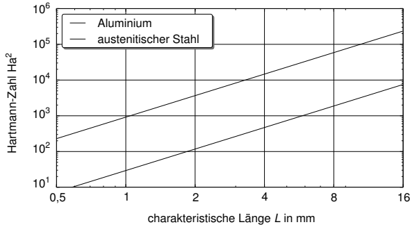
Abbildung 2.12: Hartmann-Zahl für Aluminium und austenitischen Stahl bei einer Magnetfeldstärke von B = 0,5 \text{ T} .
