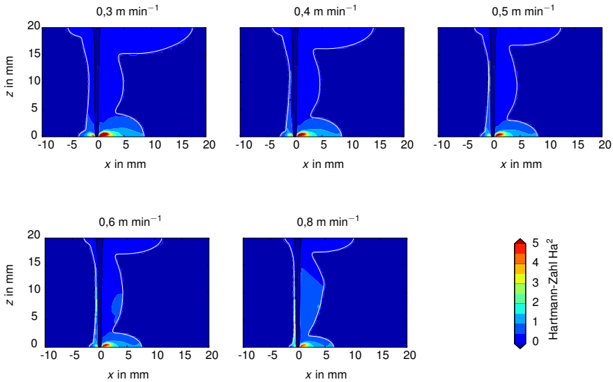
Abbildung 4.21: Hartmann-Zahl Ha^2 im Schmelzbad bei f = 3 \text{ kHz} und B = 95 \text{ mT} für eine charakteristische Länge von 5 \text{ mm} bei verschiedenen Schweißgeschwindigkeiten.
