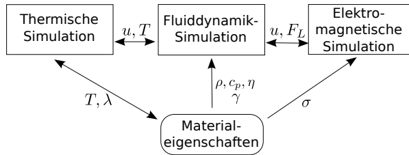
Abbildung 2.15: Kopplung der physikalischen Teilaspekte bei einer gekoppelten Thermofluidsimulation mit Berücksichtigung elektromagnetischer Feldgrößen.
