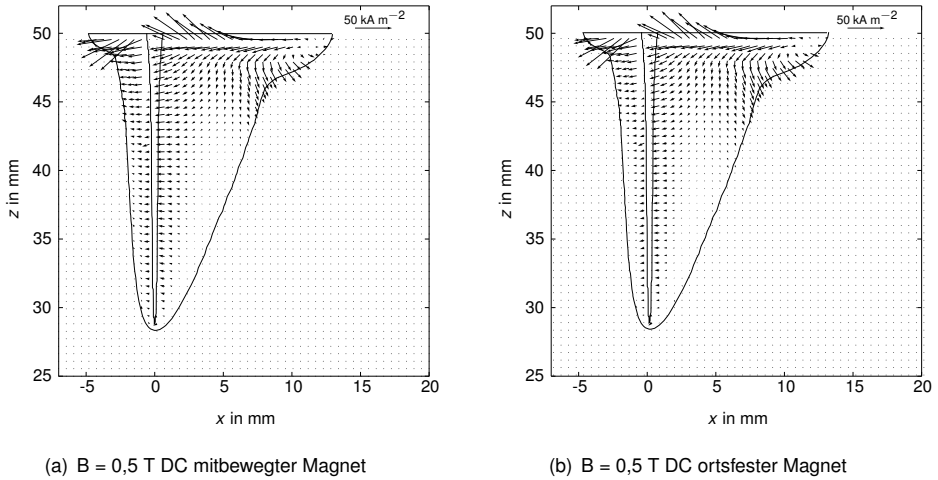
Abbildung 5.5: Qualitative Vektorfelder der elektrischen Stromdichte im Schmelzbad für mitbewegte bzw. ortsfeste Magneten.
