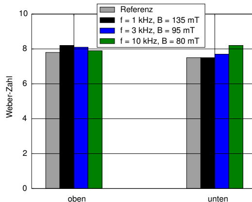
Abbildung 5.16: Vergleich der Weber-Zahlen aus den Simulationen aus Abschnitt 4.2 für die obere und untere Schmelzbadoberfläche mit und ohne elektromagnetische Unterstützung.
