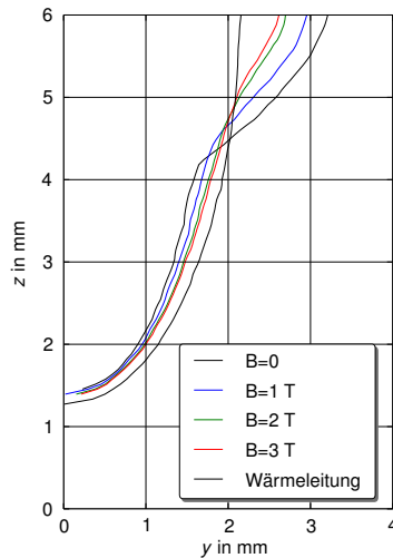
Abbildung 4.39: Querprofile aus der Computersimulation für verschiedene Magnetfeldstärken.
