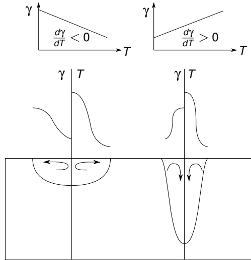
Abbildung 2.3: Schematische Marangonikonvektion im Schmelzbad nach [11, 50].
