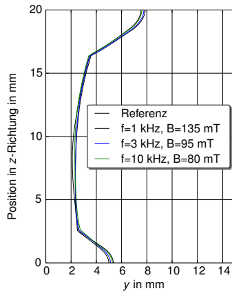
Abbildung 4.20: Querprofile aus der Simulation für optimale Druckkompensation bei unterschiedlichen Oszillationsfrequenzen an 20 mm dickem AISI 304 bei u_{\text{weld}} = 0,3\text{ m/min} . Dargestellt ist der jeweilige Verlauf der Schmelzisoothermen bei T = 1700\text{ K} in der Mitte des Erstarrungsintervalls.
