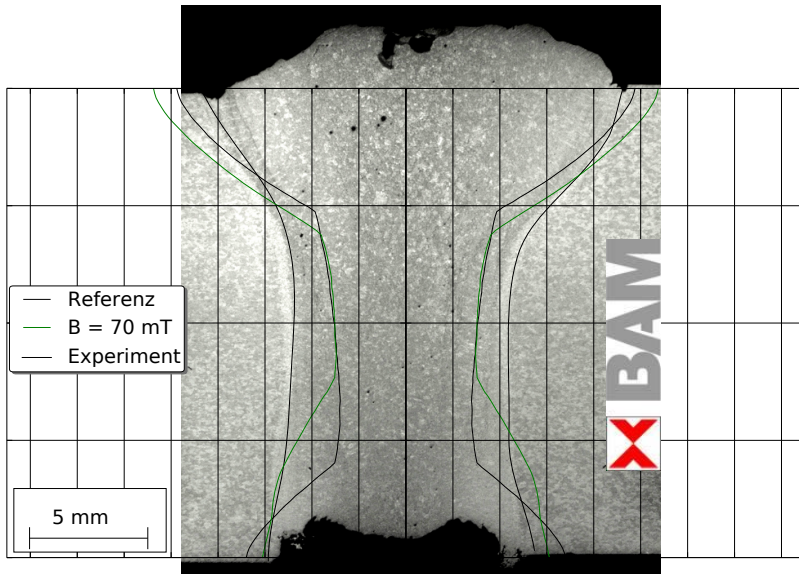
Abbildung 5.8: Vergleich von Querschliffen aus dem Experiment ( P_{\text{Laser}} = 15 \text{ kW} , u_{\text{weld}} = 0,5 \text{ m/min} , B = 77 \text{ mT} ) mit Ergebnissen aus der Simulation (Referenz ohne Magnetfeld und B = 70 \text{ mT} ).
