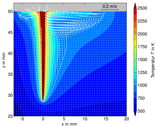
Abbildung 4.40: Temperaturverteilung und Geschwindigkeitsvektoren in der Symmetrieebene für den Referenzfall ohne elektromagnetische Felder.
