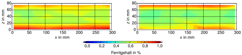
Abbildung 4.23: Ferritgehalt auf beiden Oberflächen einer 10 mm dicken Platte des Werkstoffs AISI 304.
