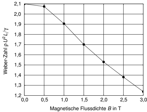
Abbildung 4.35: Weber-Zahl an der Schmelzbadoberfläche an einer Position einen Millimeter hinter der Dampfkapillare für eine Schmelzbadhalbbreite von 3,2 mm.
