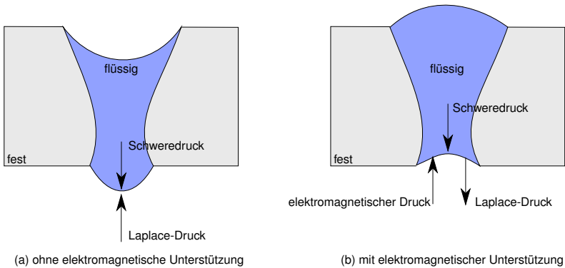
Abbildung 5.14: Laplace-Druck an der unteren Schmelzbadoberfläche abhängig von ihrer Krümmung. Gezeigt ist hier ein schematischer Querschnitt des Schmelzbades.
