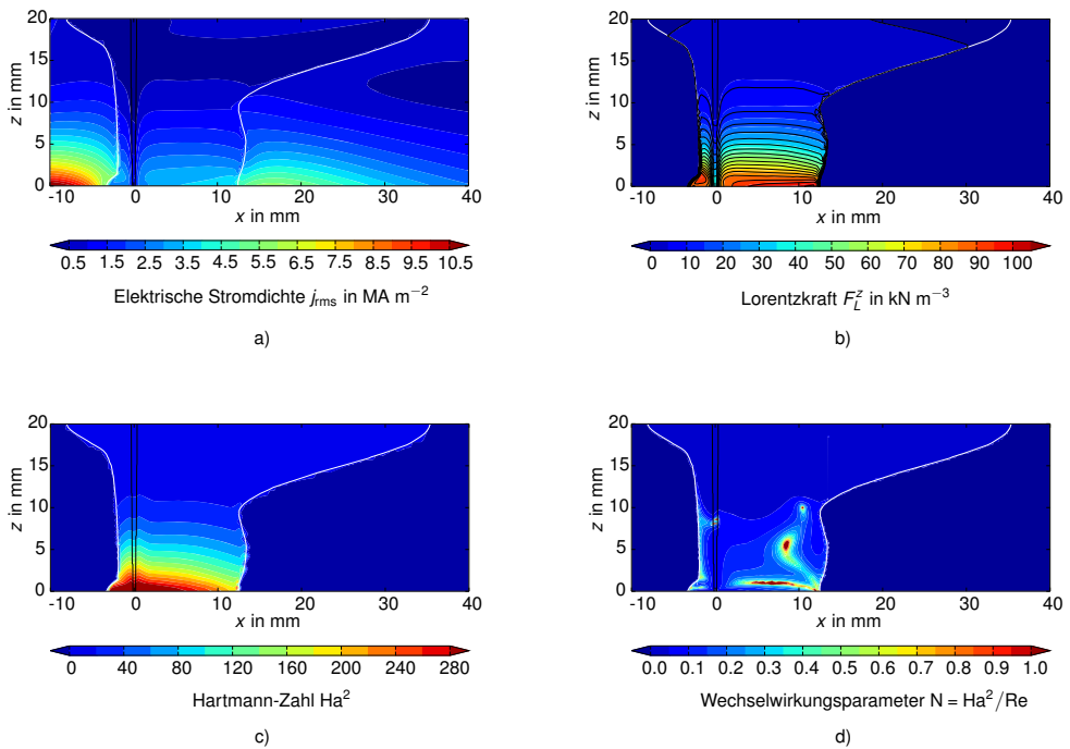
Abbildung 4.9: (a) Verteilung der elektrischen Stromdichte im Schmelzbad und zugehörige Isolinien. (b) Verteilung der vertikalen Komponente der Lorentzkraft im Schmelzbad. (c) Verteilung der Hartmann-Zahl im Schmelzbad basierend auf einer Halbbreite des Schmelzbades von 5 mm. (d) Verteilung des Wechselwirkungsparameters im Schmelzbad basierend auf einer Halbbreite des Schmelzbades von 5 mm.
