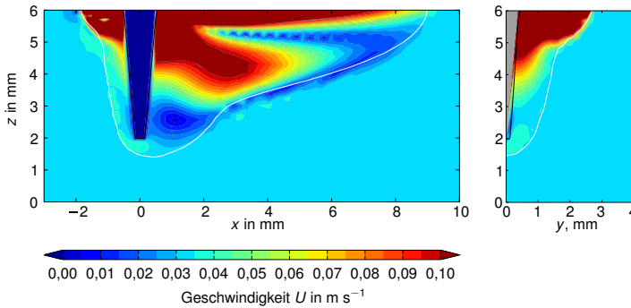
Abbildung 4.30: Geschwindigkeitsvektoren in der Symmetrieebene und quer zur Schweißrichtung durch den Dampfkanal für den Referenzfall ohne elektromagnetische Felder. Zur besseren Übersichtlichkeit sind Geschwindigkeitsbeträge über 0,1 m/s rot dargestellt.
