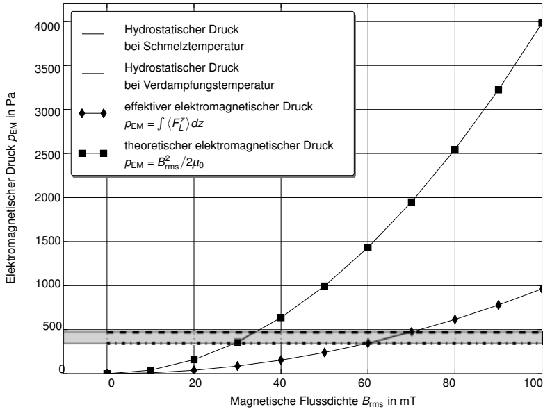
Abbildung 4.3: Ausbildung des magnetischen Druckes für verschiedene magnetische Flussdichten. Dargestellt sind der theoretische Maximalwert und der tatsächlich erreichte Wert des magnetischen Druckes aus der Simulation.
