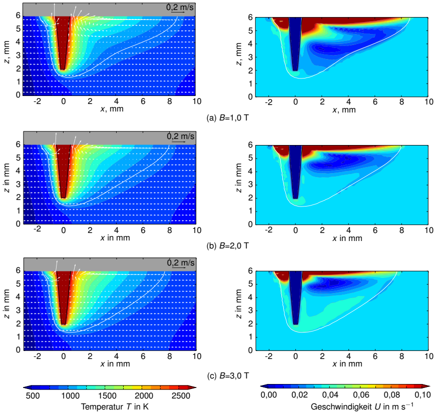
Abbildung 4.32: Temperatur- und Geschwindigkeitsverteilungen in der Symmetrieebene für verschiedene Stärken des magnetischen Feldes.
