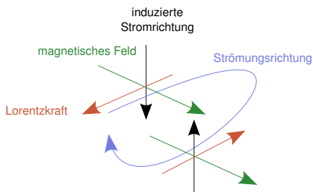
Abbildung 5.17: Schematischer Mechanismus der Wirkung des Hartmann-Effektes an einem Marangoni-Wirbel im Schmelzbad.
