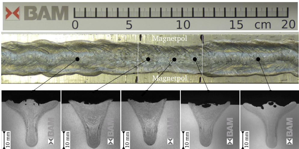
Abbildung 4.55: Nahtoberseite sowie ausgewählte Querschliffe an einer Schweißung mit montierten Permanentmagneten.
