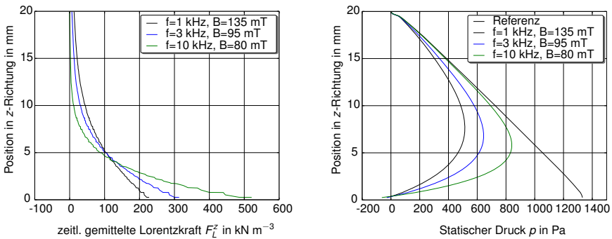
Abbildung 4.19: Zeitlich gemittelte vertikale Komponente der Lorentzkraft im Schmelzbad 3 mm hinter der Dampfkapillare in der Symmetrieebene bei einer Schweißgeschwindigkeit von 0,3 m/min an 20 mm dickem AISI 304.
