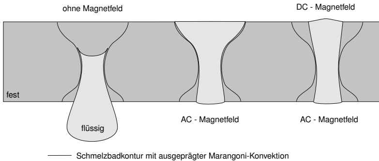
Abbildung 6.1: Querprofile von Schweißungen ohne, mit, sowie kombinierter Anwendung oszillierender und statischer elektromagnetischer Felder zur Verhinderung des Schmelzaustropfens und der Beruhigung der Schmelzbadynamik.
