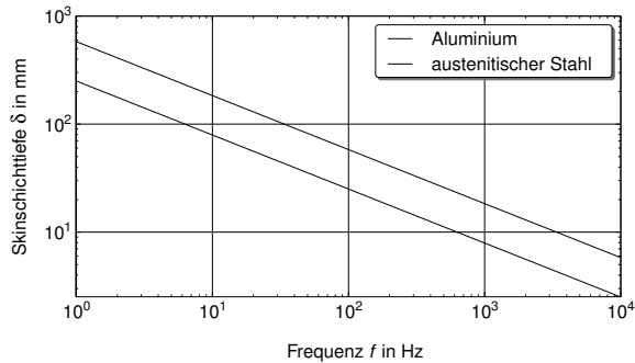
Abbildung 2.9: Die Eindringtiefe eines oszillierenden Magnetfeldes (Skin-Effekt) für flüssiges Aluminium und austenitischen Stahl AISI 304 als Funktion der Oszillationsfrequenz gemäß Gl. (2.14).
