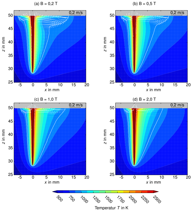
Abbildung 4.43: Temperaturverteilung und Geschwindigkeitsvektoren für verschiedene Stärken des Magnetfeldes in der Symmetrieebene.
