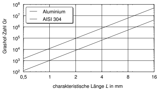
Abbildung 2.5: Grashof-Zahl für die Flüssigmetallströmung im Schmelzbad für Aluminium und austenitischen Stahl AISI 304 in flüssigem Zustand aus Gl. (2.9) abgeleitet. Materialkennwerte siehe Abschnitt 3.1.1.
