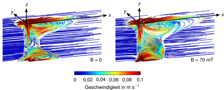
Abbildung 4.8: Stromlinienbild des Referenzfalls sowie der optimalen Kompensation B = 70 \text{ mT} . Geschwindigkeiten oberhalb von 0,1 \text{ m/s} sind zur besseren Übersichtlichkeit rot dargestellt.
