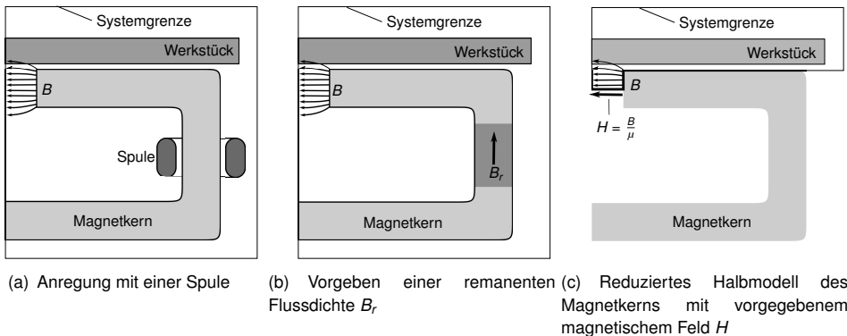
Abbildung 3.6: Verschiedene Möglichkeiten der numerischen Modellierung des magnetischen Feldes bei einer vorgegebenen Geometrie des Magneten bzw. seines Polschuhs, hier dargestellt in einer Ebene senkrecht zur Schweißrichtung im Zentrum des Magnetsystems.
