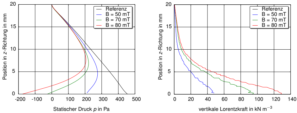
Abbildung 4.6: links: vertikaler Druckverlauf im Schmelzbad 3 mm hinter dem Dampfkanal in der Symmetrieebene, rechts: Verteilung der Lorentzkraft im Schmelzbad 3 mm hinter dem Dampfkanal in der Symmetrieebene.
