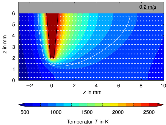
Abbildung 4.38: Temperaturverteilung und Geschwindigkeitsvektoren in der Symmetrieebene für den Fall konstanter Strömungsgeschwindigkeit im gesamten Berechnungsgebiet.
