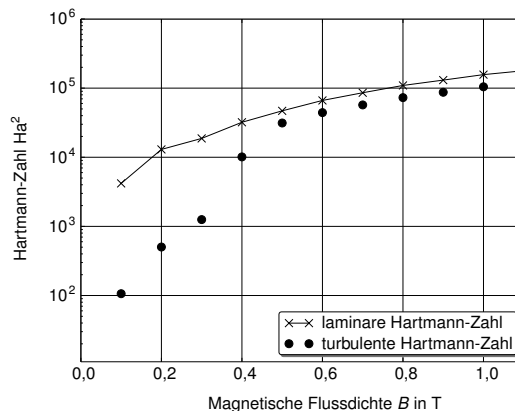
Abbildung 5.19: Lokale Hartmann-Zahl 5 mm hinter dem Dampfkapillarzentrum und 5 mm unter der Schmelzbadoberfläche für verschiedene Magnetfeldstärken.
