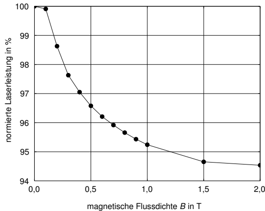
Abbildung 4.50: In das Schmelzbad eingebrachte normierte Leistung bei verschiedenen Stärken des Magnetfeldes.
