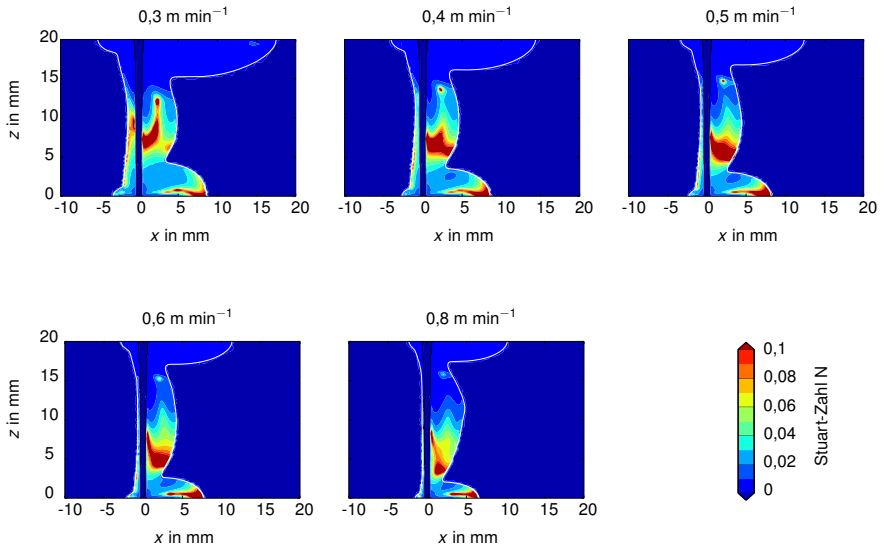
Abbildung 4.22: Interaktionsparameter N im Schmelzbad bei f = 3 \text{ kHz} und B = 95 \text{ mT} für eine charakteristische Länge von 5 \text{ mm} bei verschiedenen Schweißgeschwindigkeiten.
