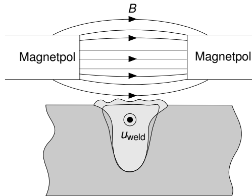
Abbildung 2.13: Einfluss des Hartmann-Effekts beim Laserstrahlschweißen dicker Aluminiumbleche. Die durchgezogene Schmelzbadkontur entspricht dem Fall ohne Nutzung von Lorentzkraften. Die gestrichelte Linie zeigt eine Schmelzisotheime unter magnetischer Beeinflussung unter Ausnutzung des Hartmann-Effekts
