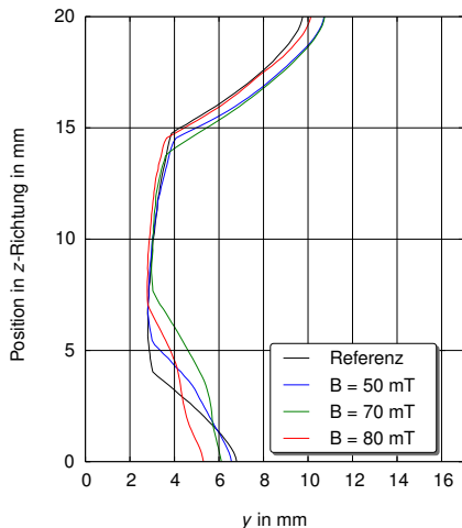
Abbildung 4.7: Querprofile aus der Simulation mit verschiedenen Magnetfeldstärken.
