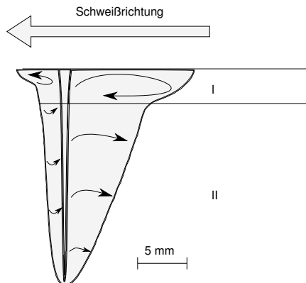
Abbildung 5.3: Schematische Ansicht der Hauptströmungsrichtungen in der Symmetrieebene des Schmelzbades von Aluminiumschweißungen beim Einschweißen unter Einwirkung eines permanentmagnetischen Feldes B_{DC} = 500 \text{ mT} .
