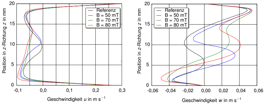
Abbildung 4.5: Geschwindigkeitsverteilungen der u - und w -Komponente der Geschwindigkeit 3 mm hinter der Dampfkapillare.
