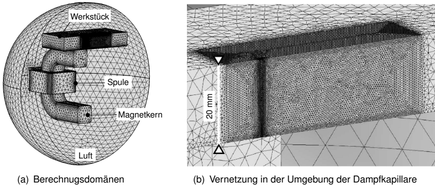
Abbildung 3.4: Beispielhaftes Berechnungsgitter, welches für die Simulationen stationär ist.
