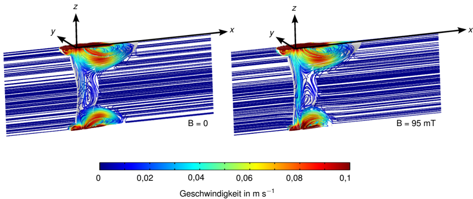
Abbildung 4.17: Stromlinienbild des Referenzfalls sowie der optimalen Kompensation bei f = 3 \text{ kHz} und B = 95 \text{ mT} . Geschwindigkeiten oberhalb von 0,1 \text{ m/s} sind zur besseren Übersichtlichkeit rot dargestellt.
