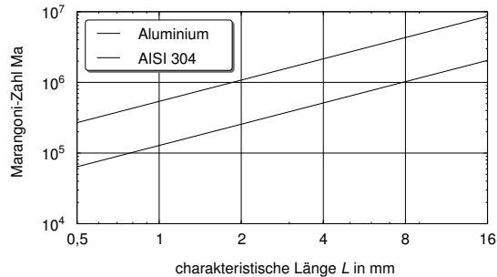
Abbildung 2.4: Marangoni-Zahl für die Flüssigmetallströmung im Schmelzbad für Aluminium und austenitischen Stahl AISI 304 in flüssigem Zustand aus Gl. (2.6) abgeleitet. Materialkennwerte siehe Abschnitt 3.1.1.
