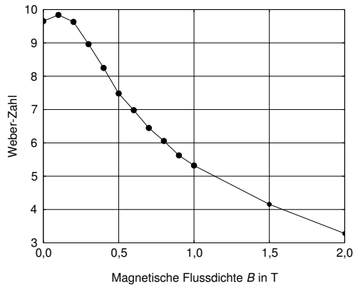
Abbildung 4.47: Lokale Weber-Zahl 3 mm hinter dem Dampfkapillarzentrum im Punkt des größten Geschwindigkeitsbetrages an der Schmelzbadoberfläche für verschiedene Magnetfeldstärken.
