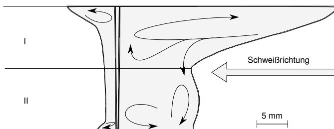
Abbildung 5.2: Schematische Ansicht der Hauptströmungsrichtungen in der Symmetrieebene des Schmelzbades von Aluminiumschweißungen beim Durchschweißen unter elektromagnetischer Beeinflussung mittels oszillierender Magnetfelder B_{AC}^{rms} = 70 \text{ mT} .
