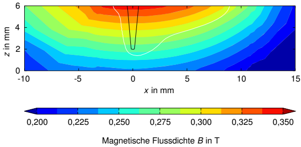
Abbildung 4.31: Simulierte Verteilung der magnetischen Flussdichte in der Symmetrieebene für den Fall B = 500 \text{ mT} .
