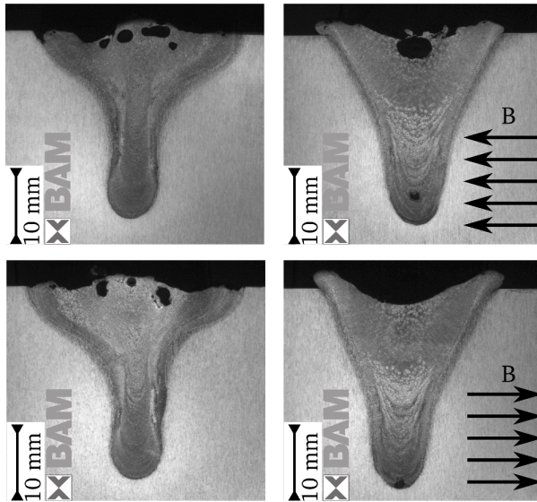
Abbildung 4.56: Querschliffe an Schweißungen mit gedrehter Polarisierung des magnetischen Feldes (links: Referenzfall, rechts: magnetisch beeinflusste Schweißung).
