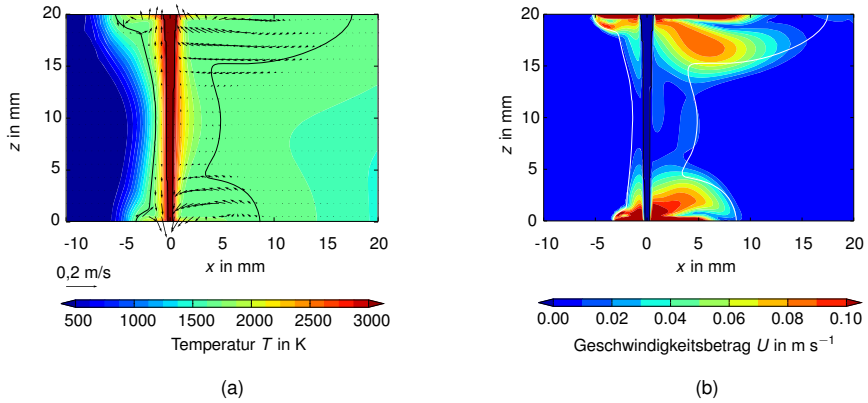
Abbildung 4.16: Simulation der optimalen Kompensation des hydrostatischen Druckes mit einer magnetischen Flussdichte von B = 95 \text{ mT} an 20 mm dickem AISI 304, Schweißgeschwindigkeit u_{\text{weld}} = 0,3 \text{ m/min} . (a) Temperatur- und Geschwindigkeitsverteilung sowie Schmelzisotherme in der Symmetrieebene, (b) Geschwindigkeitsbetrag.
