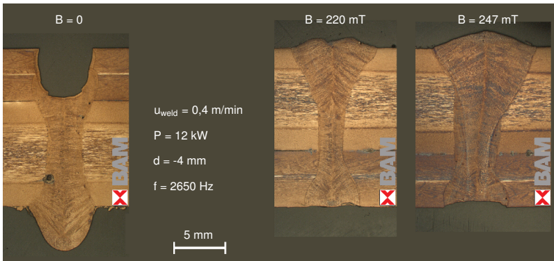
Abbildung 4.26: Experimentelle Ergebnisse zur elektromagnetischen Kompensation des hydrostatischen Druckes in einem 15 mm tiefen Schmelzbad des Werkstoffs AISI 304.
