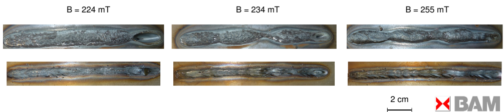
Abbildung 4.27: Experimentelle Ergebnisse zur elektromagnetischen Kompensation des hydrostatischen Druckes in einem 20 mm tiefen Schmelzbad bestehend aus den Werkstoffen S235JRC (Oberseite) und AISI 304 (Unterseite).
