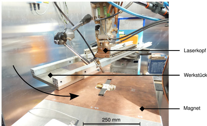
Abbildung 3.10: Experimenteller Aufbau mit AC-Magnet unterhalb des Werkstücks.
