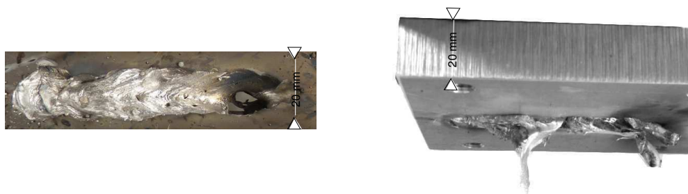
Abbildung 4.11: Fotografie eines geschweißten 20 mm dicken Werkstücks aus AlMg3 mit nicht-optimaler elektromagnetischer Unterstützung bei einer magnetischen Flussdichte von 65 mT (links: Draufsicht, rechts: Seitenansicht).
