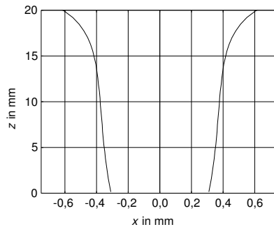
Abbildung 3.7: Skaliertes rotationssymmetrisches Modell der Dampfkapillare von AISI 304 für die Simulation aus der FE-Software BeamSIM [175] für Abschnitt 4.2.
