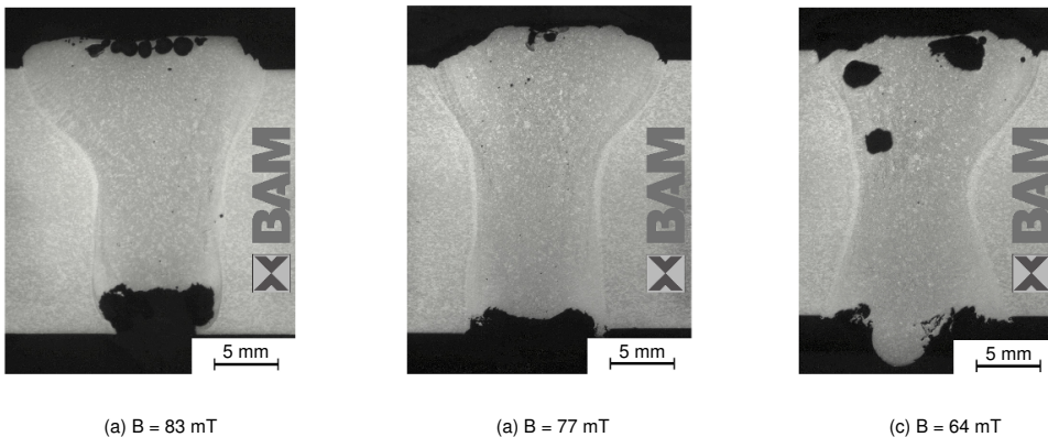
Abbildung 4.10: Querschliffe an 20 mm dicken AlMg3-Platten mit elektromagnetischer Schmelzbadunterstützung durch oszillierende Magnetfelder.
