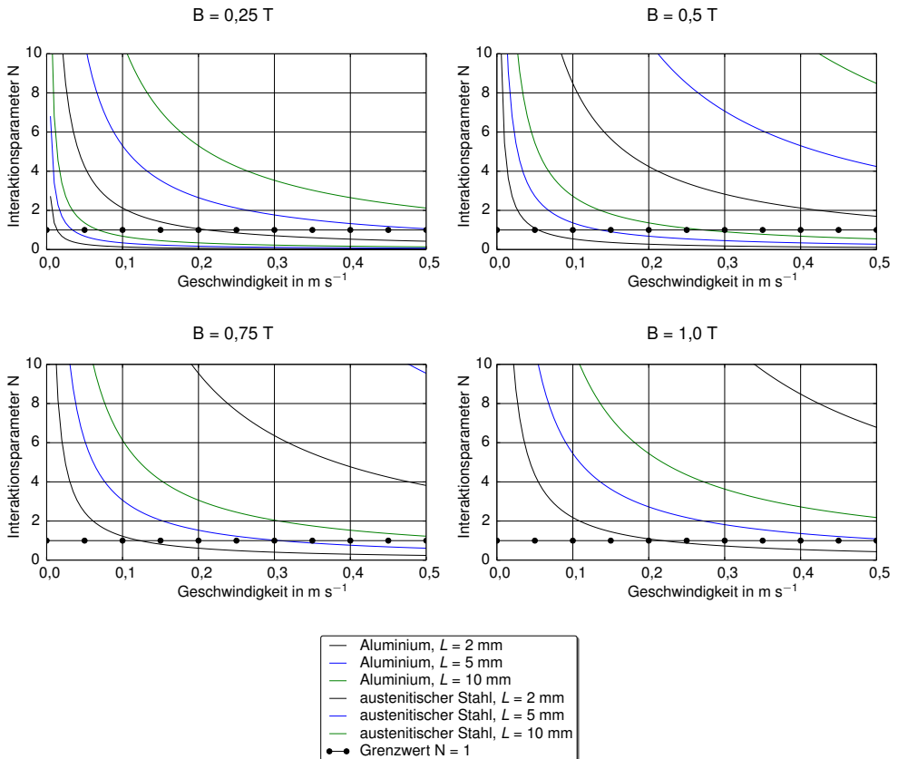
Abbildung 5.21: Interaktionsparameter N für Aluminium und austenitischen Stahl AISI 304 für verschiedene magnetische Flussdichten abhängig von der lokalen Strömungsgeschwindigkeit in Anlehnung an [50].
