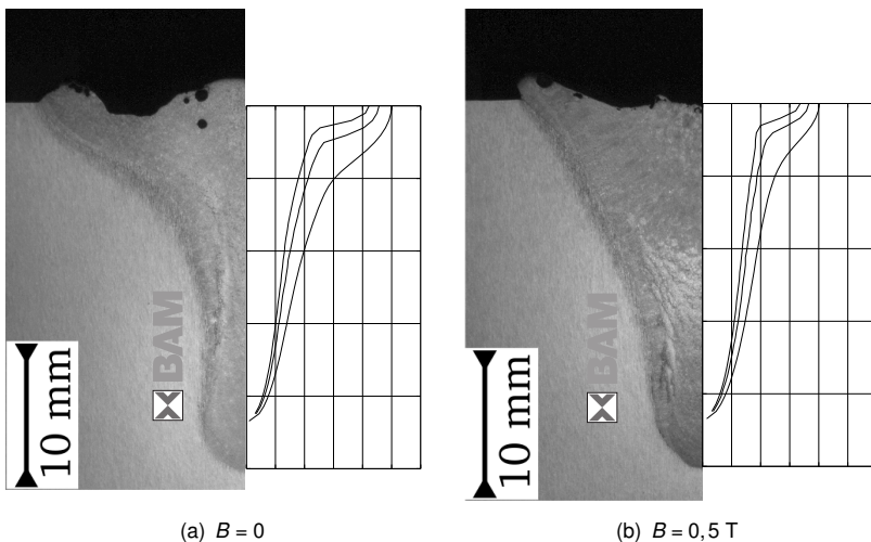
Abbildung 5.18: Vergleich der Querprofile des Schmelzbades ohne und mit elektromagnetischer Beeinflussung. Die durchgezogene Linie repräsentiert die Schmelzisotheorie, die gestrichelten Linien das numerische Erstarrungsintervall.
