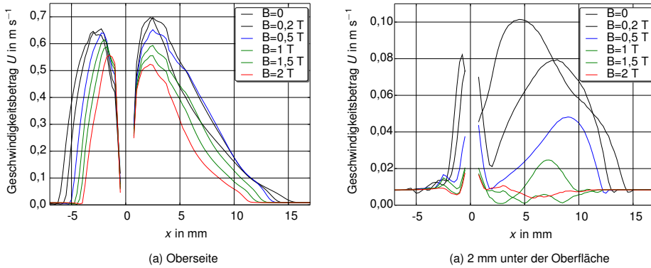
Abbildung 4.46: (a) Geschwindigkeitsbeträge entlang der Schweißrichtung an der Oberfläche. (b) Geschwindigkeitsbeträge entlang der Schweißrichtung 2 mm unter der Oberfläche.
