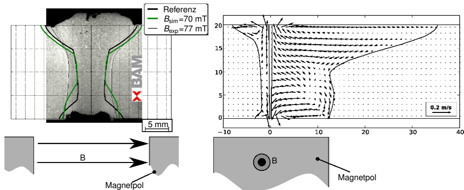
Abbildung 5.11: Quer- und Längsprofil der erzeugten Schweißnaht in Relation zu den Abmaßen der Magnetpole.
