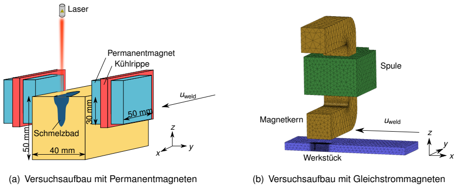
Abbildung 3.12: Versuchsaufbau zum Hartmann-Effekt.
