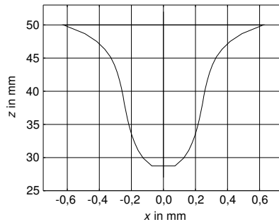
Abbildung 3.8: Skaliertes rotationssymmetrisches Modell der Dampfkapillare von Aluminium für die Simulation aus der FE-Software BeamSIM [175] für Abschnitt 4.4.
