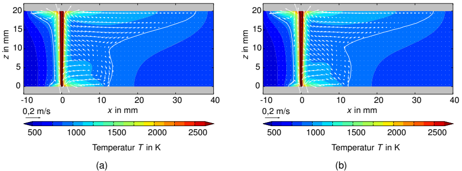
Abbildung 5.10: Temperatur- und Geschwindigkeitsverteilungen im Schmelzbad für die Simulation des Schweißprozesses von 20 mm Aluminium im Falle der Anwendung elektromagnetischer Felder mit B = 70 \text{ mT} . (a) verallgemeinertes Ohm'sches Gesetz mit Berücksichtigung geschwindigkeitsabhängiger Terme, (b) ohne Berücksichtigung geschwindigkeitsabhängiger Terme.
