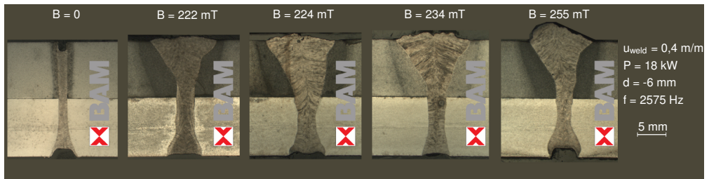
Abbildung 4.27: Experimentelle Ergebnisse zur elektromagnetischen Kompensation des hydrostatischen Druckes in einem 20 mm tiefen Schmelzbad bestehend aus den Werkstoffen S235JRC (Oberseite) und AISI 304 (Unterseite).
