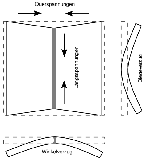
Abbildung 2.11: Dreidimensionaler Verzug eines geschweißten Bauteils nach [98].
