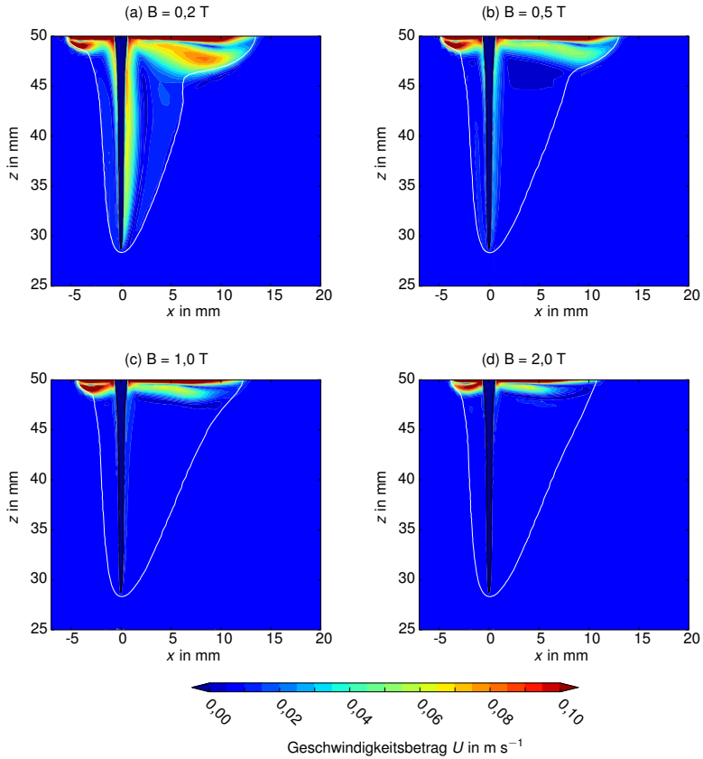
Abbildung 4.44: Geschwindigkeitsverteilung für verschiedene Stärken des Magnetfeldes in der Symmetrieebene.
