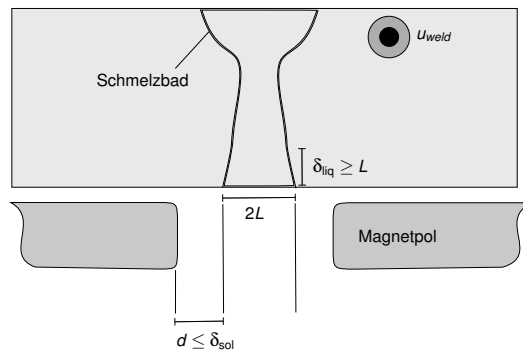
Abbildung 5.7: Maße für die Wahl einer geeigneten Oszillationsfrequenz für das Magnetfeld.
