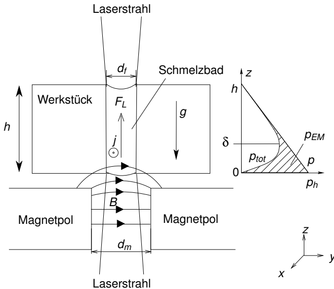
Abbildung 2.10: Prinzipielles Schema der kontaktlosen induktiven AC-Magnetfeldunterstützung des Schmelzbades beim Einlagen-Laserstrahlschweißen von dicken Platten nach [63]. Der AC-Magnet befindet sich unter dem Werkstück. Der Laserstrahl ist oberhalb des Werkstücks positioniert (PA-Position), kann aber ggf. auch unterhalb (Überkopf-Position) der Platte angebracht werden, wobei der Laserstrahl dann mittig durch den Spalt zwischen den Magnetpolen geführt wird.
