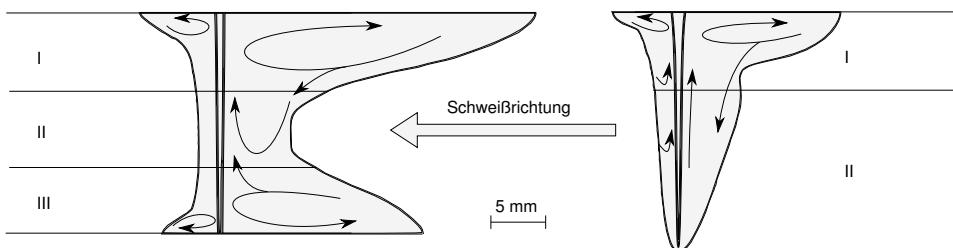
Abbildung 5.1: Schematische Ansicht der Hauptströmungsrichtungen in der Symmetrieebene des Schmelzades von Aluminiumschweißungen. Links: Durchschweißen, rechts: Einschweißen.
