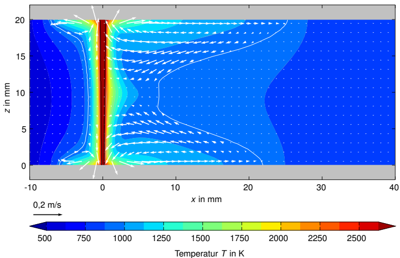
Abbildung 4.2: Temperatur- und Geschwindigkeitsverteilungen im Schmelzbad für die Simulation des Schweißprozesses von 20 mm Aluminium ohne Anwendung elektromagnetischer Felder sowie ohne freie Konvektion.
