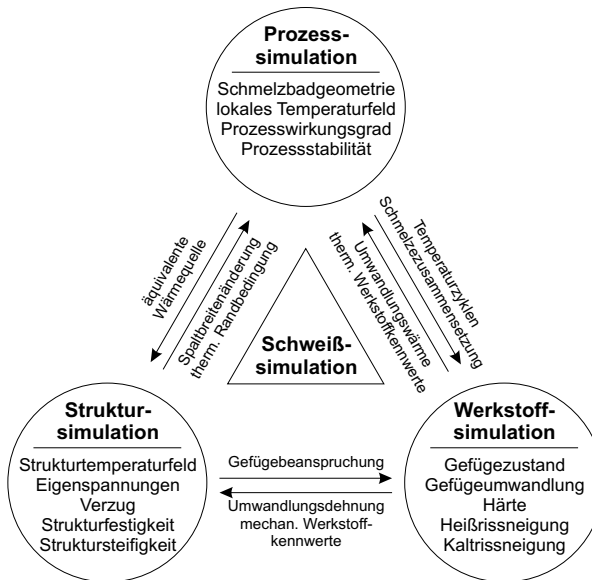
Abbildung 2.14: Verschiedene Aspekte der Schweißsimulation in Anlehnung an [122], entnommen aus [123].
