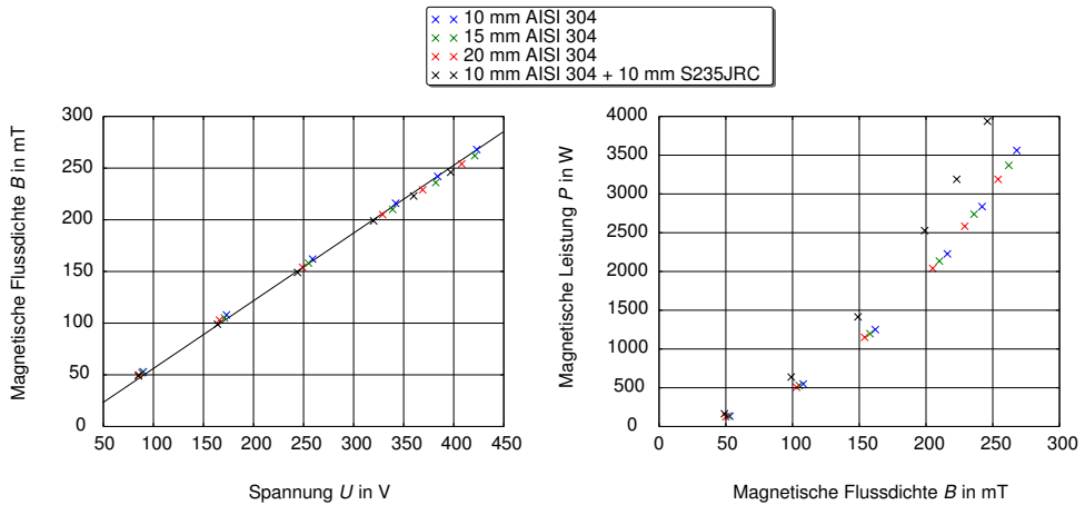
Abbildung 3.11: Kalte Messungen am AC-Magnet für verschiedene Stahlsorten. Die ermittelte Wirkleistung des Magneten stützt sich auf die im Schwingkreis gemessenen Werte von Strom und Spannung.
