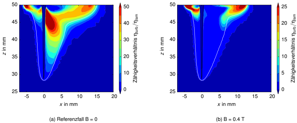
Abbildung 5.20: Verhältnis von turbulenter zu molekularer Viskosität im Schmelzbad.
