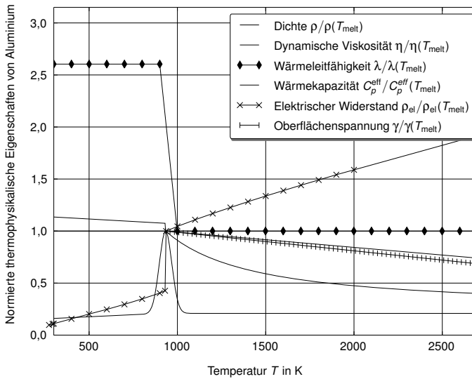
Abbildung 3.1: Normierte thermophysikalische Eigenschaften von reinem Aluminium [159–161].
