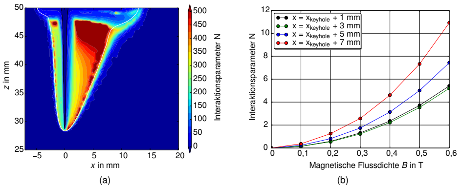
Abbildung 4.49: Interaktionsparameter N (a) im Schmelzbad bei B = 0,5 \text{ T} und (b) an verschiedenen Punkten an der Schmelzbadoberfläche hinter der Dampfkapillare für ansteigende magnetische Flussdichte.
