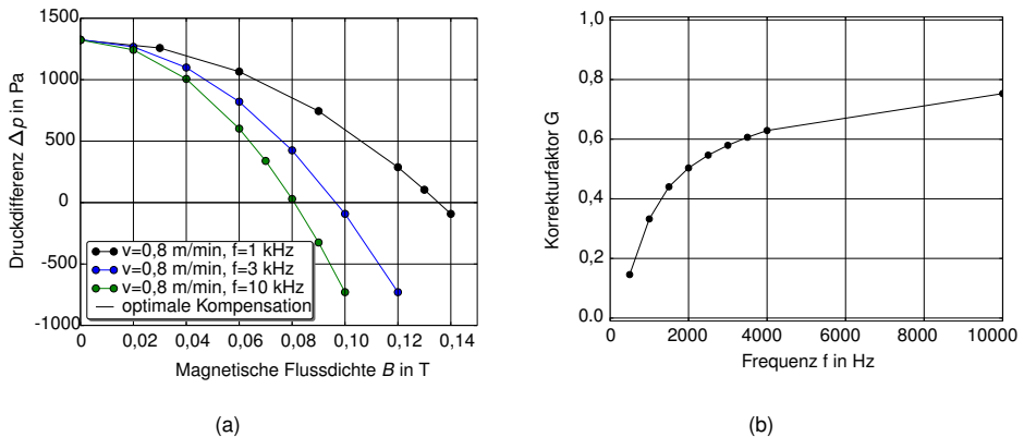
Abbildung 4.14: (a) Kompensation des hydrostatischen Druckes im Schmelzbad für verschiedene Oszillationsfrequenzen und Stärken der magnetischen Flussdichte bei 20 mm dickem AISI 304, Schweißgeschwindigkeit u_{\text{weld}} = 0,8 m/min, (b) Korrekturfaktor.
