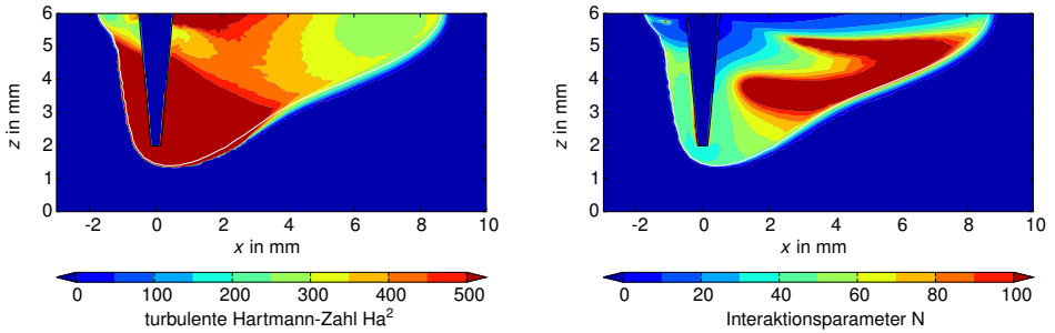
Abbildung 4.36: Turbulente Hartmann-Zahl und der zugehörige Interaktionsparameter im Schmelzbad bei einer magnetischen Flussdichte von B = 1 \text{ T} .
