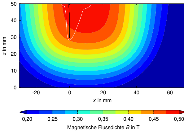
Abbildung 4.42: Simulierte Verteilung der magnetischen Flussdichte in der Symmetrieebene für den Fall B = 500 \text{ mT} .
