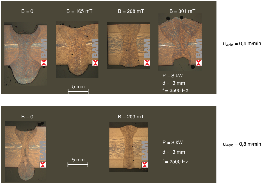
Abbildung 4.24: Experimentelle Ergebnisse zur elektromagnetischen Kompensation des hydrostatischen Druckes in einem 10 mm tiefen Schmelzbad des Werkstoffs AISI 304.
