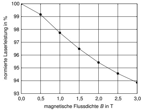
Abbildung 4.37: In das Schmelzbad eingebrachte normierte Laserleistung.
