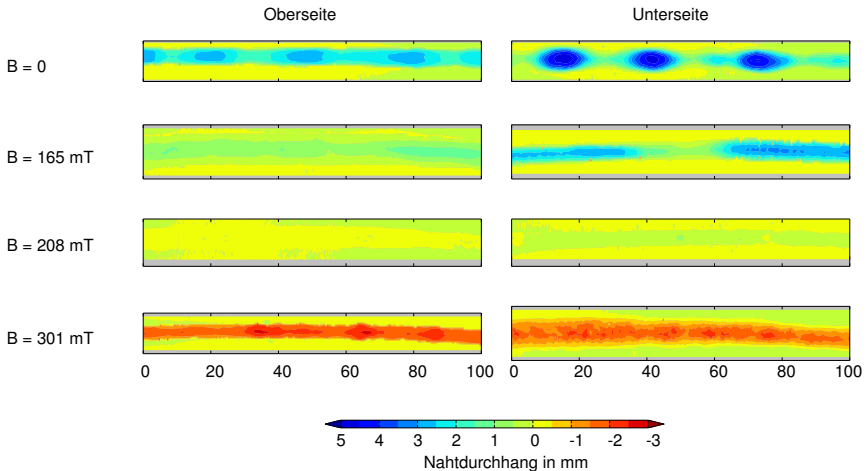
Abbildung 4.25: Oberflächenvermessung an 10 mm dicken Proben AISI 304 für verschiedene magnetische Flussdichten bei einer Frequenz von 2,5 kHz und einer Schweißgeschwindigkeit von 0,4 m/min.
