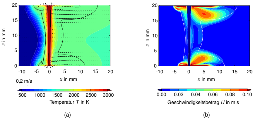
Abbildung 4.13: Referenzsimulation ohne magnetische Unterstützung an 20 mm dickem AISI 304, Schweißgeschwindigkeit u_{\text{weld}} = 0,3 \text{ m/min} . (a) Temperatur- und Geschwindigkeitsverteilung sowie Schmelzisotherme in der Symmetrieebene, (b) Geschwindigkeitsbetrag.
