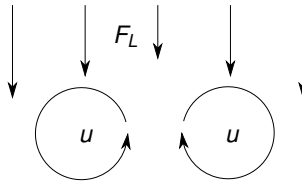
Abbildung 5.12: Entstehung rotatorischer Geschwindigkeitskomponenten durch inhomogene Lorentzkraftverteilungen.
