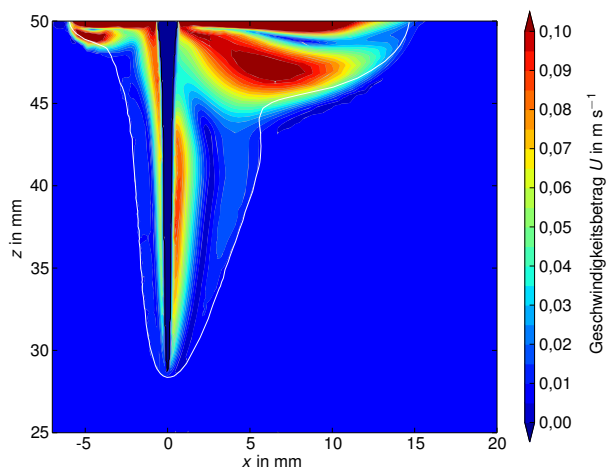
Abbildung 4.41: Geschwindigkeitsverteilung in der Symmetrieebene für den Referenzfall ohne elektromagnetische Felder.
