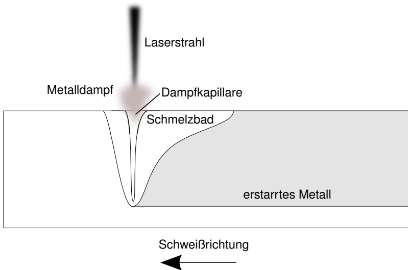
Abbildung 2.1: Laserstrahlschweißen nach [8].
