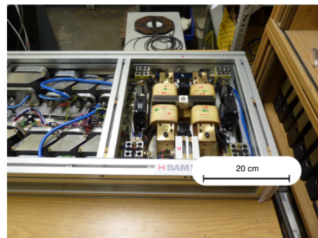
Abbildung 3.9: Schema und Foto des AC-Magneten zur Erzeugung oszillierender Magnetfelder.
