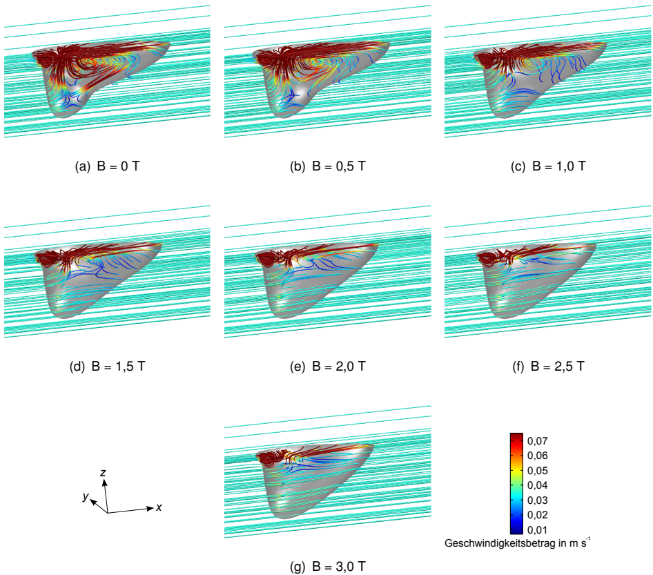
Abbildung 4.34: Stromlinien der Geschwindigkeit für verschiedene Stärken des magnetischen Feldes.
