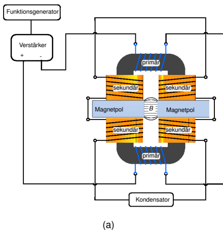
Abbildung 3.9: Schema und Foto des AC-Magneten zur Erzeugung oszillierender Magnetfelder.
