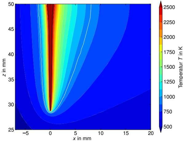
Abbildung 4.51: Berechnung des Temperaturfeldes unter Berücksichtigung eines konstant konvektiven Terms durch die Vorschubgeschwindigkeit.
