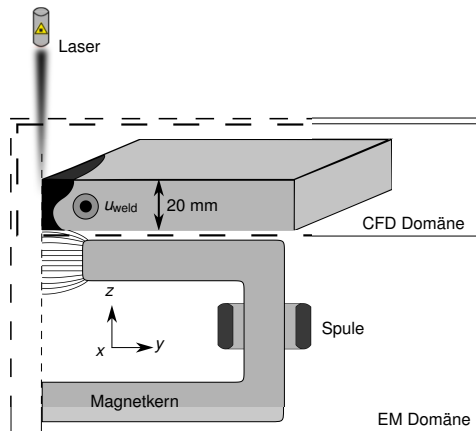
Abbildung 3.3: Simulationsanordnung.
