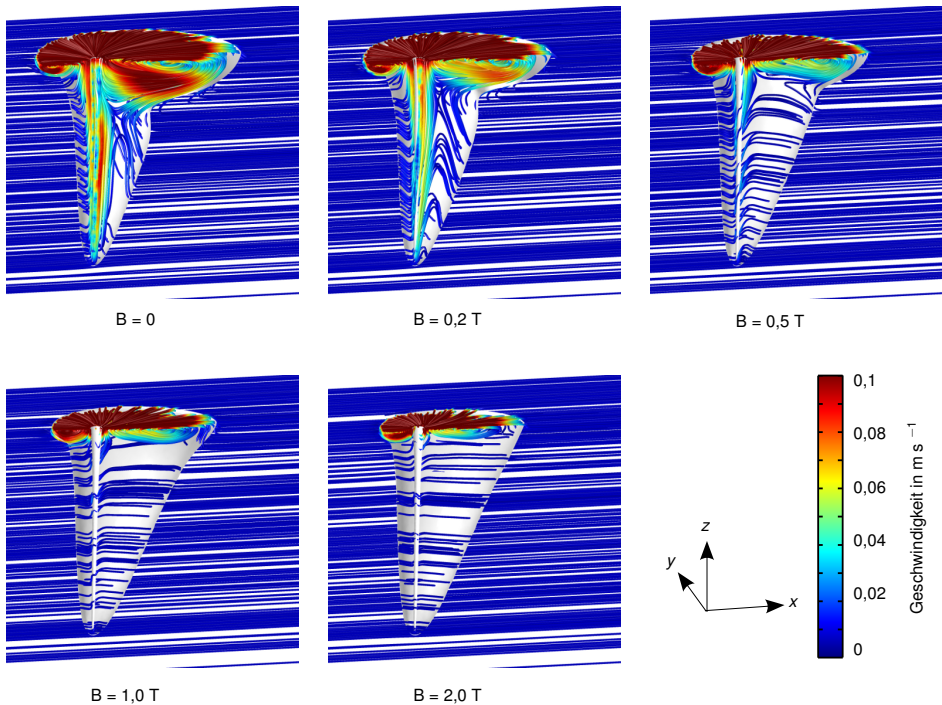
Abbildung 4.45: Geschwindigkeitsstromlinien im Schmelzbad bei verschiedenen Stärken des Magnetfeldes. Geschwindigkeiten oberhalb von 0,1 m/s sind rot dargestellt.
