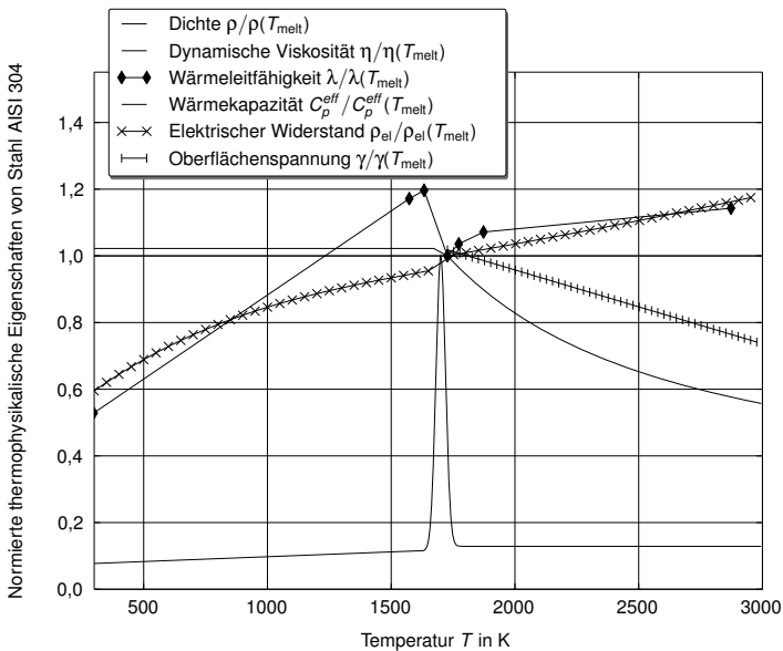
Abbildung 3.2: Normierte thermophysikalische Eigenschaften von Chrom-Nickel-Stahl AISI 304 [51, 159, 162].
