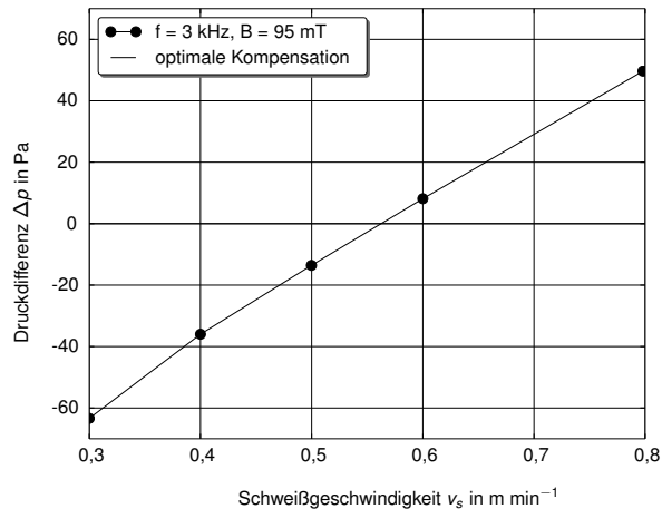
Abbildung 4.15: Abhängigkeit der Kompensation des hydrostatischen Druckes von der Schweißgeschwindigkeit bei einer Oszillationsfrequenz von 3 kHz und einer magnetischen Flussdichte von 95 mT.
