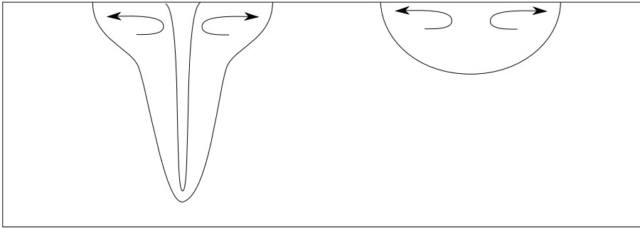
Abbildung 2.2: Schnitt quer zur Schweißrichtung angelehnt an [4]. Links: Tiefschweißen mit ausgebildeter Dampfkapillare und Marangoni-Strömung bei negativem Gradienten der Oberflächenspannung \gamma' . Rechts: Reines Wärmeleitungsschweißen.
