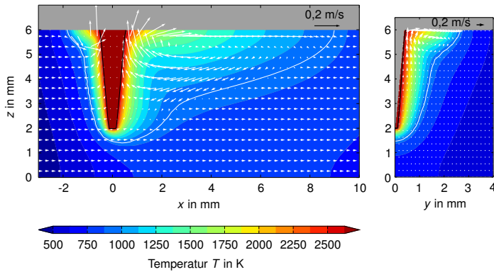
Abbildung 4.29: Temperaturverteilung und Geschwindigkeitsvektoren in der Symmetrieebene und quer zur Schweißrichtung durch den Dampfkanal für den Referenzfall ohne elektromagnetische Felder.
