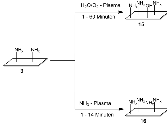
Abbildung 26: Schematische Darstellung der Erzeugung einer höheren Aminogruppendichte auf Si 3 N 4 -Oberflächen durch die Behandlung mit einem wasserbasierten Sauerstoffplasma bzw. Ammoniakplasma.
