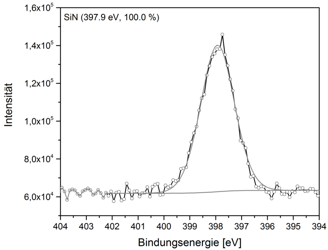
Abbildung 150: N 1s-SR-XP-Spektren einer mit Streptavidin interagierenden Si 3 N 4 -Oberfläche nach der Azidierung nach Prozess D ohne vorherige Click-Reaktion mit Biotin-PEG4-Alkin (Negativkontrolle) ( \theta=60^\circ , z_{95}=2.3 nm ( h\nu=500 eV)).
