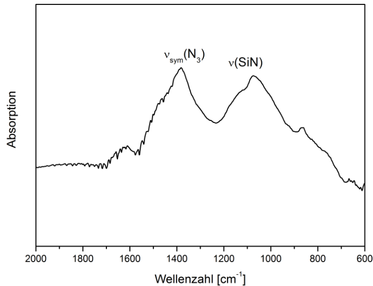
Abbildung 35: GIR-Spektrum einer mit Natirumazid in DMF/H 2 O (Prozess A) azidierten \text{Si}_3\text{N}_4 -Oberfläche.
