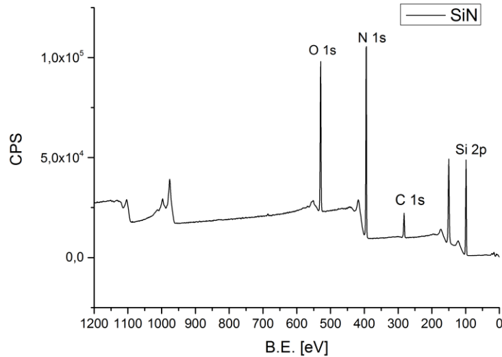
Abbildung 12: Übersichtsspektrum einer Siliziumnitrid-Oberfläche (80 nm Si 3 N 4 auf Silizium).
