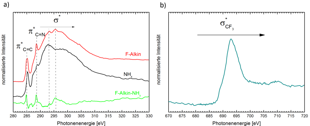
Abbildung 42: NEXAFS C K-Kante und F K-Kante einer nach Prozess C azidierten und mit 1-Ethynyl-3,5-bis(trifluormethyl)benzol in Ethanol geklickten Siliziumnitrid-Oberfläche 9 , aufgenommen bei 55°. Die C K-Kante zeigt die geklickte Probe im Vergleich zu einer gereinigten Oberfläche 3 . In der F K-Kante sind \sigma^* -Resonanzen der CF 3 -Gruppe zu sehen.
