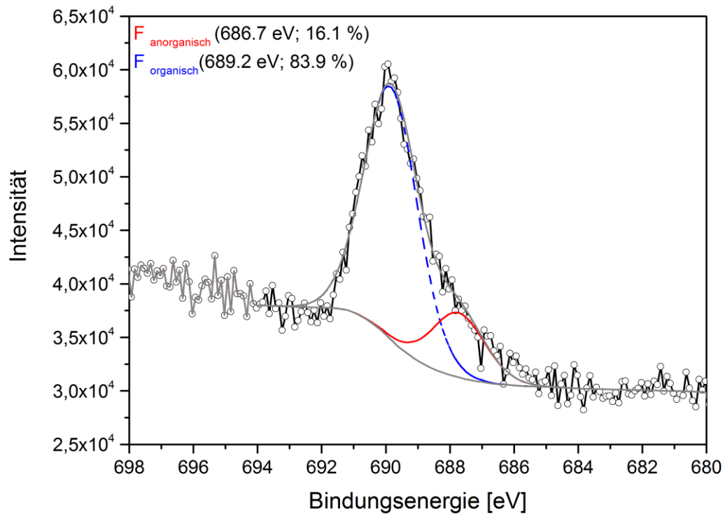
Abbildung 97: F 1s-SR-XP-Spektren einer mit \text{NaN}_3 in Anwesenheit von tert -Butylnitrit azidierten (Prozess D) und mit 1-Ethynyl-3,5-bis(trifluormethyl)benzol in tert -Butanol/Wasser geclickten \text{Si}_3\text{N}_4 -Oberflächen ( \theta=60^\circ , z_{95}=0.7 nm ( h\nu=780 eV)).
