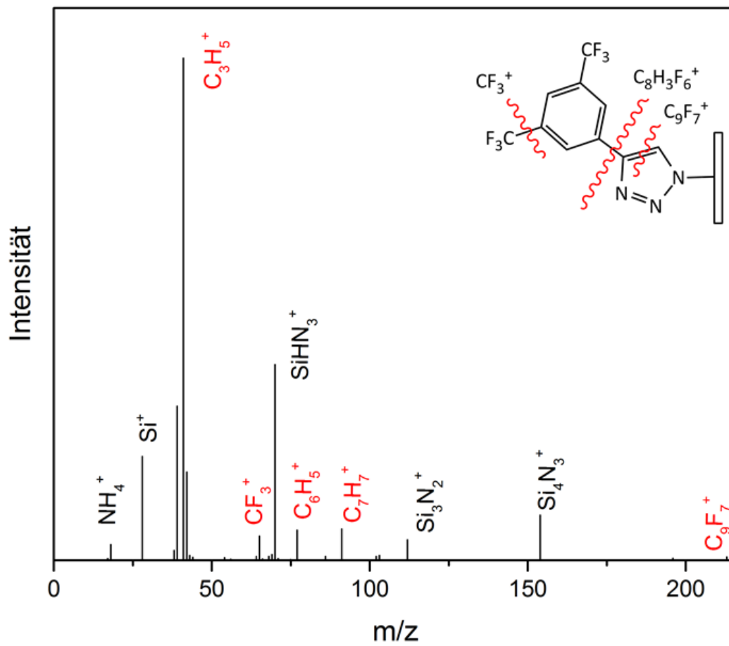
Abbildung 90: ToF-SIMS-Massenspektrum einer mit NaN_3 azidierten (Prozess A) und mit 1-Ethynyl-3,5-bis(trifluormethyl)-benzol in tert -Butanol/Wasser gelickten Si_3N_4 -Oberflächen.
