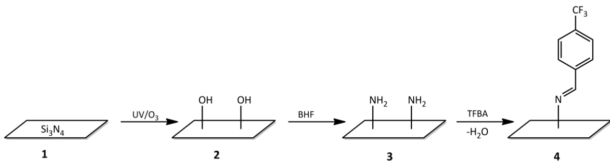
Abbildung 24: Schematische Darstellung der optimalen Reinigungsmethode der verwendeten Si 3 N 4 -Oberflächen. Nach der Reduzierung von Kohlenstoffkontaminationen mit Isopropanol und UV/O 3 folgt die Entfernung der nativen Sauerstoffschicht mit BHF. Die erzeugten Aminogruppen wurden nach der Derivatisierung mit TFBA mittels CD-XPS quantifiziert.
