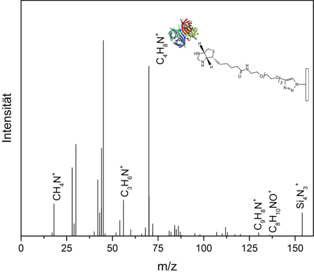
Abbildung 110: ToF-SIMS-Massenspektrum einer mit NaN_3 azidierten (Prozess A) und mit Biotin-PEG4-Alkin geklickten und mit Streptavidin interagierenden Si_3N_4 -Oberflächen.
