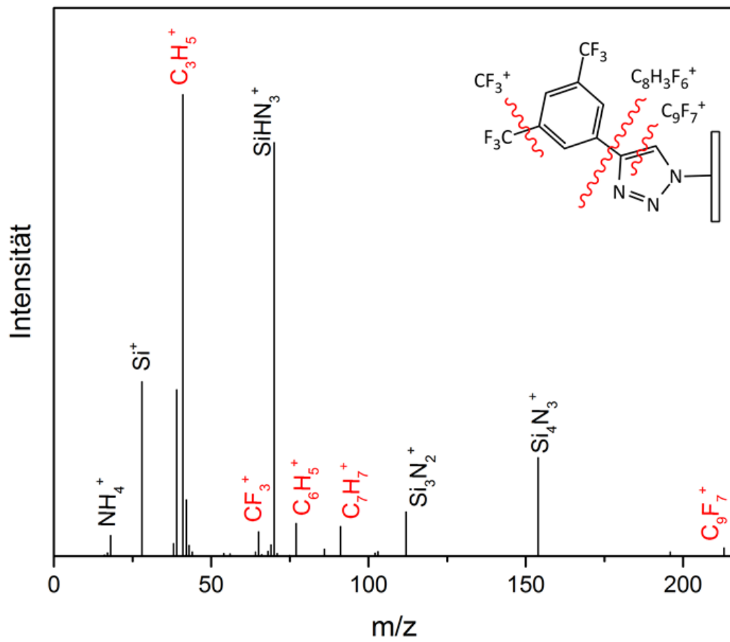
Abbildung 101: ToF-SIMS-Massenspektrum einer mit \text{NaN}_3 in Anwesenheit von tert -Butylnitrit azidierten (Prozess D) und mit 1-Ethynyl-3,5-bis(trifluormethyl)benzol in tert -Butanol/Wasser geclickten \text{Si}_3\text{N}_4 -Oberflächen.
