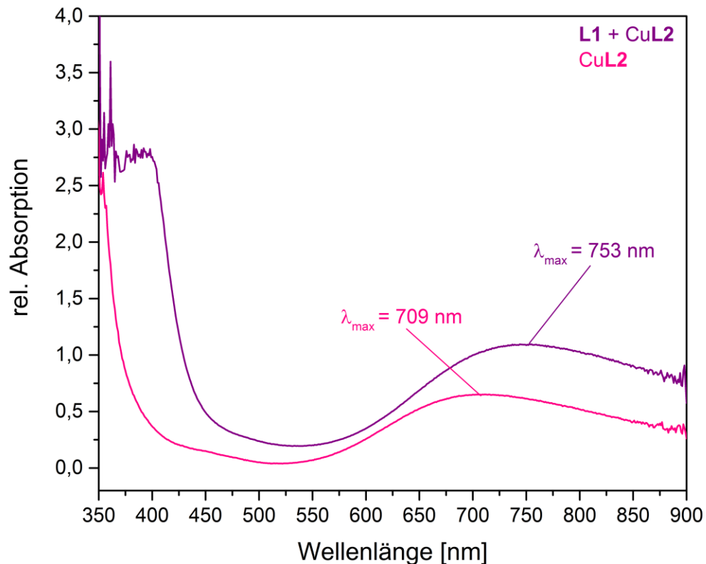
Abbildung 71: UV/Vis-Spektrum des Cu-Komplexes (CuL2) und des gebildeten 1:1-Komplexes (L1+CuL2).
