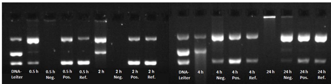
Abbildung 73: Spaltaktivität des immobilisierten Cu(II)trifluormethoxyphenanthrolin-Komplexes auf Si 3 N 4 gegenüber pBR322-Plasmid-DNA in MOPS-Puffer (50 mM) und L-Ascorbinsäure (0.32 mM) für 0.5 h, 2 h, 4 h und 24 h bei 37 °C. Gezeigt sind sowohl die Ergebnisse der Agarose-Gelelektrophorese als auch die prozentuale Zusammensetzung der geschnittenen DNA der Formen II bzw III.
