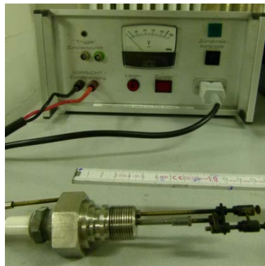
Abb. 27: Kondensatorzündgerät mit Gleitfunkenzünder
