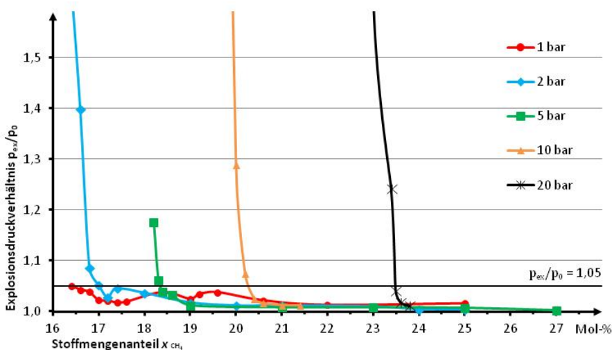
Abb. 36: Explosionsdrucksteigerung in Abhängigkeit vom Brenngasanteil an der OEG für \text{CH}_4/\text{Luft} bei p_0 = (1, 2, 5, 10, 20) bar, schwarze Gerade: Druckschwellenkriterium p_{\text{ex}}/p_0 = 1,05
