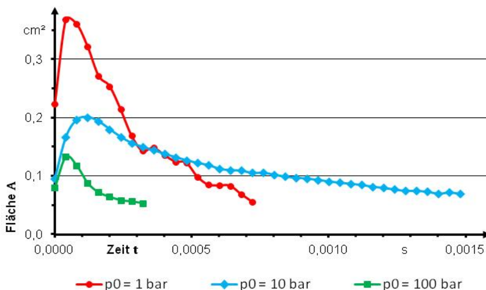
Abb. 62: Expansion des Funkens (Fläche A in \text{cm}^2 ) für Gleitfunkenzünder in Luft in Abhängigkeit vom Anfangsdruck p_0 , Messpunkte: Mittelwert aus sechs Versuchen, Aufnahmefrequenz f_a = 25.000 fps
