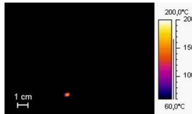
Abb. 50: Frontale Thermografieaufnahme ( f_a = 850 fps bei 160 \times 120 Bildpunkten) Hochspannungsfunkenzündung
