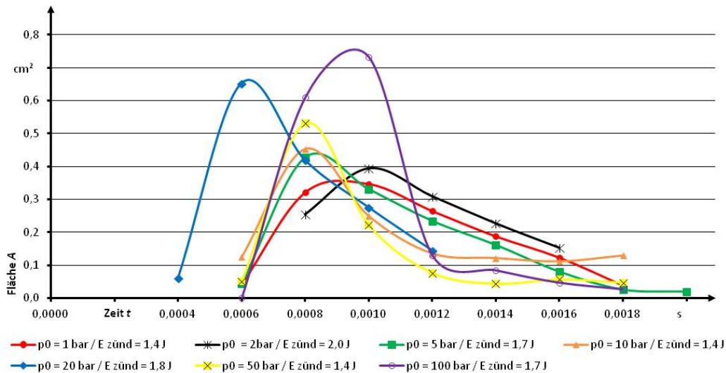
Abb. 54: Expansion des Lichtbogens (Fläche A in \text{cm}^2 ) für explodierenden Draht ( E_{\text{Zünd}} \approx 1 \text{ J} ) in Luft in Abhängigkeit des Anfangsdrucks p_0 , Mittelwert aus drei Versuchen, Aufnahme­frequenz f_a = 5000 \text{ fps} , Zündenergie berechnet aus Strom- und Spannungsverlauf (Mittelwert aus drei Versuchen)
