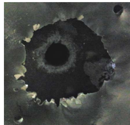
Abb. 69: Ausgebrannte Zünderbohrung (mittig) und weggebrannte Aluminiumplatte des Autoklavenstandes
