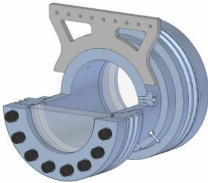
Abb. 19: Schnittdarstellung des an der BAM konstruierten und gebauten Fensterautoklavs
