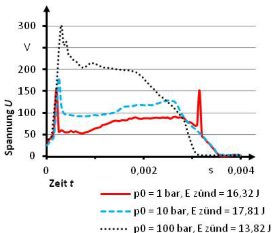
Abb. 52: Spannungsverlauf für explodierenden Draht in Abhängigkeit vom Anfangsdruck für E_{\text{zünd}} = (15 \pm 5) J
