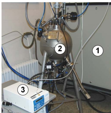
Abb. 23: Versuchsaufbau: Wärmepumpe (1), Autoklav mit Heizmantel (2), HPLC-Pumpe (3)
