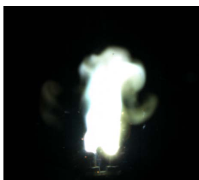
Abb. 29: Highspeedaufnahme ( f_a = 5000 fps) einer Schmelzdrahtzündung
