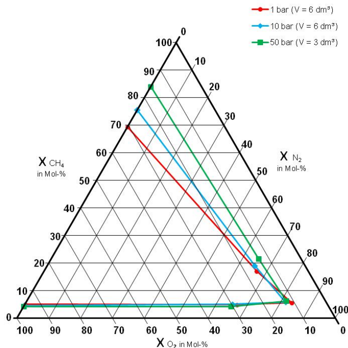
Abb. 63: Explosionsbereiche für CH_4/N_2/O_2 bei p_0 = 1 bar, p_0 = 10 bar und p_0 = 50 bar
