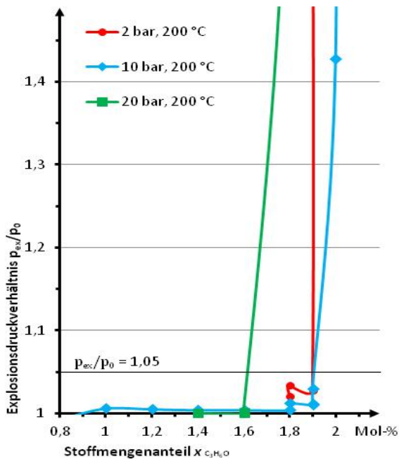
Abb. 44: Explosionsdrucksteigerung in Abhängigkeit vom Brenngasanteil an der UEG für C_3H_6O /Luft bei p_0 = (2, 10, 20) bar und T_0 = 200 °C, schwarze Gerade: Druckschwellenkriterium p_{ex}/p_0 = 1,05
