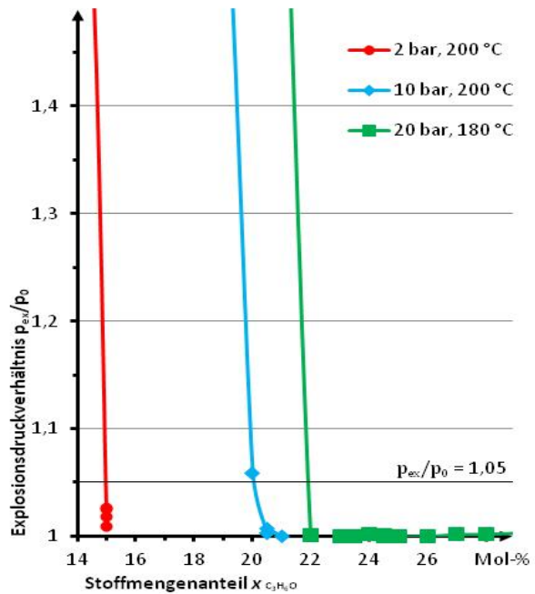
Abb. 45: Explosionsdrucksteigerung in Abhängigkeit vom Brenngasanteil an der OEG für C_3H_6O /Luft bei p_0 = (2, 10, 20) bar und T_0 = (200 bzw. 180) °C, schwarze Gerade: Druckschwellenkriterium p_{ex}/p_0 = 1,05
