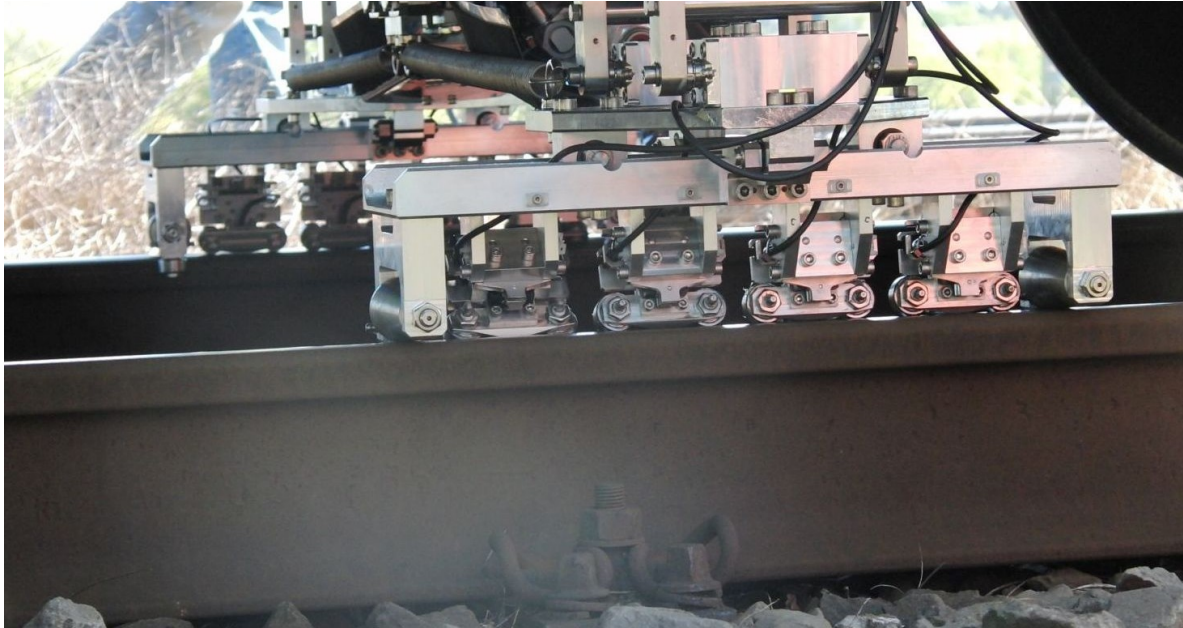
Abbildung 2: Neuentwickelter Sondenträger mit einzelnen Sondenwagen
