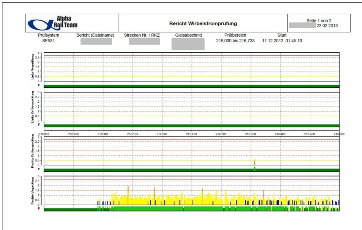
Abbildung 5: Automatisch generierter, vereinfachter Prüfbericht nach Vorgaben der DB
