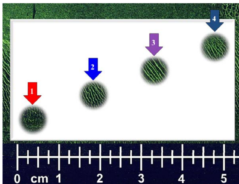
Abb. 3.9. Magnetpulverprüfung an dem Prüfabschnitt mit den Sondenwirkbreiten
