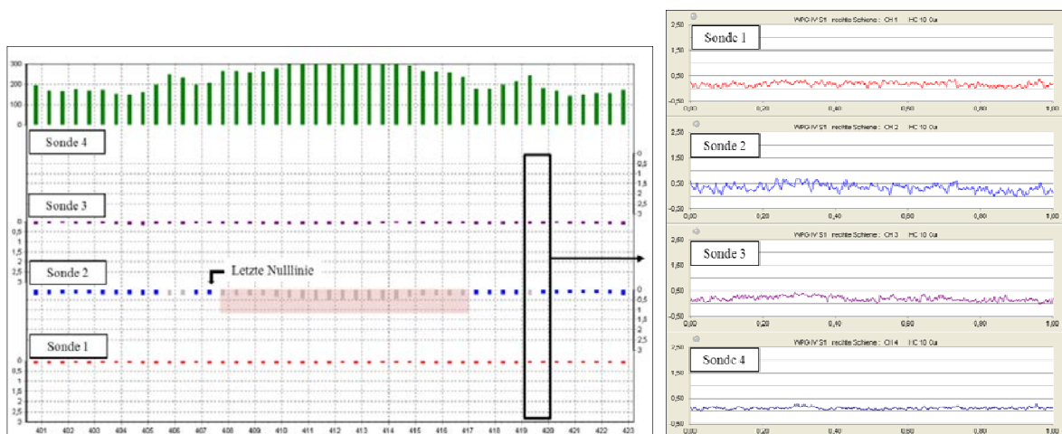
Abb. 3.4. Auswertung erstes Beispiel Stahlsorte R350HT über 22 m und Wirbelstromsignale aus einem Meter
