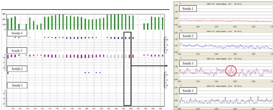
Abb. 3.8. Auswertung der Stahlsorte R370CrHT über 22 m und Wirbelstromsignale aus einem Meter
