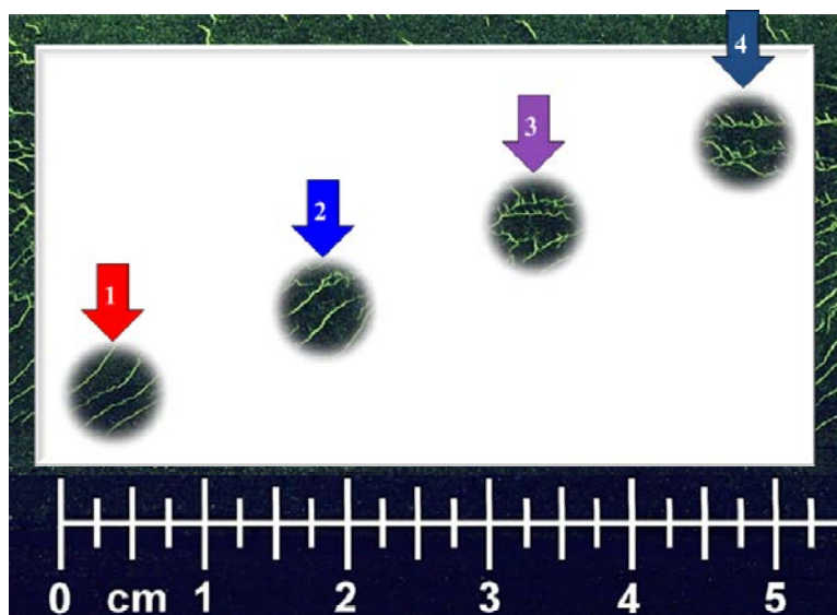
Abb. 3.3. Magnetpulverprüfung an dem Prüfabschnitt mit den Sondenwirkbreiten
