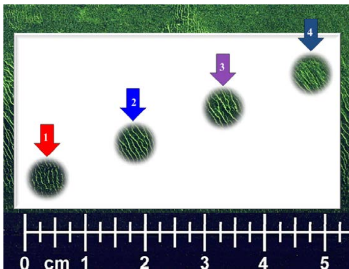
Abb. 3.7. Magnetpulverprüfung an dem Prüfabschnitt mit den Sondenwirkbreiten
