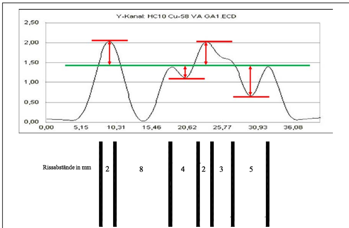
Abb. 2.4. Wirbelstromsignale am Testkörper mit Rissen gleicher Tiefe
