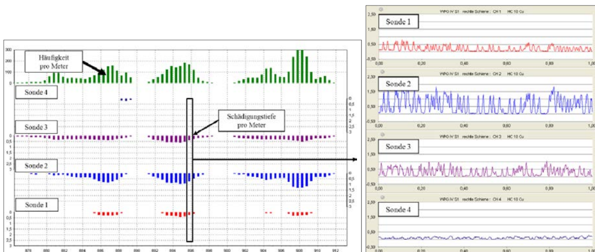
Abb. 3.1. Auswertung erstes Beispiel Stahlsorte R260 über 22 m und Wirbelstromsignale aus einem Meter
