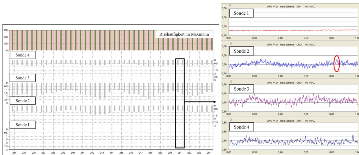
Abb. 3.6. Auswertung zweites Beispiel Stahlorte R350HT über 22 m und Wirbelstromsignale aus einem Meter
