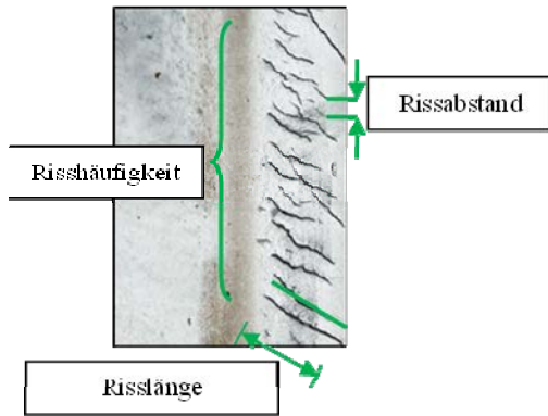
Abb. 2.1. Draufsicht Head Checks
