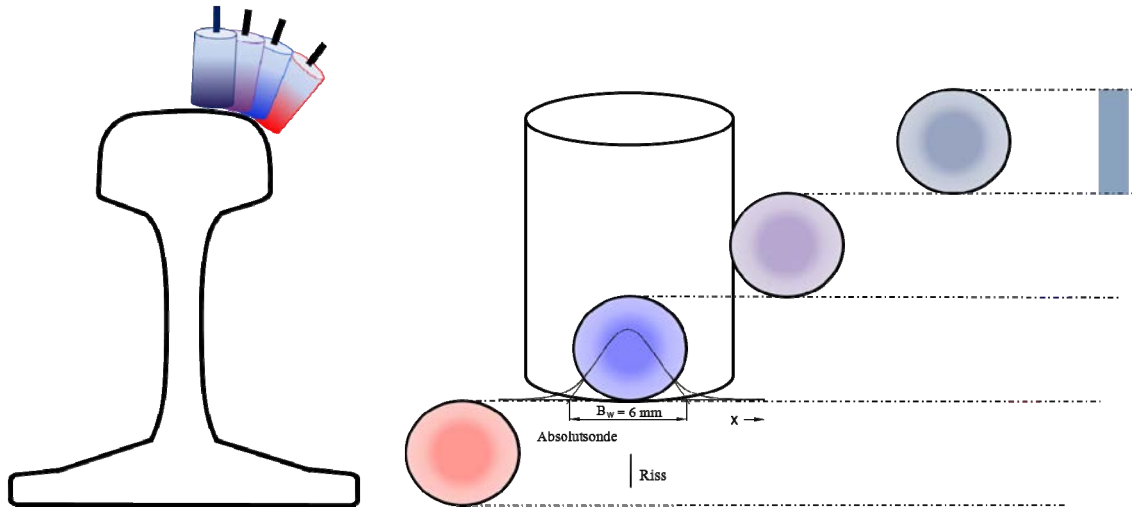
Abb. 2.3. Schematische Darstellung der Sondenpositionen an der Schiene und Wirkbreitenbereich
