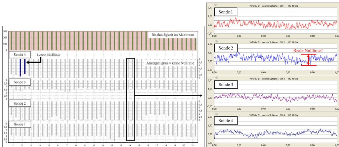
Abb. 3.2. Auswertung zweites Beispiel Stahlsorte R260 über 22 m und Wirbelstromsignale aus einem Meter
