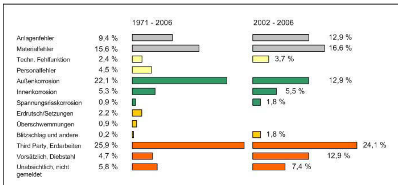
Abb. 3: prozentuale Verteilung der Freisetzungursachen bei Ölpipelines 1971 bis 2006 und 2002-2006
