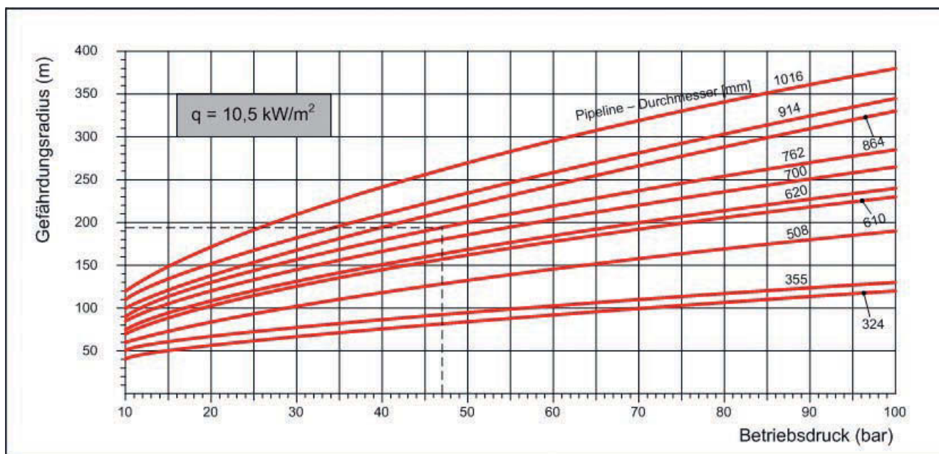
Abb. 10: Gefährdungsradien für eine kritische Bestrahlungsstärke von 10,5 \text{ kW/m}^2
