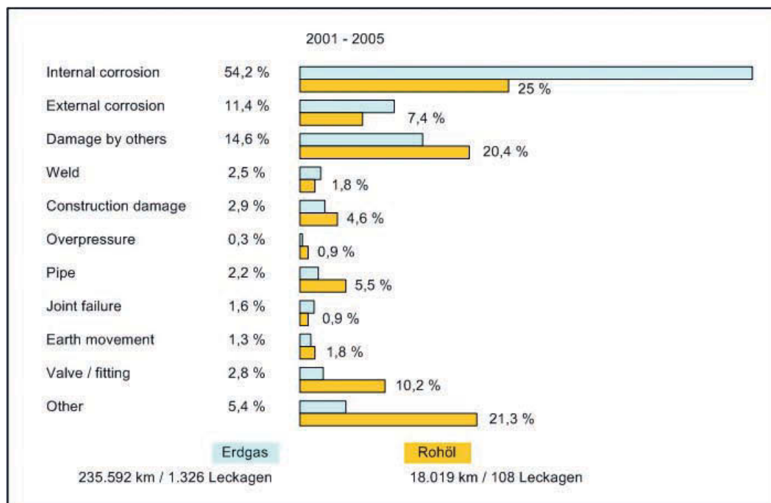
Abb. 4: Ursachen von Pipelineleckagen in der Provinz Alberta/Canada (nach [7])
