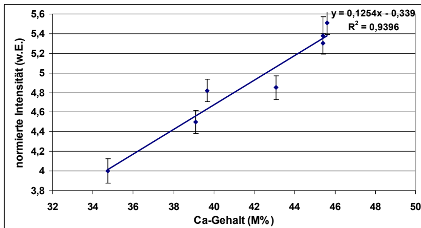
Abbildung 46: Kalibrierfunktion Ca@643,9 nm für Zementstein
