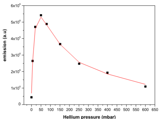
Abbildung 50: Emission der Cl@837,6 nm in Abhängigkeit vom He-Druck nach [AS11]
