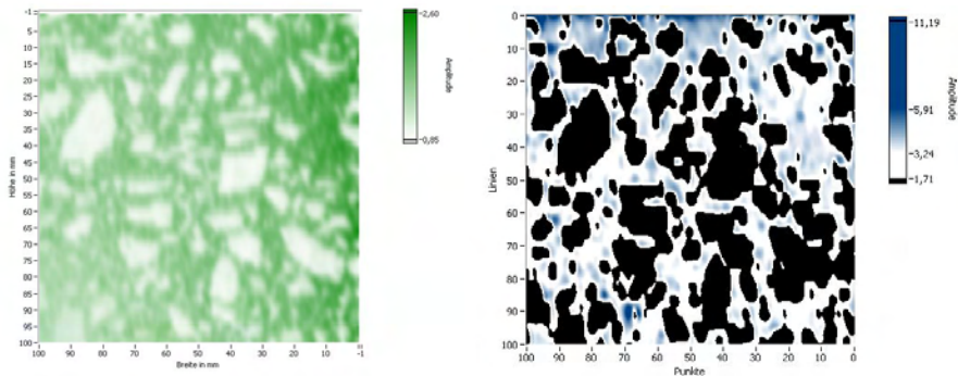
Abbildung 110: Bildgebende Ca-Verteilung mit silikatischen Gesteinskörnungen (links) sowie Na-Verteilung unter Abbildung eines \text{Ca}@825/\text{O}@844} Verhältnis \geq 0,22 (schwarz= Gesteinskörnung mit \text{Ca}/\text{O} < 0,22 ) in einer Probe aus Fahrbahndeckenbeton (rechts)
