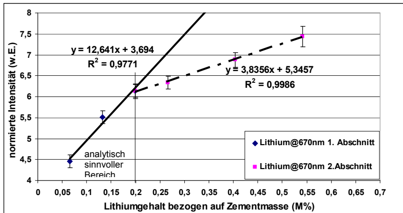
Abbildung 41: Abgestufte Kalibrierfunktionen Li@670,8 nm für Zementstein
