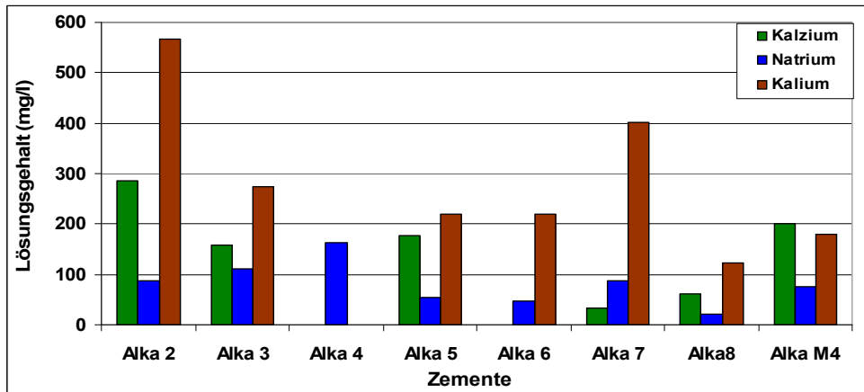
Abbildung 79: Alkalizusammensetzung der veränderten Lösungen in den deion. \text{H}_2\text{O} beaufschlagten Proben
