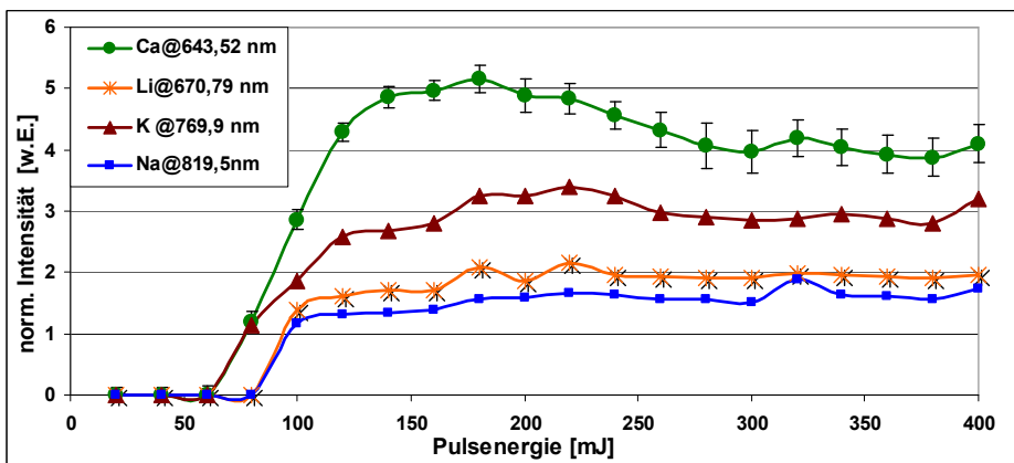
Abbildung 17: Normierte Emissionsintensität (Peak/Untergrund) in Abhängigkeit zur Pulsenergie
