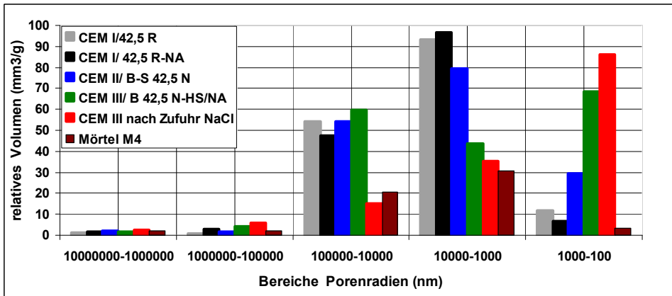
Abbildung 71: Relative Volumenanteile in Abhängigkeit von Porenradienbereichen
