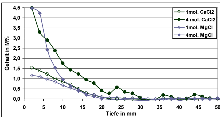
Abbildung 96: Chlorgradient bei Zufuhr von EMH-Lösungen im CEM II/ A-M (Alka 6)
