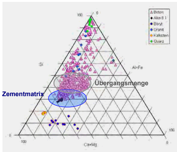
Abbildung 112: Differenzierung der norm. Intensitäten von Zement, Beton und ausgesuchten Gesteinskörnung im Dreistoffdiagramm (Messungen mit Echelle-Spektrometer)
