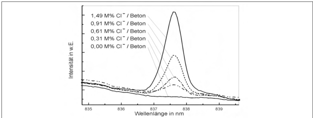
Abbildung 40: Intensität der Spektrallinie Cl@837,6 nm im Verhältnis zum Chlorgehalt des Betons aus [WIL1]
