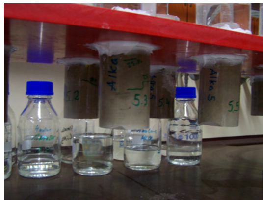
Tafel 3: Übersicht der Proben bei Zufuhr der Lösungen; Markierungen für das Vordringen der Wasserfront
