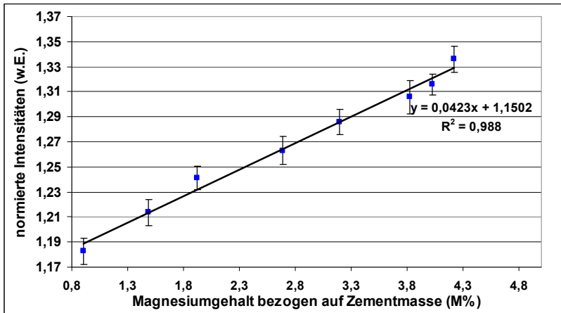
Abbildung 43: Kalibrierfunktion Magnesium Mg@880,7 nm
