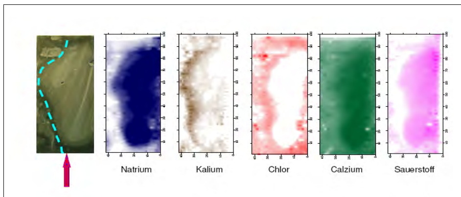
Abbildung 108: Verteilung elementspezifischer, normierter Intensitäten entlang eines Längsrisse; CEM II (Alka 1.2), Zufuhrlösung 4 mol KCl in Pfeilrichtung
