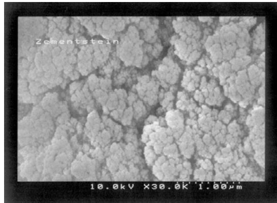
Abbildung 22: Demgegenüber REM-Aufnahme einer unbehandelten, geschnittenen Zementsteinoberfläche
