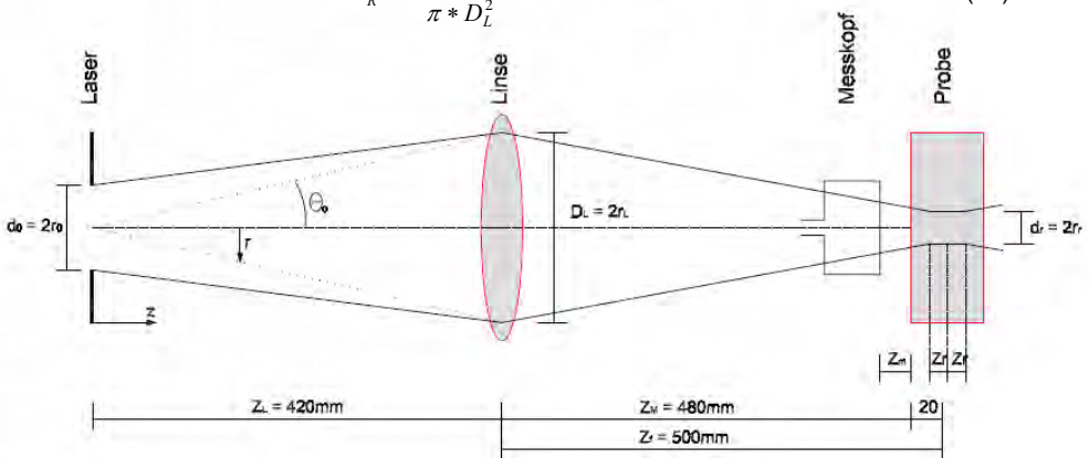
Abbildung 14: Fokussierter Laserstrahl im Meßaufbau
