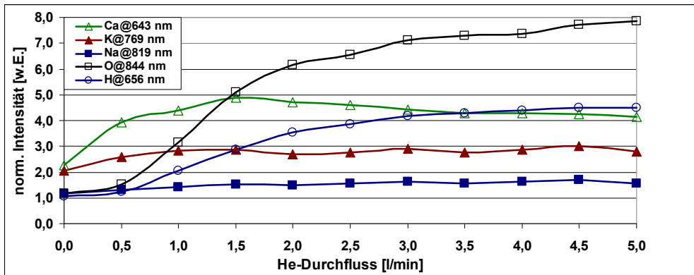
Abbildung 52: Einfluß des He-Spülvolumens auf die normierte Intensität verschiedener Emissionslinien bei Zementstein CEM II (Alka 6, Tabelle 9)
