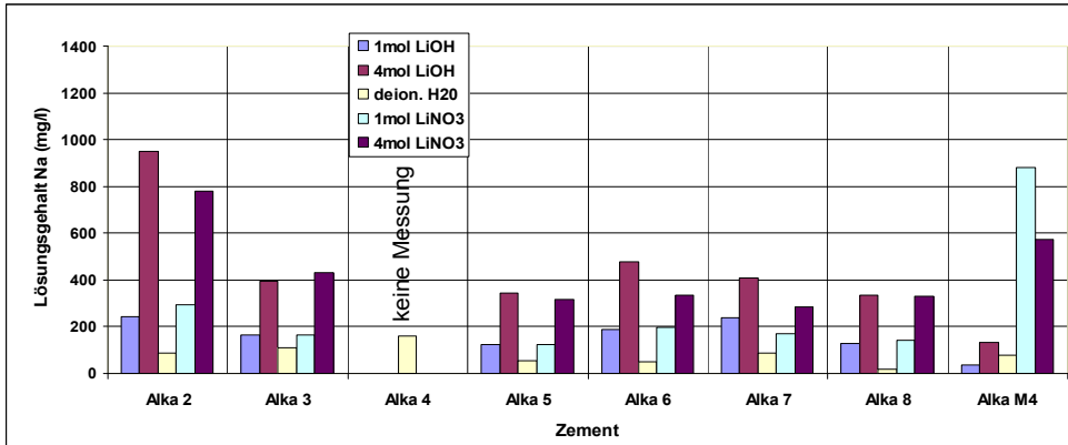
Abbildung 78: Veränderter, spezifischer Natriumgehalt in den lithumbasierten Lösungen nach Abbruch
