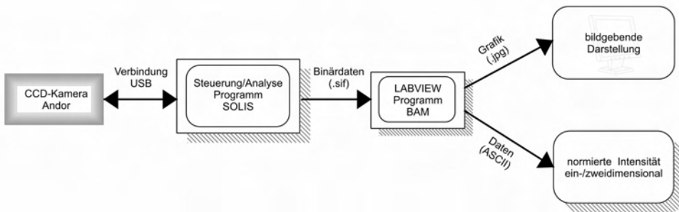
Abbildung 29: Schema der Signal- und Datenverarbeitung
