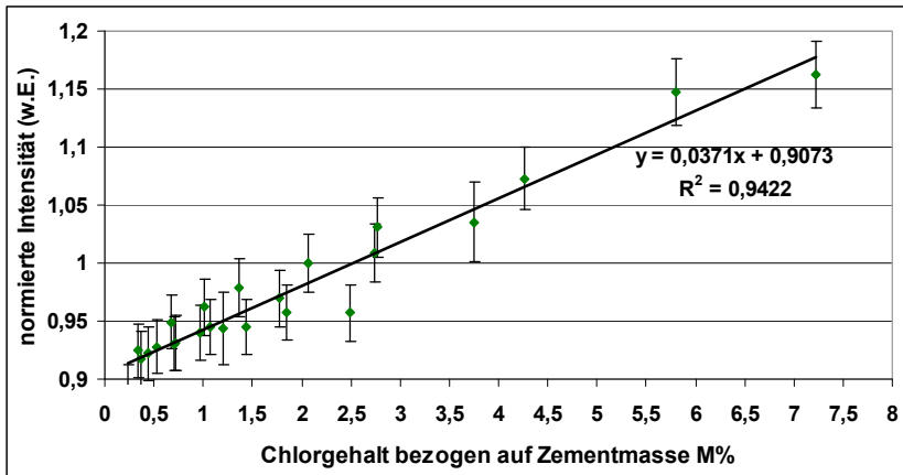
Abbildung 45: Kalibrierfunktion Cl@837,6 nm für Zementstein
