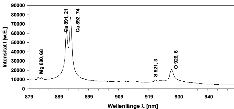
Abbildung 34: Emissionslinien im Spektrum SPZ@913 nm,
