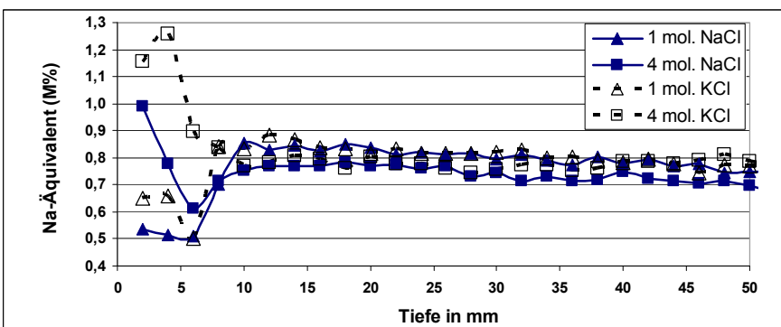
Abbildung 86: Vergleich zu den lösungsspezifischen \text{Na}_2\text{O} -Äquivalenten im CEM III/ B (Alka 8)
