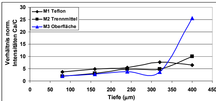
Abbildung 119: Tiefenentwicklung des Verhältnisses normierter Intensitäten \text{Ca}@849/\text{C}@248
