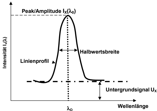
Abbildung 35: Beschreibung der Auswertegrößen an der Spektrallinie
