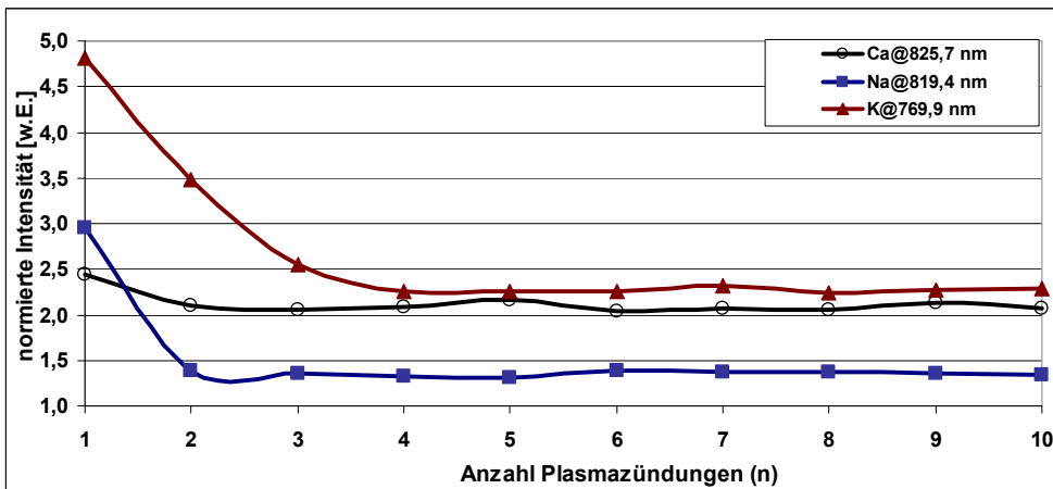
Abbildung 64: Höhere oberflächennahe Intensitäten bei der ersten Plasmazündung; Zementstein CEM II (ALKA 6, Tabelle 9)
