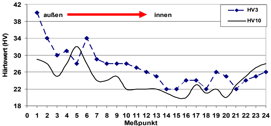
Abbildung 105: Härtewerte nach Vickers in den Prüflasten 3 und 10 kp in Probenquerrichtung
