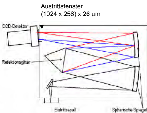
Abbildung 24: Prinzip nach Czerny-Turner
