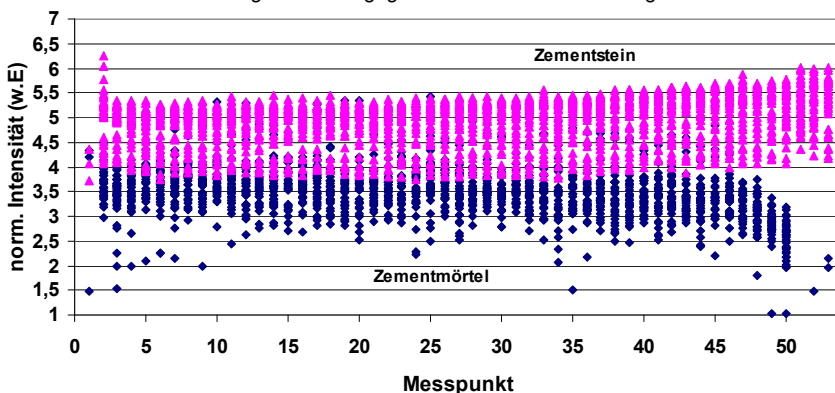
Abbildung 114: Differenzierung im norm. Signal der Linie H@656,3 nm zwischen Zementstein (oben) und Zementmörtel (unten)
