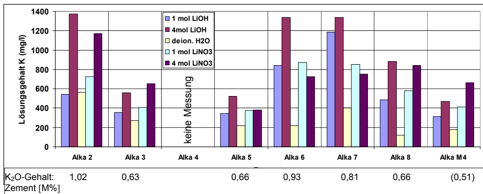
Abbildung 77: Veränderter Kaliumgehalt in den lithumbasierten Lösungen nach Abbruch
