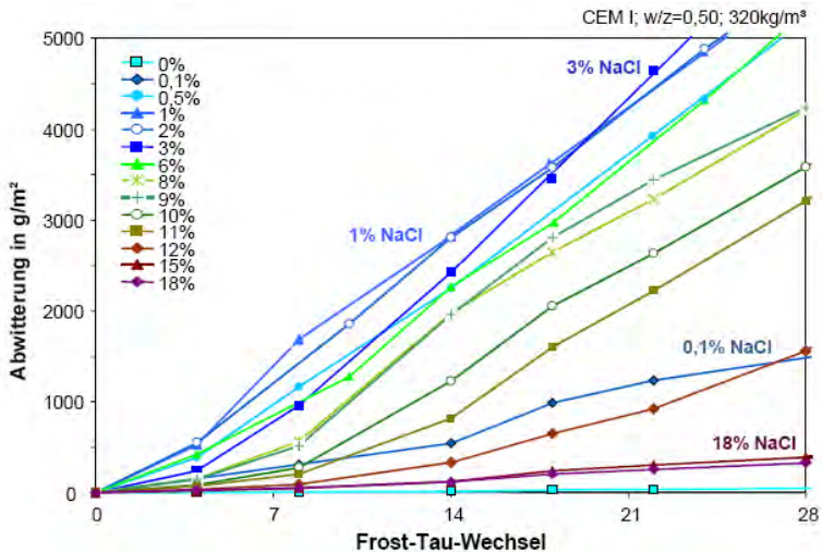
Abbildung 4: Abwitterungsergebnisse eines Beton mit CEM I; w/z=0,5 im CIF- und CDF-Verfahren unter verschiedenen NaCl-Lösungskonzentrationen [SET3]
