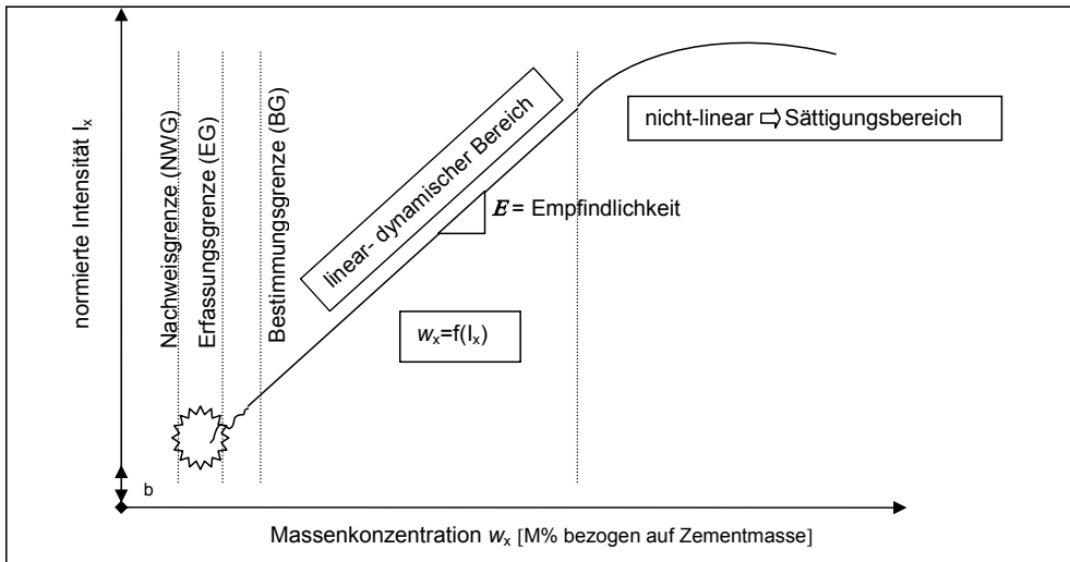
Abbildung 39: Leistungsmerkmale und Abschnitte der Kalibrierfunktion
