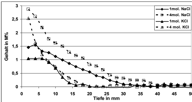
Abbildung 95: Chlorgradient bei hohem Kaliumgehalt mit w(K)=0,867 M% im CEM I/ 42,5 (Alka 2)
