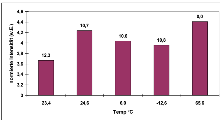
Abbildung 61: Nutzsignal bei K@769,9 nm bei w(K)=0,7 M% in Abhängigkeit von der Proben­temperatur und dem Feuchtigkeitsgehalt (in M% als Wert oberhalb der Diagrammsäulen)
