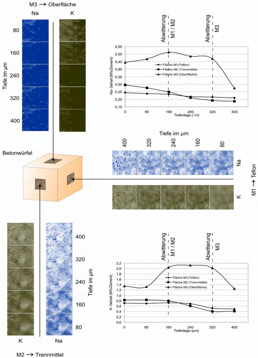
Abbildung 116: Durch schichtenweises Ablatieren erzielte oberflächennahe Elementverteilung von Na und K in Abhängigkeit von der Schaffläche
