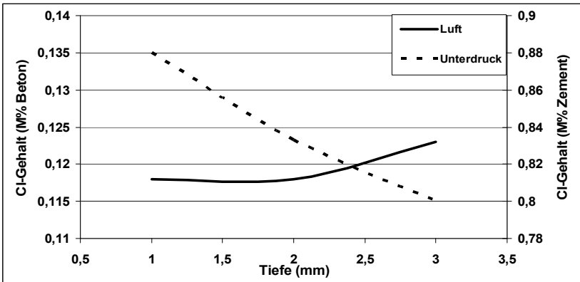
Abbildung 58: Veränderungen im Chlorgradient bei Proben im Unterdruck und Atmosphärendruck
