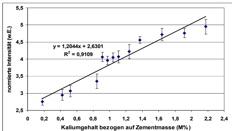
Abbildung 42: Kalibrierfunktion der Emissionslinie K@769,9 nm
