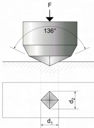
Abbildung 102: Bestimmung der Vickers-Härte
