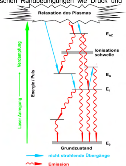
Abbildung 9: Prinzip der Anregung und spektralen Emission
