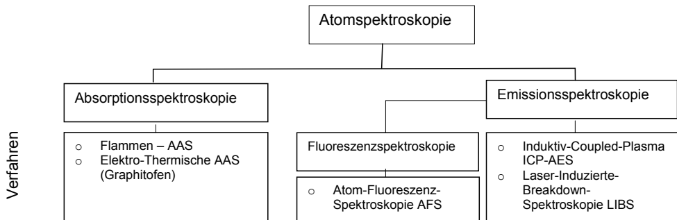
Abbildung 6: Übersicht über ausgesuchte atomspektroskopische Analyseverfahren
