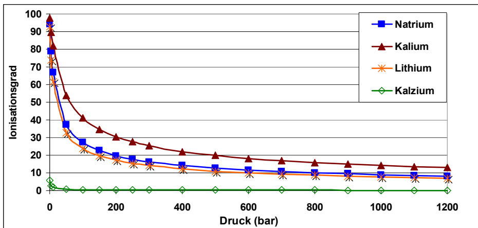
Abbildung 57: Zusammenhang zwischen Ionisationsgrad und Druck nach der Saha-Gleichung bei T=10000^{\circ}\text{K}
