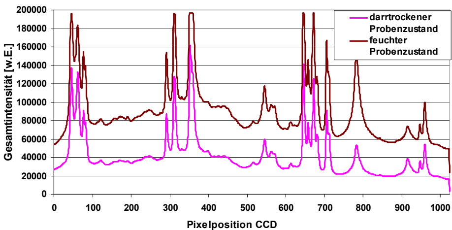
Abbildung 62: Gesamtintensität und Untergrundsignal im Spektrum \text{SPZ}@630 \text{ nm} in Abhängigkeit von der Probenfeuchtigkeit an Zementstein CEM I, NA (Alka 4, Tabelle 9) mit \text{KCl} -Beaufschlagung (feucht= 13 M% freies \text{H}_2\text{O} )
