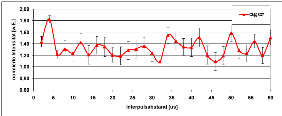
Abbildung 49: Intensitätsänderungen bei Doppelpulsanregung bei \text{Cl@837,6 nm} im Spektrum 808nm unter Luftatmosphäre (Steinsalzprobe ILT)
