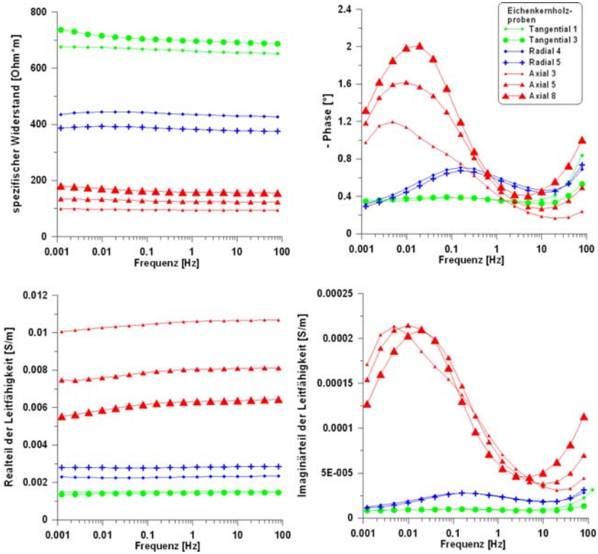
Abbildung 5.3: Vergleich der richtungsabhängigen Messungen von Eichenkernholzproben. Dabei sind deutliche Unterschiede zwischen den axialen, radialen und tangentialen Proben zu sehen.
