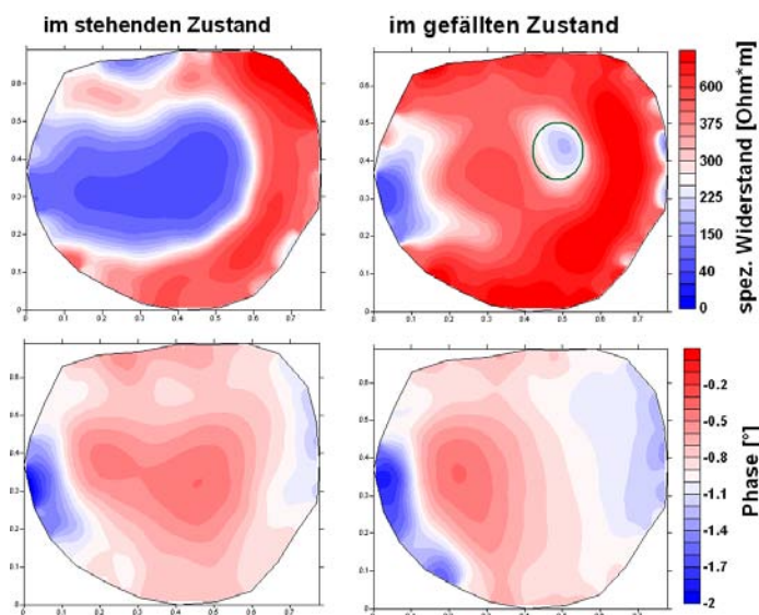
Abbildung 6.9: Eiche Nr. 1 - Pilzbefall: Vergleich der Tomographieergebnisse von Mesesebene 2 für f = 0,312 Hz. Links die Messung am stehenden Baum (vgl. Abb. 6.8), rechts am selben Stammstück nach 4-wöchiger Trocknung an der Luft. Der am stärksten befallene Bereich zeichnet sich durch hohe spezifische Widerstände und niedrige Phasen aus.
