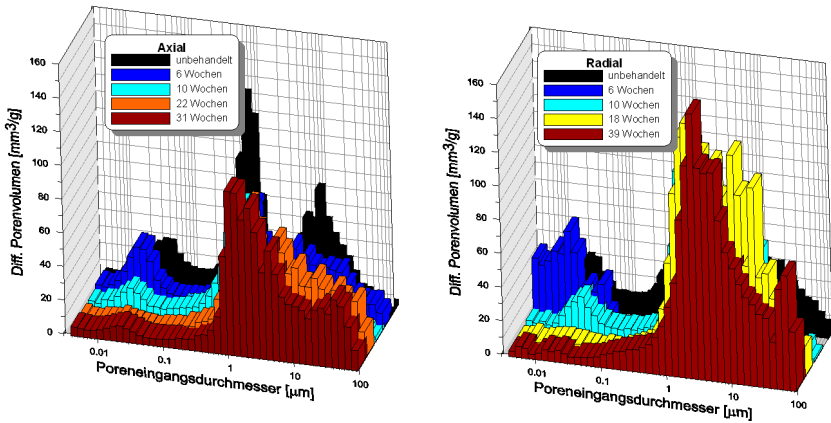
Abbildung 5.17: Dreidimensional Darstellung der Verteilung der Poreneingangsdurchmesser für ausgewählte axiale (links) und radiale Proben. Mit zunehmender Inkubationszeit wird aus der trimodalen eine beinahe unimodale Verteilung.
