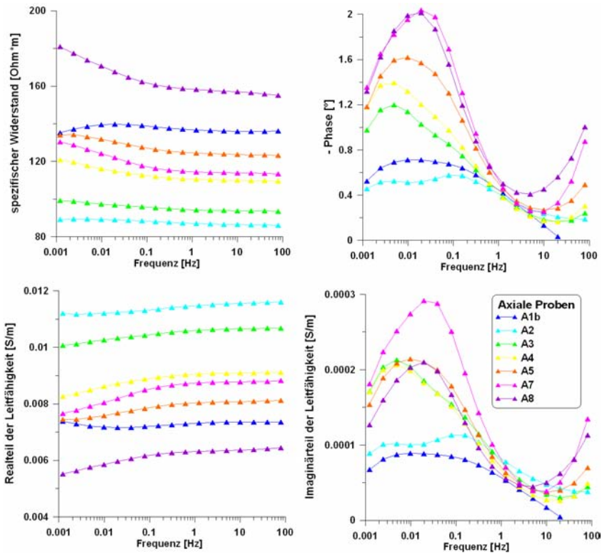
Abbildung 5.2: Spektren der axialen Eichenkernholzproben. Es zeigt sich eine Abhängigkeit des spezifischen Widerstands, der Phase und der realen und imaginären Leitfähigkeit vom Entnahmeort. Proben von der Stammachse (Probe A1b, A2) sind in der Tendenz leitfähiger und weniger polarisierbar als Proben in der Nähe des Baumrandes (Probe A8).
