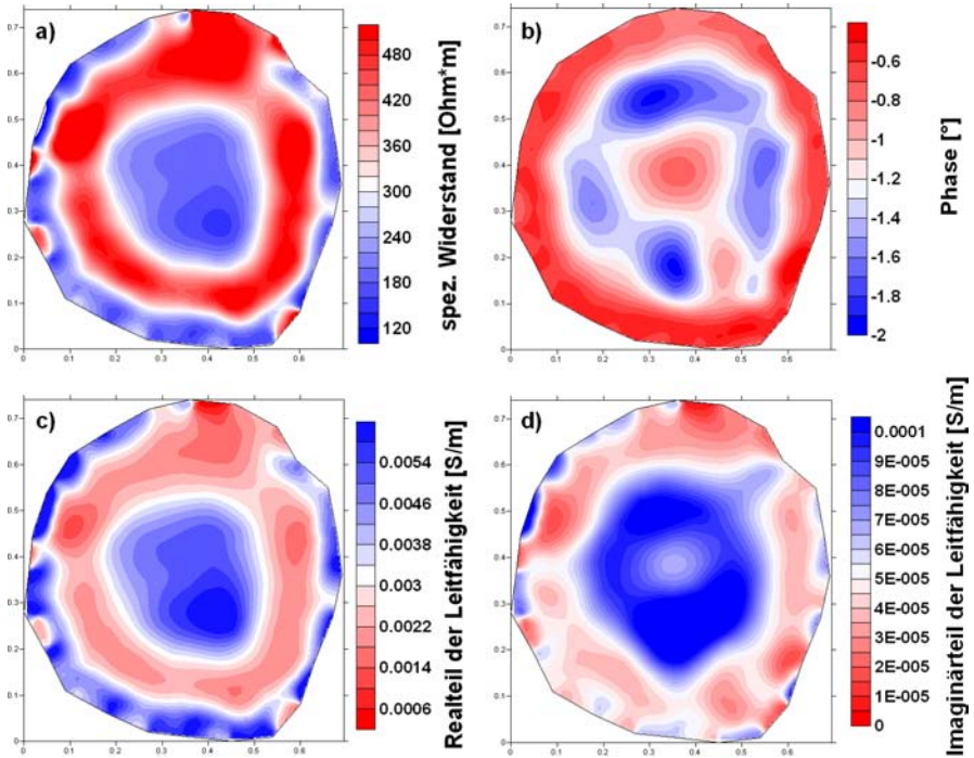
Abbildung 6.1: Tomogramme des spezifischen Widerstands (a), der Phasenverschiebung (b) und des Real- (c) und Imaginärteil (d) der Leitfähigkeit einer gesunden Eiche (Referenzreihe) auf dem BAM Testgelände für die Frequenz 0,156 Hz im Sommer. Deutlich sind konzentrische, ringförmige Strukturen zu erkennen.
