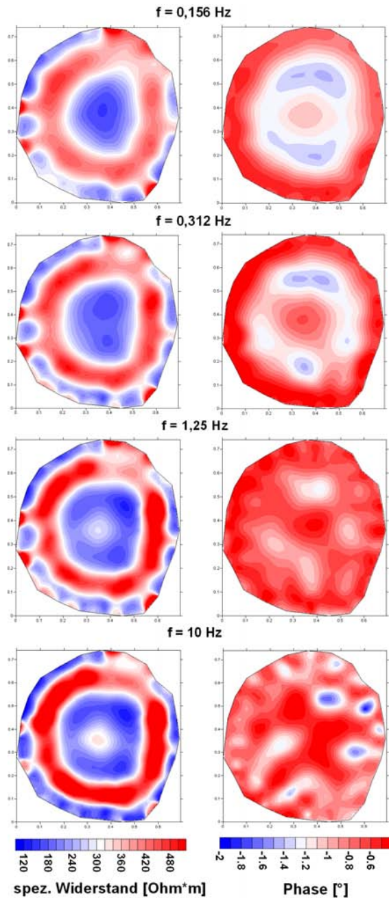
Abbildung 6.2: Frequenzabhängige Tomogramme des spezifischen Widerstands (links) und der Phasenverschiebung (rechts) der Referenzreihe im Sommer 2008. Während im spezifischen Widerstand nur geringfügige Änderungen erkennbar sind, werden die Tomogramme der Phasenverschiebung bei Frequenzen über 1 Hz deutlich unstrukturierter.
