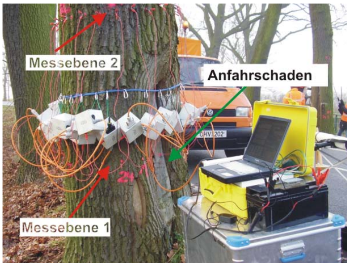
Abbildung 6.7: Foto des Messaufbaus an einer Eiche (Nr. 1) mit Anfahrtschaden. Die Messungen fanden in zwei Ebenen statt.
