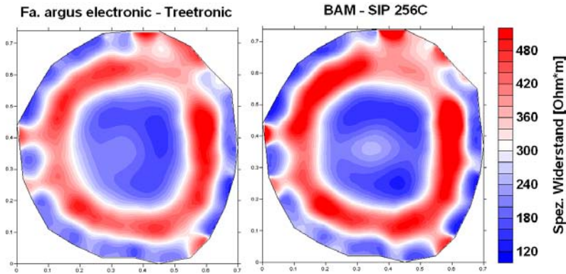
Abbildung C.3: Vergleich zwischen den spezifischen Widerstandsmessungen an der Referenzreihe (August 2007). Links: Messhardware Treetronic der Fa. argus electronic (Lothar Göcke), invertiert mit DC2dTree. Rechts: Messhardware SIP 256C, invertiert mit DC2dTree ( f = 0,156 Hz). Zwischen beiden Tomogrammen bestehen nur sehr geringe Unterschiede.
