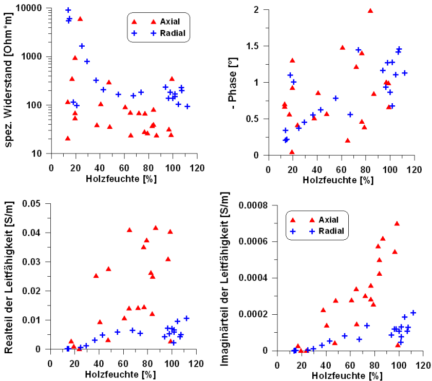
Abbildung 5.16: Spezifischer Widerstand, Phase, Real- und Imaginärteil der Leitfähigkeit aufgetragen über die Holzfeuchte für axiale und radiale Proben. Die Phase nimmt tendenziell mit steigender Holzfeuchte zu. Der spezifische Widerstand nimmt bis zu einer Holzfeuchte von ca. 50 % stark ab. Real- und Imaginärteil der Leitfähigkeit nehmen für beide Orientierungen unterschiedlich stark zu.
