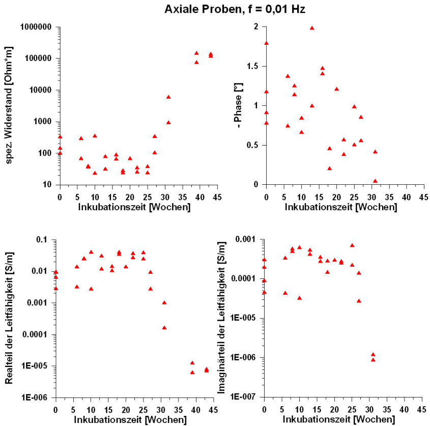
Abbildung 5.13: Spezifischer Widerstand, Phase, reelle und imaginäre Leitfähigkeitsanteile aufgetragen über die Inkubationszeit bei der Frequenz des Phasenmaximums ( f=0,01 Hz) für die axialen Proben. Ab einer Inkubationszeit von 25 Wochen ist eine Trendumkehr zu beobachten.
