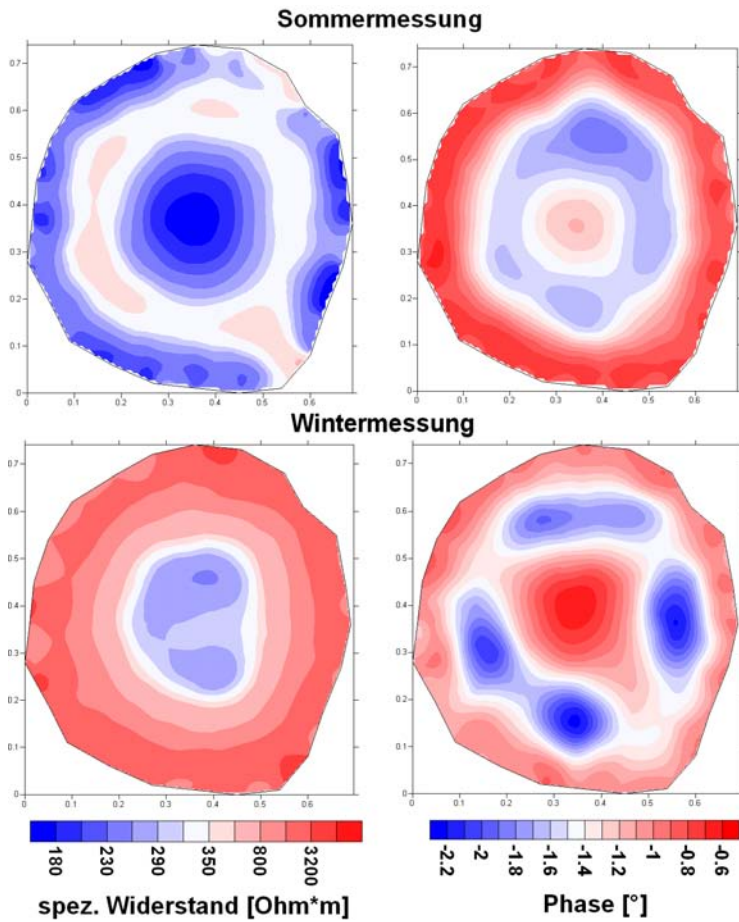
Abbildung 6.3: Jahreszeitenabhängige Tomogramme des spezifischen Widerstands (links) und der Phasenverschiebung (rechts) der Referenzreihe (Dipol-Dipol-Konfiguration). Im Winter (untere Tomogramme) sind infolge des eingestellten Wassertransportes und des Temperatureffektes die spezifischen Widerstände wesentlich höher.
