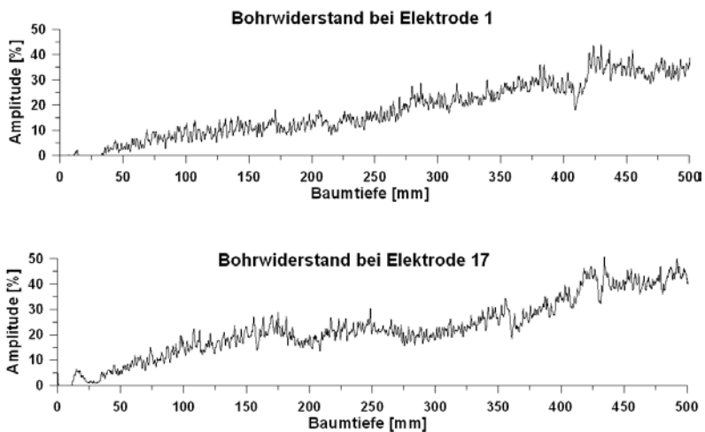
Abbildung C.2: Bohrwiderstandsmessungen an der Referenzeiche. Der Bohrkanal befindet sich bei den SIP-Messelektroden 1 (oben) und 17. Der mechanische Bohrwiderstand nimmt in Richtung Bauminneres zu. Der Baum ist an den gebohrten Stellen gesund.
