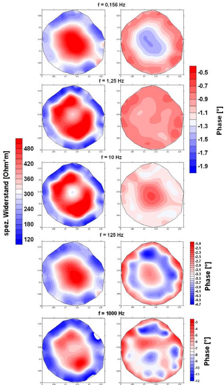
Abbildung 6.5: Frequenzabhängige Tomogramme des spezifischen Widerstands und der Phasenverschiebung für eine gesunde, 60-jährige Eiche im Sommer 2008. Achtung: für f = 125 \text{ Hz} und für f = 1000 \text{ Hz} ändert sich die Farbskala der Phase.
