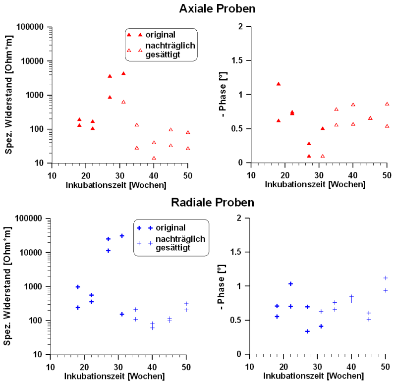
Abbildung B.14: Versuch mit dem Schwefelporling. Spezifischer Widerstand und Phase aufgetragen über die Zeit für das jeweilige Phasenmaximum ( f_{max}^{axial} = 0,1 Hz, f_{max}^{radial} = 0,01 Hz). Unterscheidung zwischen Proben ohne zusätzliche Sättigung (original) und mit nachträglicher Sättigung.
