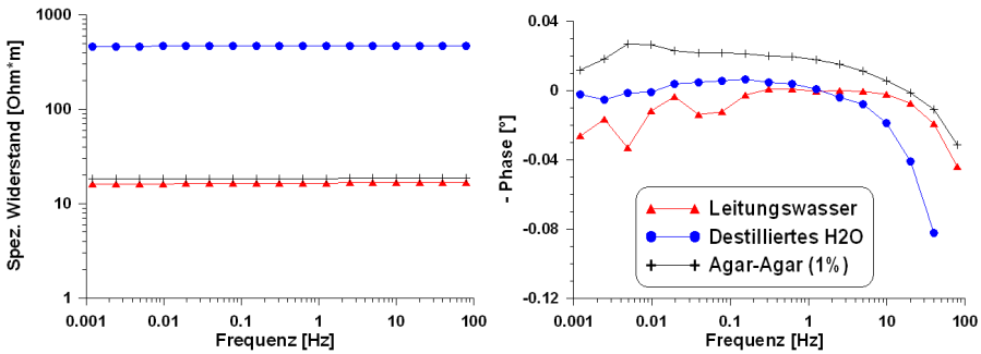
Abbildung 3.5: Links: Spezifischer Widerstand einer mit Leitungswasser, destilliertem Wasser und mit 1%-iger Agar-Agar-Lösung gefüllten Messzelle. Rechts: Zugehörige Phasendarstellung. Alle drei Ankopplungsmittel weisen erst bei höheren Frequenzen Eigeneffekte auf.
