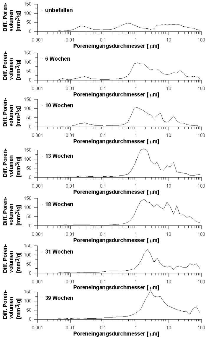
Abbildung B.7: Poreneingangsdurchmesser für alle in Kapitel 5.3.1 untersuchten radialen Eichenwirrlingsproben. Oben ist die unfallenen Probe zu sehen; darauf folgend die Proben mit zunehmender Inkubationszeit.
