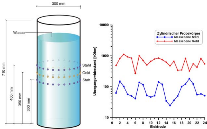
Abbildung 4.1: Schematische Zeichnung des zylindrischen Probekörpers. In dem nach unten abgedichteten und nach oben offenen Rohr wurden drei Elektrodenebenen angebracht. Die äußeren beiden bestanden aus herkömmlichen Stahlelektroden, die mittlere Ebene aus Goldelektroden. Das Rohr war für die Versuche mit Wasser gefüllt.
