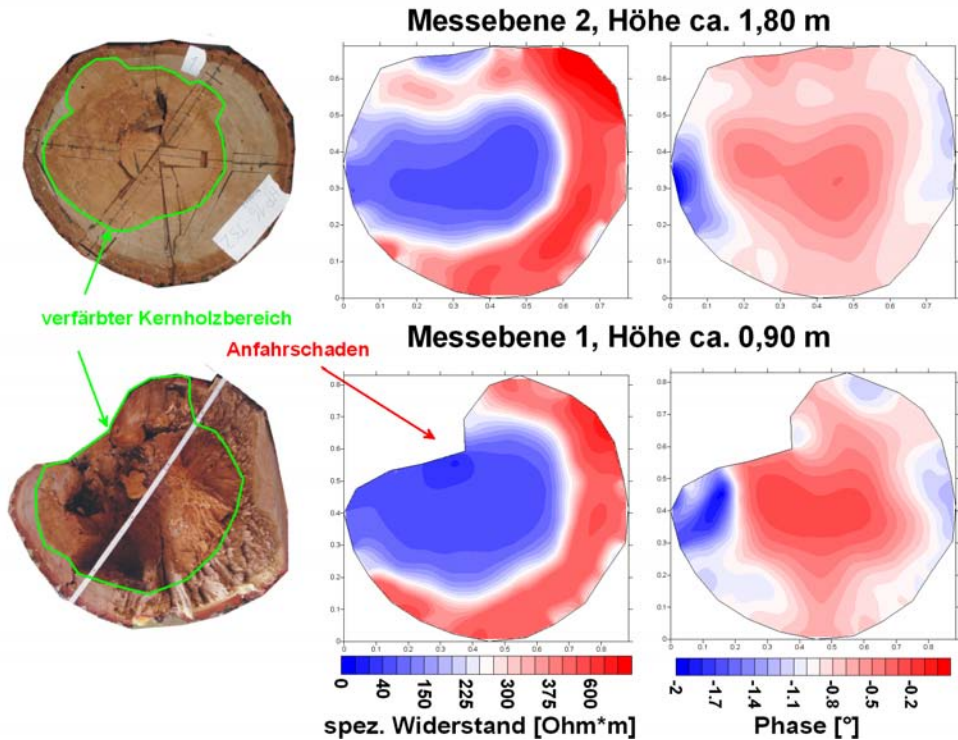
Abbildung 6.8: Eiche Nr. 1 - Pilzbefall: Foto (links) und Tomogramme des spezifischen Widerstands (mittig) und der Phase (rechts) für beide Messebenen ( f = 0,312 Hz). Der befallene Bereich stellt sich als niederohmige Anomalie im spezifischen Widerstand dar.
