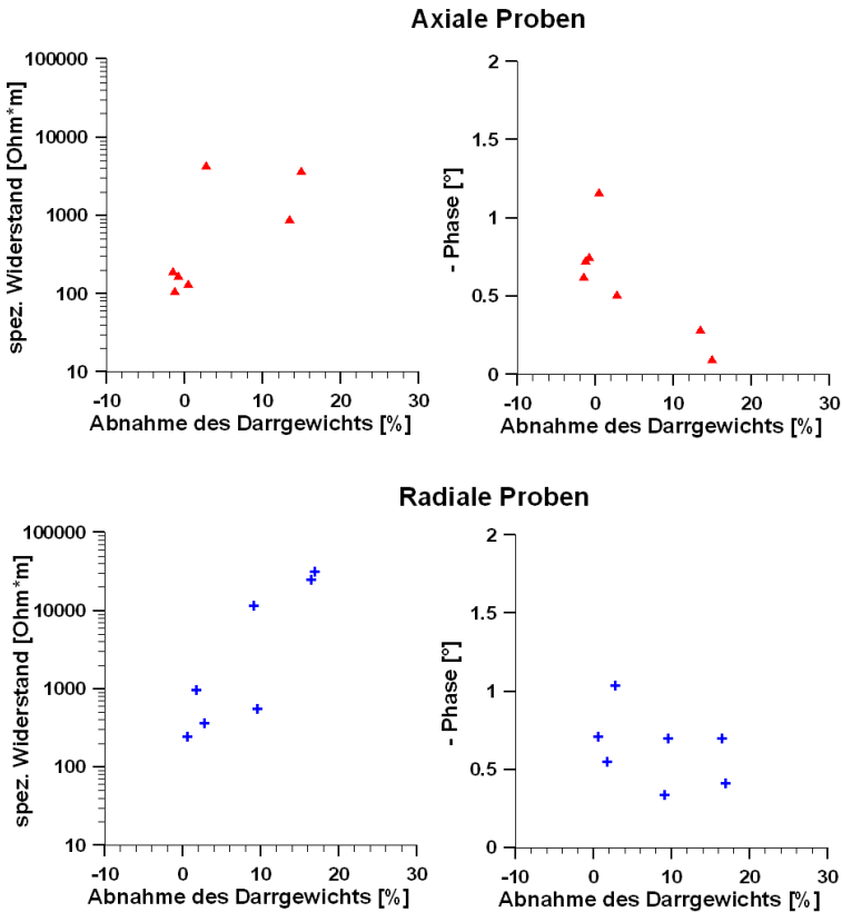
Abbildung 5.24: Versuch mit dem Schwefelporling. Darstellung des spezifischen Widerstands und der Phase aufgetragen gegen die Abnahme des Darrgewichts für axiale (oben) und radiale (unten) Proben. Mit Abnahme des Darrgewichts steigen die spezifischen Widerstände und sinken die Phasen.
