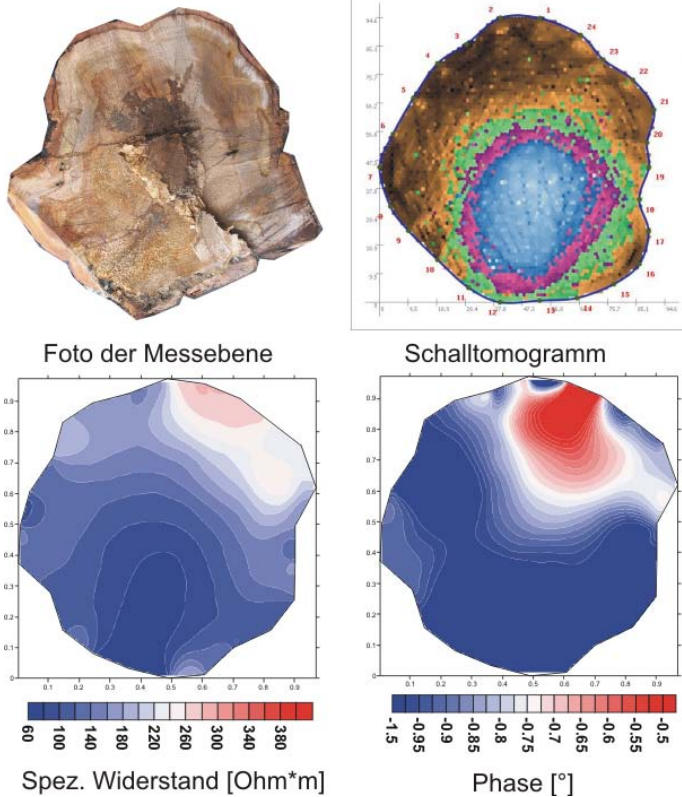
Abbildung 6.13: Eiche Nr. 2 - Pilzbefall: Tomogramme des spezifischen Widerstands und der Phase für f = 0,312 Hz sowie von der Schallmessung für Messebene 1. Im Vergleich dazu das unmittelbar nach der Fällung aufgenommene Foto.
