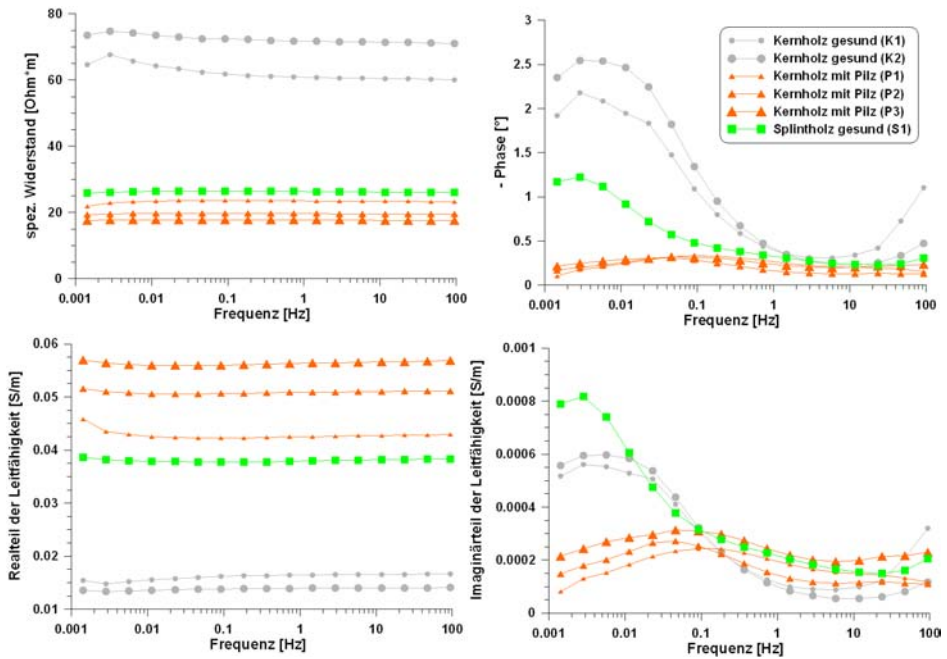
Abbildung 5.32: Spezifischer Widerstand, Phase, Real- und Imaginärteil der Leitfähigkeit einer mit Schwefelporling infizierten Eiche. Die unbeefallenen Kernholzproben haben niedrige spezifische Widerstände ( \sim 70 \Omega\text{m} ). Diese werden durch den Pilzbefall deutlich verringert. In der Phase sind die pilzbeefallenen Kernholzproben eindeutig von den anderen Kernholzproben unterscheidbar.
