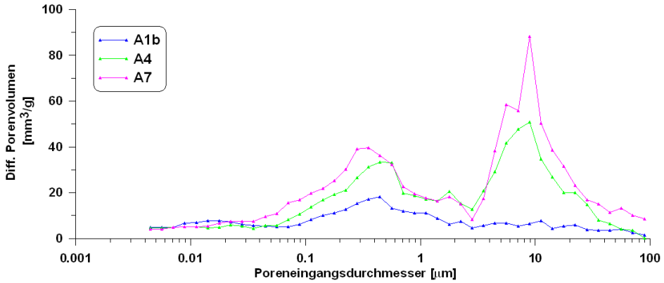
Abbildung 5.4: Verteilung der Poreneingangsdurchmesser für drei axiale Eichenkernholzproben.
