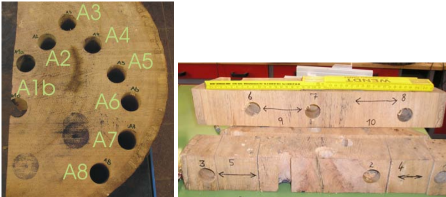
Abbildung 5.1: Fotos der Probenentnahme für die Anisotropiemessungen. Links: axiale Probenentnahme. Rechts: radiale und tangentialen Probenentnahme.
