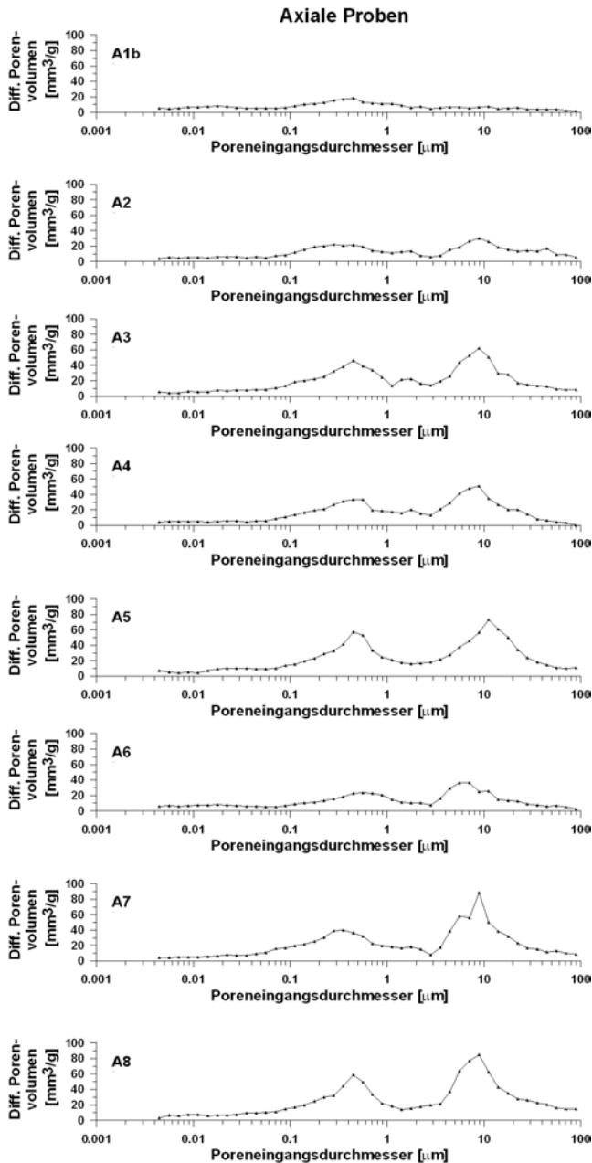
Abbildung B.3: Verteilung der Poreneingangsdurchmesser für alle im Anisotropiever- such (Kap. 5.1) gemessenen axialen Proben. Proben A3, A5 und A8 wurden mit einem anderen Quecksilberporositätsmessgerät gemessen als die restlichen Proben.
