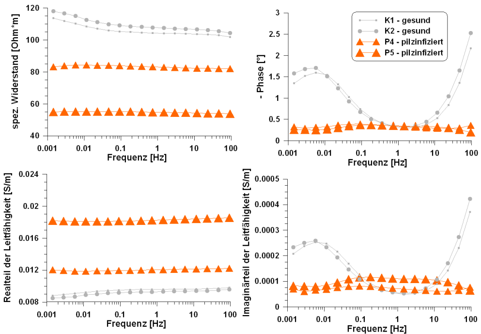
Abbildung 5.30: Spektren der mit dem Eichenwirrling befallenen Eichenkernholzproben. Deutliche Unterschiede zwischen gesunden und infizierten Proben sind zu sehen.
