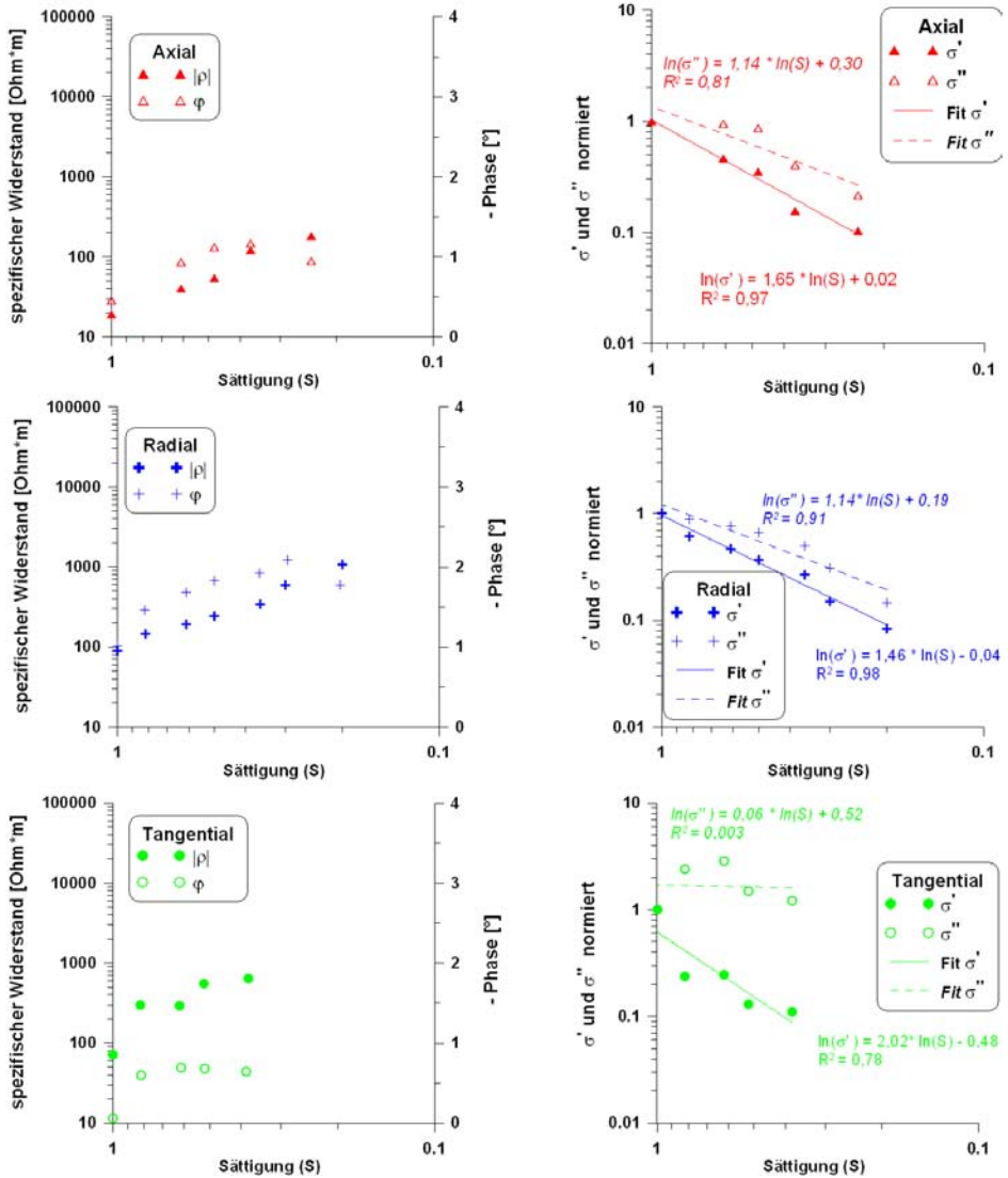
Abbildung 5.8: Entsättigungsversuch 1 an Eichenkernholz. Links: Spezifischer Widerstand und Phase für f = 0,183 Hz aufgetragen über die Sättigung über die Sättigung für axiale, radiale und tangentiale Proben. Rechts: Normierte reelle und imaginäre Leitfähigkeiten als Funktion der Sättigung.
