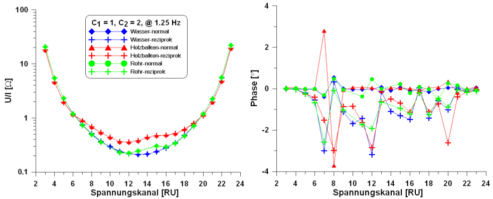
Abbildung 4.5: Vergleich von normalen und reziproken Daten für den ersten Stromdipol C_1 = 1 , C_2 = 2 . Die Unterschiede in den scheinbaren Widerständen sind gering, während in der Phasenverteilung die Daten weniger gut übereinstimmen.
