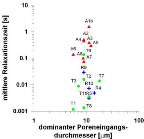
Abbildung 5.6: Mittlere Relaxationszeit aufgetragen über den dominanten Poreneingangsdurchmesser für axiale, radiale und tangentielle Eichenkernholzproben.
