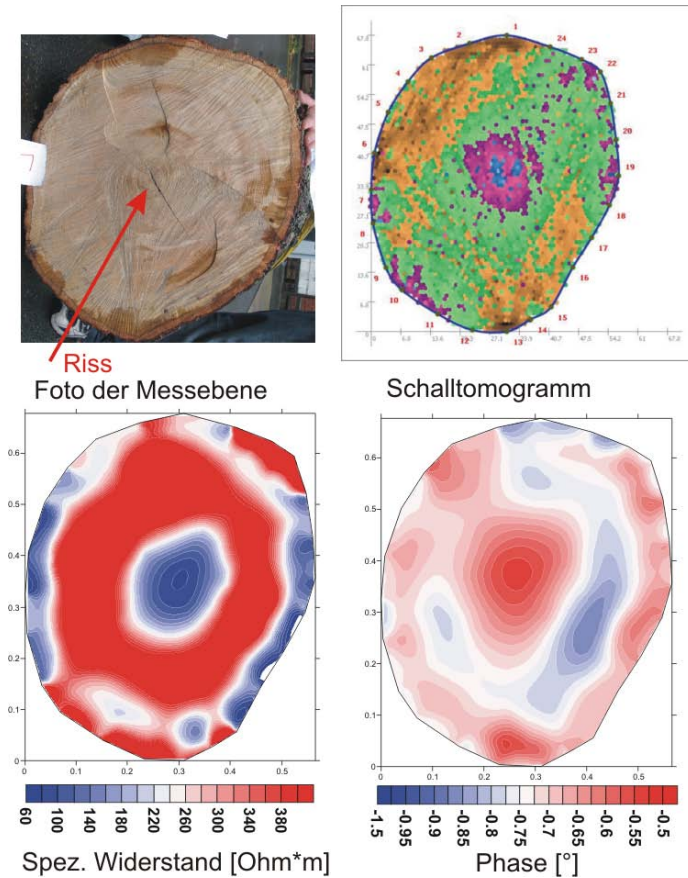
Abbildung 6.14: Eiche Nr. 2 - Pilzbefall: Tomogramme des spezifischen Widerstands und der Phase für f = 0,312 Hz sowie von der Schallmessung für Messebene 2. Im Vergleich dazu das unmittelbar nach der Fällung aufgenommene Foto.
