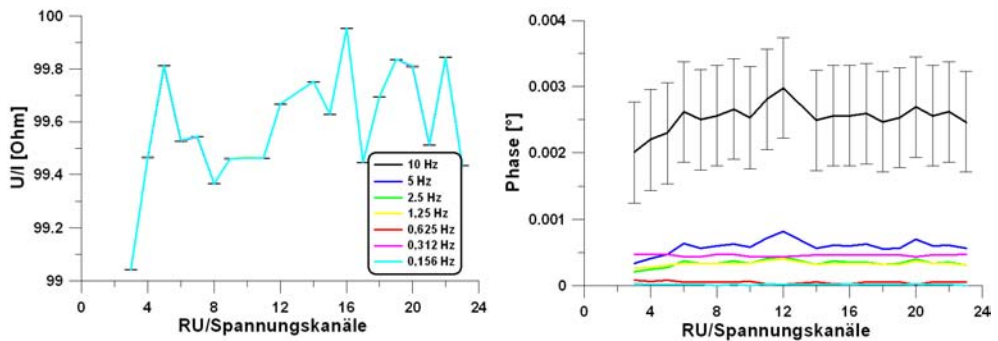
Abbildung A.1: Ergebnisse der Widerstands- und Phasenmessung am Testnetzwerk mit der SIP 256C für verschiedene Frequenzen. Die Widerstandsdaten sind frequenzunabhängig. In der Phase zeigt sich eine Zunahme der Phase mit steigender Frequenz. Der vom Gerät ausgegebene Messfehler für f = 10 Hz ist mitdargestellt. Für alle anderen Frequenzen ist er ähnlich groß.
