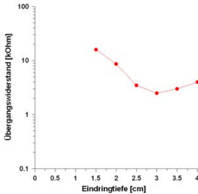
Abbildung 4.2: Übergangswiderstände an einer Eiche ( Quercus robur ) in Abhängigkeit von der Eindringtiefe der Nägel. Die niedrigsten Übergangswiderstände wurden bei einer Eindringtiefe von 3 cm erreicht.
