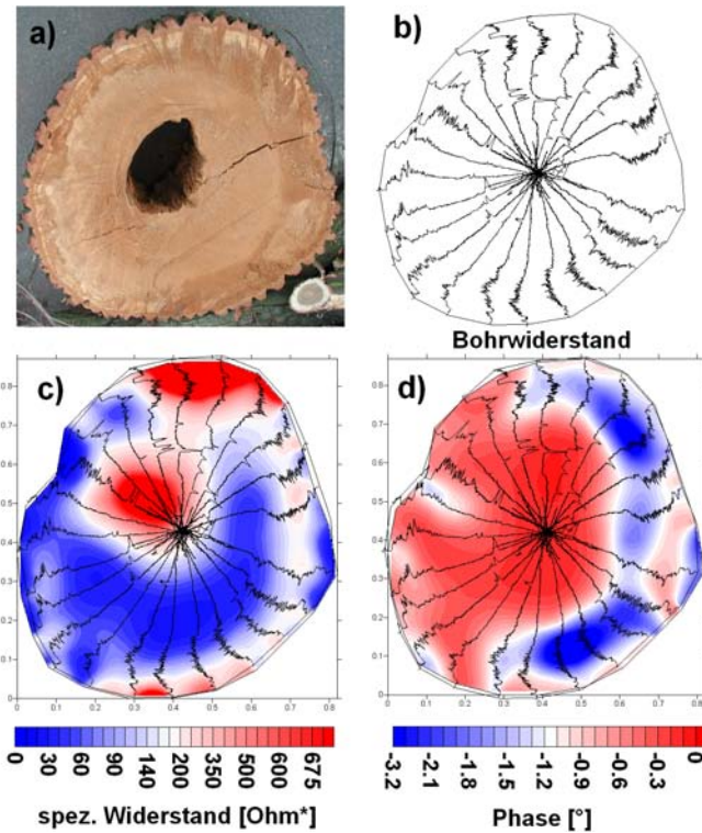
Abbildung 6.18: Eiche Nr. 3 - Pilzbefall: Foto der Messebene 2 (a), Bohrwidstandsdaten (b) sowie die Daten des spezifischen Widerstands(c) und der Phasenverschiebung (d) zum Vergleich.
