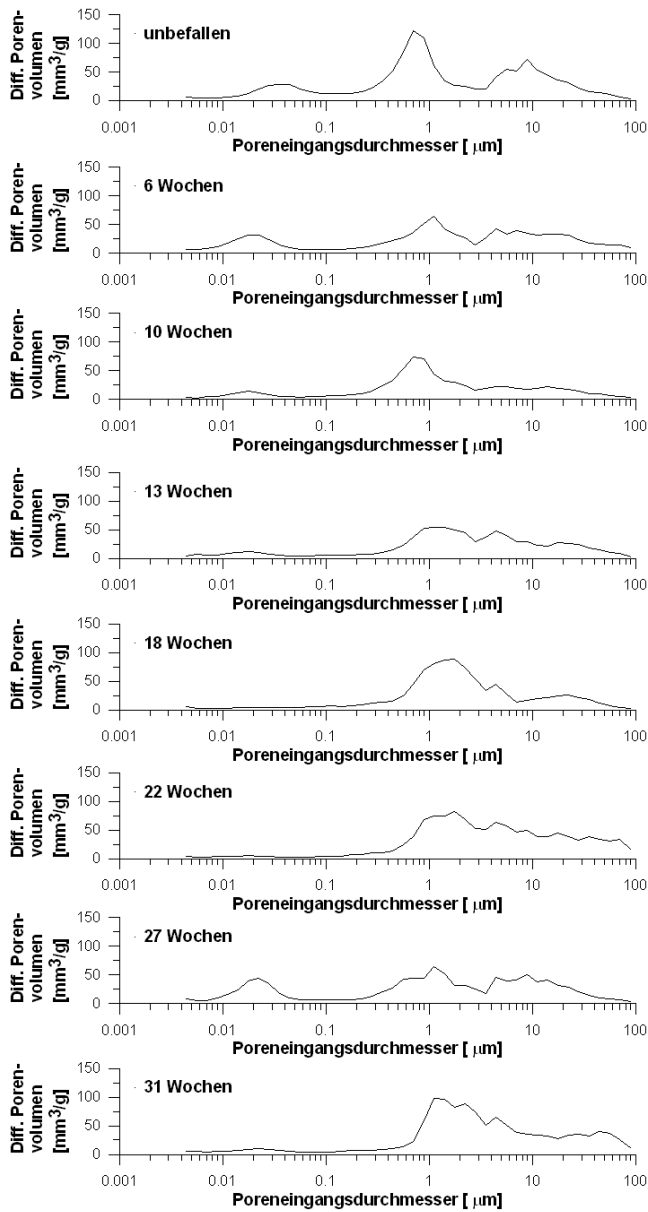
Abbildung B.6: Poreneingangsdurchmesser für alle in Kapitel 5.3.1 untersuchten axialen Eichenwirrlingsproben. Oben ist die unfallenen Probe zu sehen; darauf folgend die Proben mit zunehmender Inkubationszeit.
