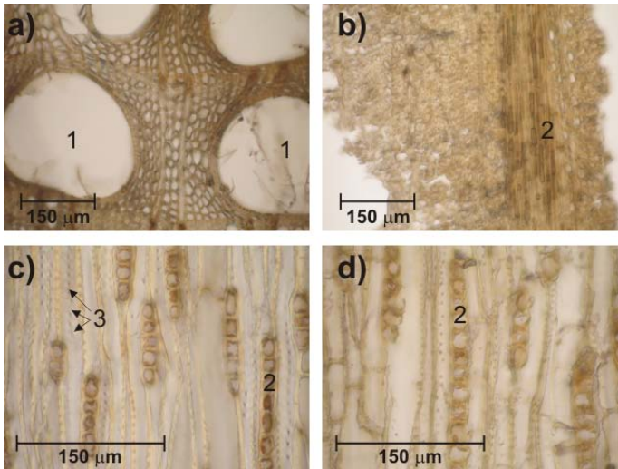
Abbildung 5.20: Mikroskopische Aufnahmen der befallenen und unbefallenen Proben. a) radialer Schnitt der axialen, unbefallenen Probe, 20-fache Vergrößerung. b) radialer Schnitt der axialen, befallenen Probe, 20-fache Vergrößerung. c) axialer Schnitt der radialen, unbefallenen Probe, 40-fache Vergrößerung. d) axialer Schnitt der radialen, befallenen Probe, 40-fache Vergrößerung. 1 - Lumen (große Poren), 2 - Holzstrahlen, 3 - Tüpfel (Porenverbindungen).
