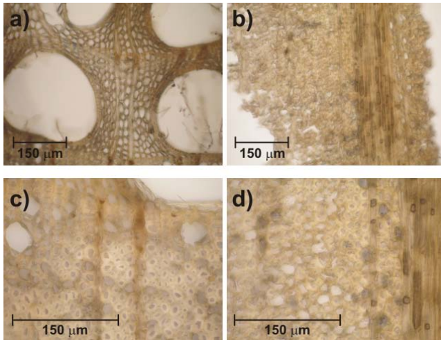
Abbildung B.12: Mikroskopische Aufnahmen der axialen Proben. Die Schnitte sind radial angesetzt. Bild a) unbeefallene Probe in 20 - facher Auflösung, Bild b) unbeefallene Probe in 40 - facher Auflösung, Bild c) befallene Probe in 20 - facher Auflösung, Bild d) befallene Probe in 40 - facher Auflösung.
