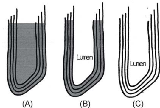
Abbildung 2.5: Drei Feuchtigkeitsgrenzzustände von Holzzellen. A: Lumen und Holzzellen sind wassergefüllt. Es herrscht Wassersättigung. Die Feuchtigkeit beträgt bis zu 200 %. B: Die Fasern sind wassergesättigt. In den Lumen ist kein Wasser. Es herrscht Fasersättigung. Der Feuchtegehalt beträgt 28 - 32 %. C: In den Lumen und Zellwänden ist kein Wasser. Das Holz ist darrtrocken. Die Feuchtigkeit beträgt 0%. (verändert nach Kempe (1999)).
